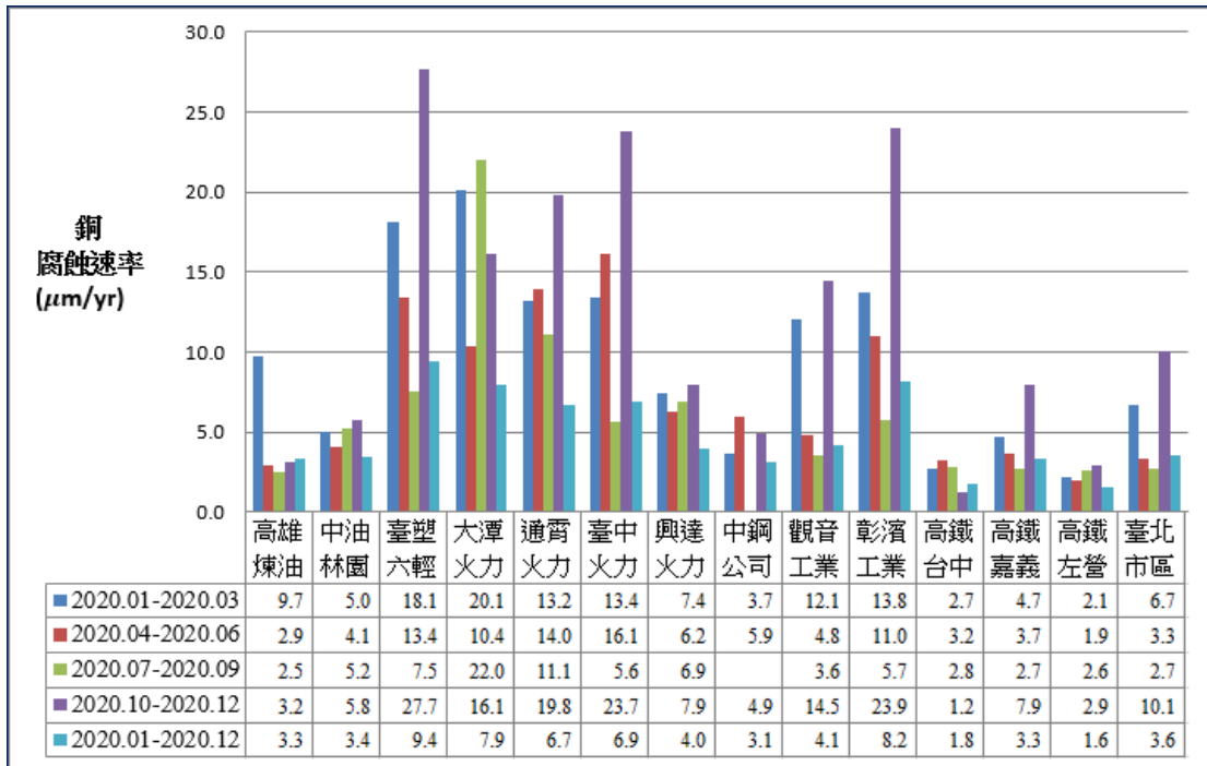
圖 6.7 特定測站銅腐蝕速率比較圖
