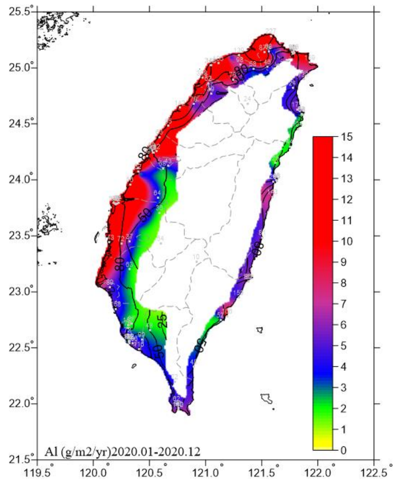
圖 6.28 2020 年一年期鋁腐蝕速率
