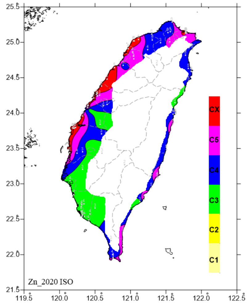
圖 6.30 2020 年鋅年腐蝕速率 ISO 分類圖
