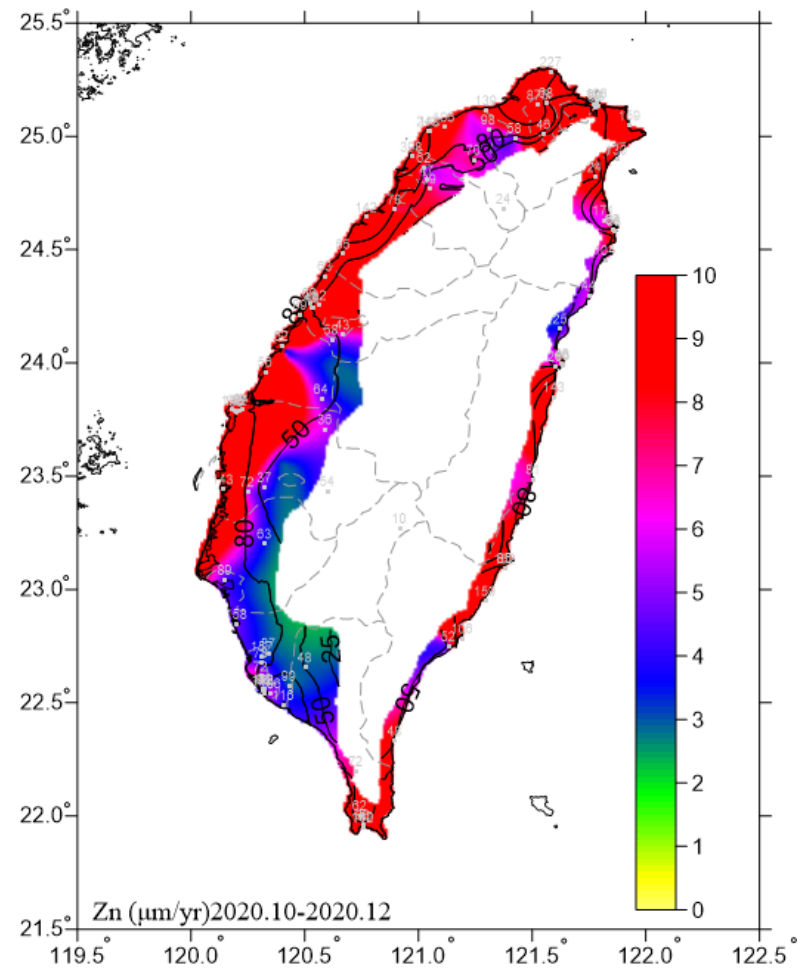
圖 6.16 2020.10-2020.12 鋅腐蝕速率圖
