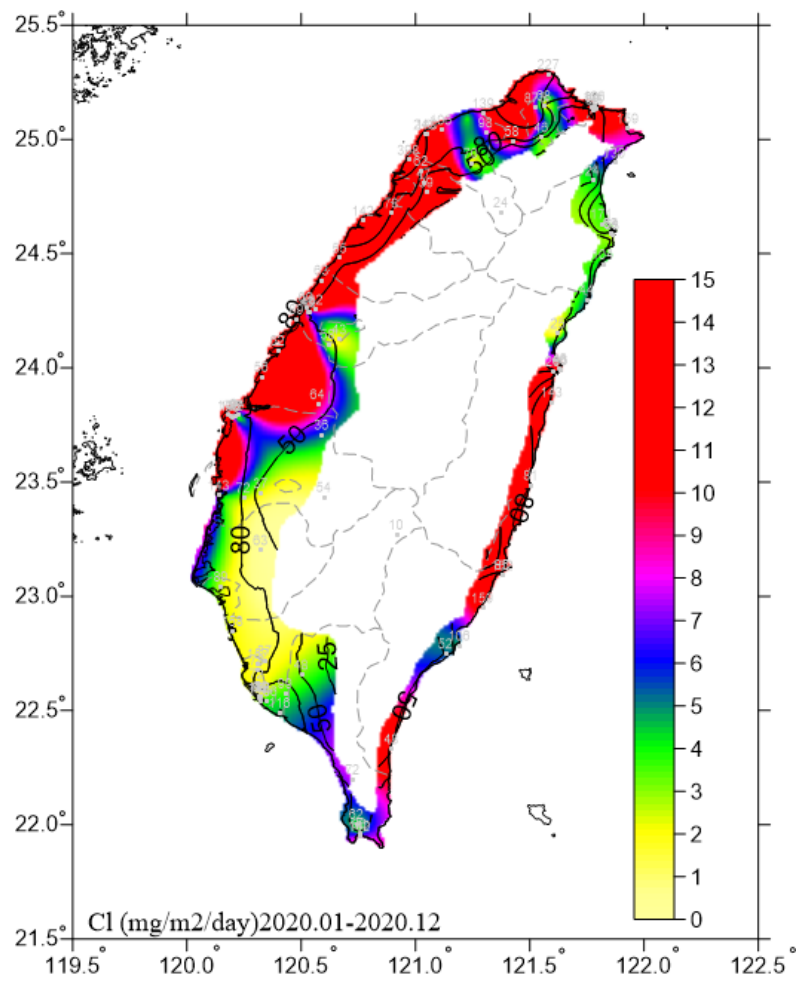
圖 4.5 2020 年一年期氣鹽沉積速率圖
