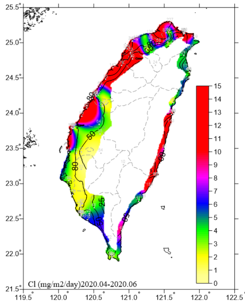
圖 4.2 2020.04-2020.06 氯鹽沉積速率圖
