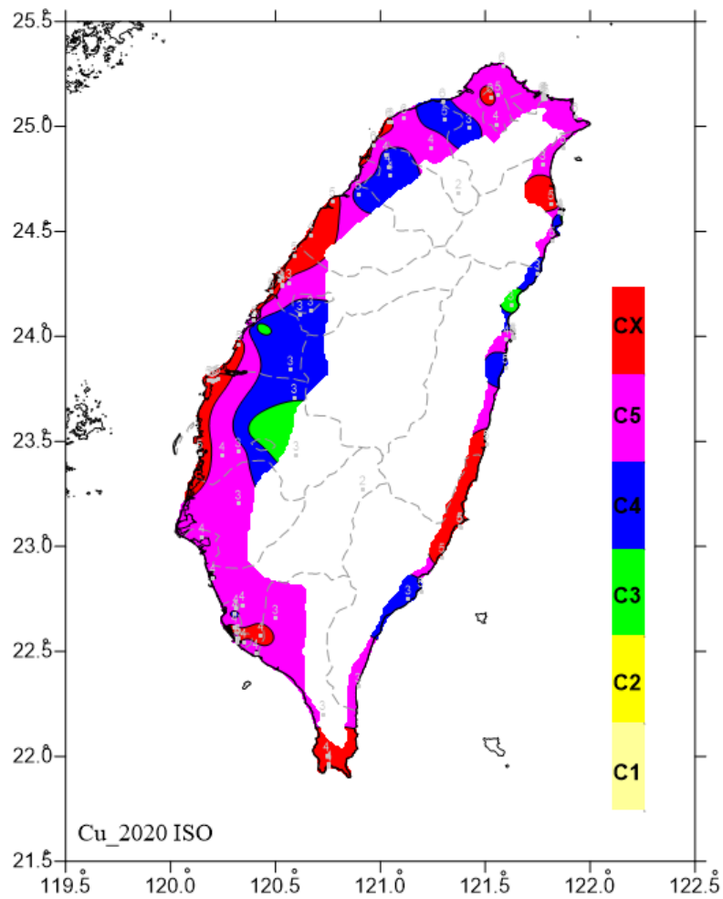
圖 6.31 2020 年銅年腐蝕速率 ISO 分類圖
