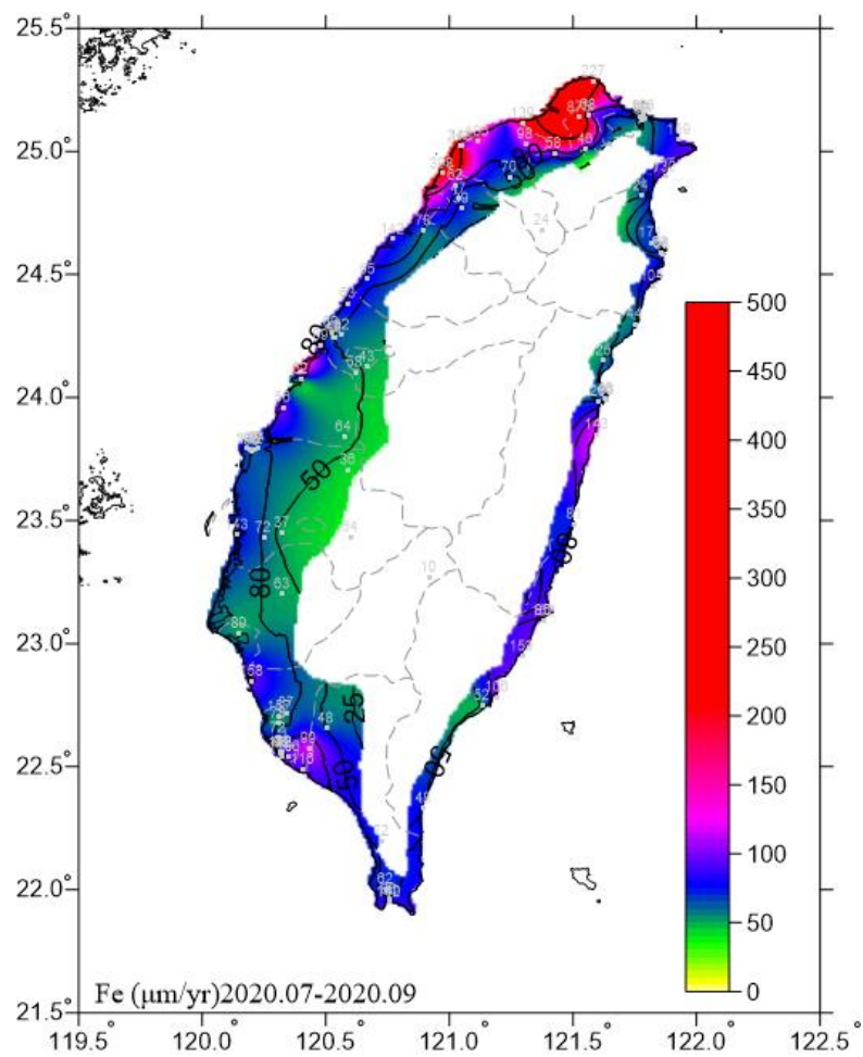
圖 6.11 2020.07-2020.09 碳鋼腐蝕速率圖
