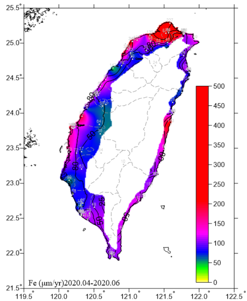
圖 6.10 2020.04-2020.06 碳鋼腐蝕速率圖
