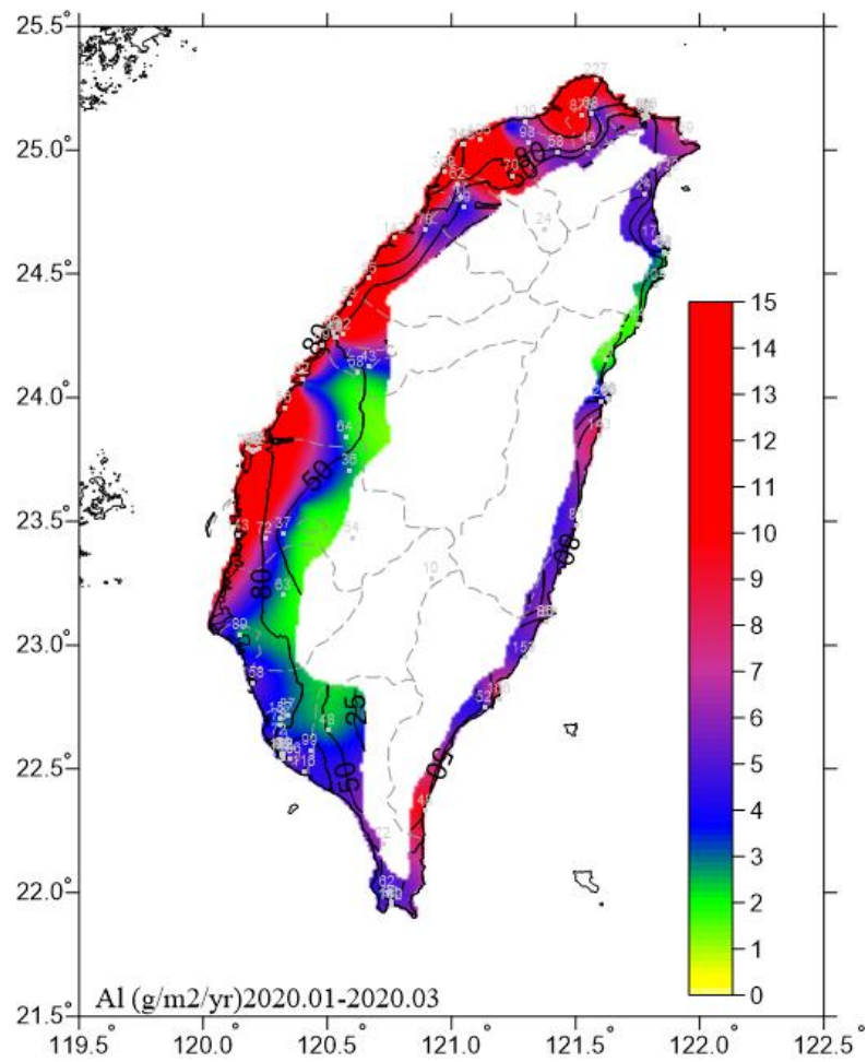
圖 6.21 2020.01-2020.03 鋁腐蝕速率圖
