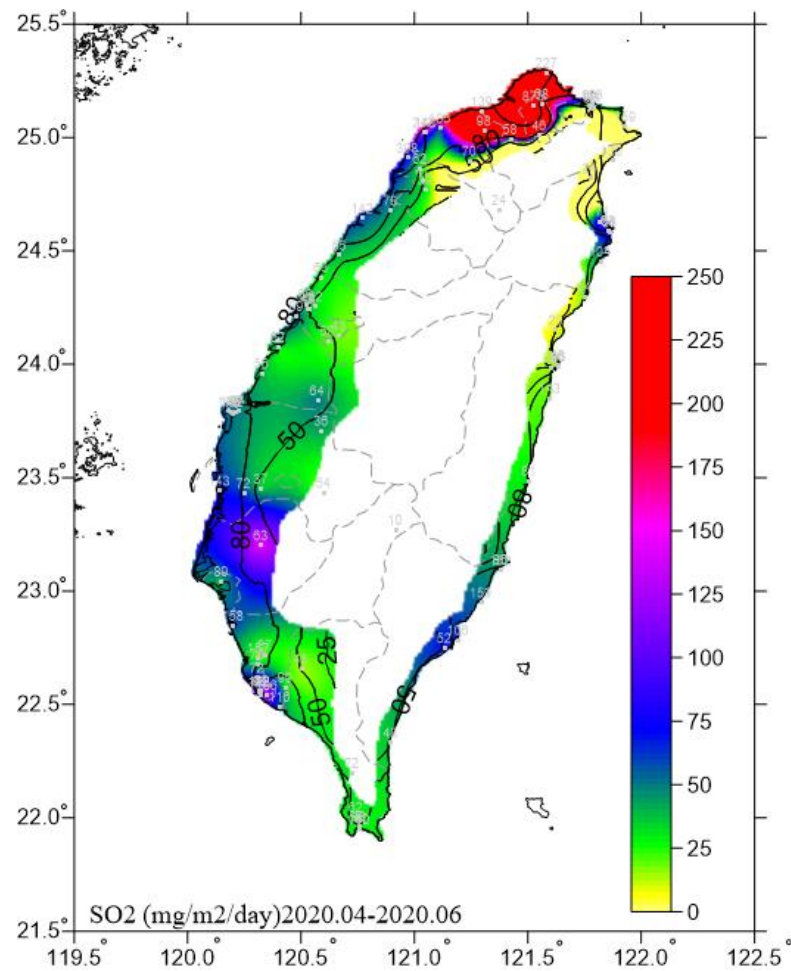
圖 5.2 2020.04-2020.06 二氧化硫沉積速率圖
