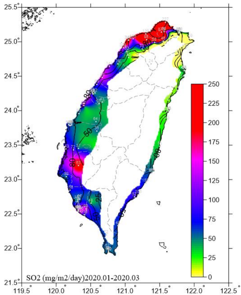
圖 5.1 2020.01-2020.03 二氧化硫沉積速率圖
