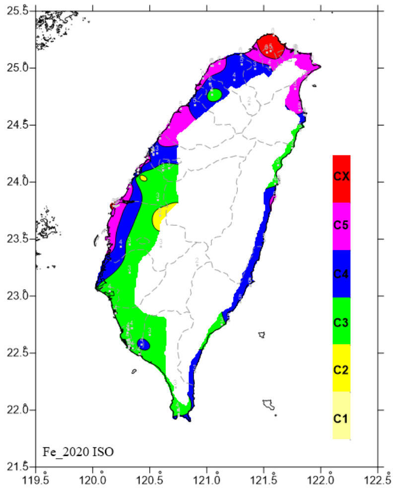
圖 6.29 2020 年碳鋼年腐蝕速率 ISO 分類圖
