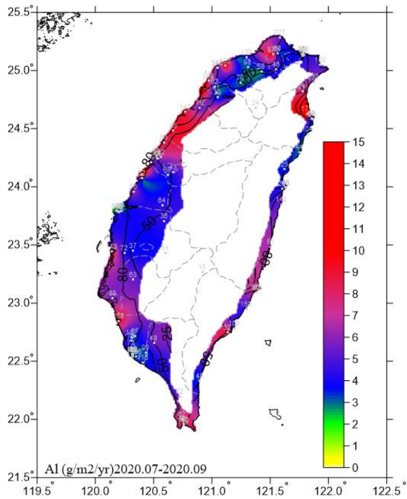
圖 6.23 2020.07-2020.09 鋁腐蝕速率圖
