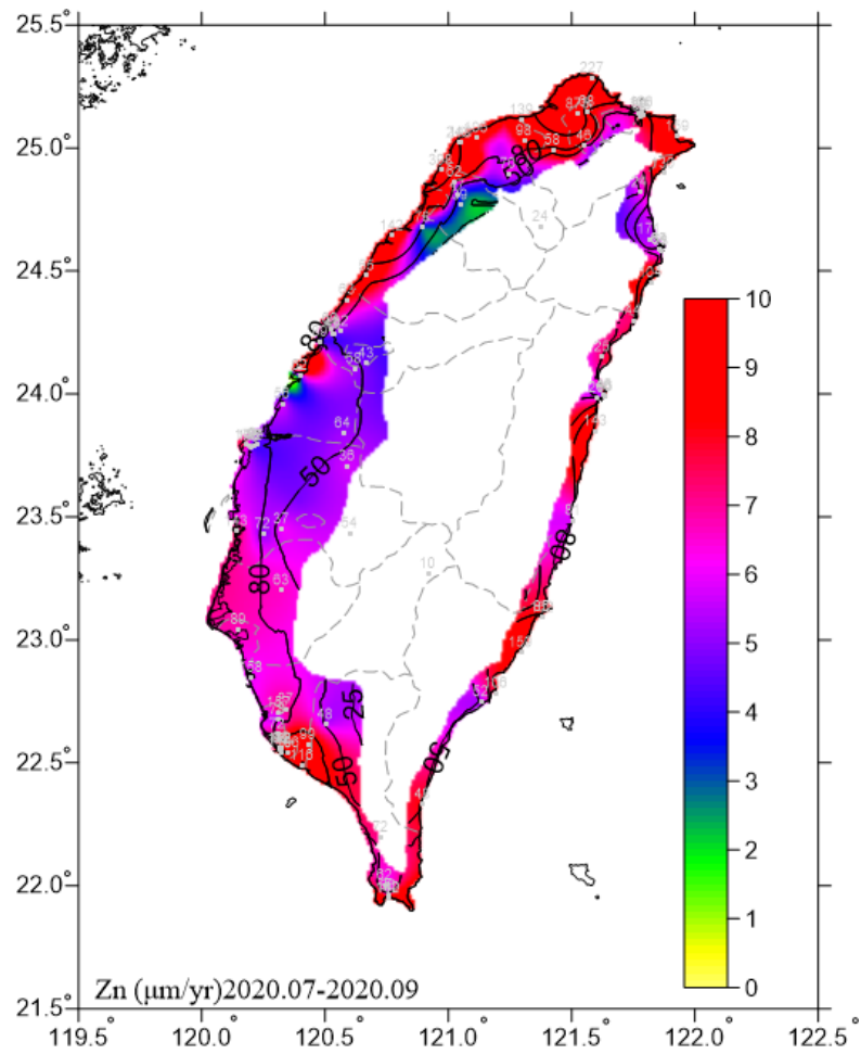
圖 6.15 2020.07-2020.09 鋅腐蝕速率圖
