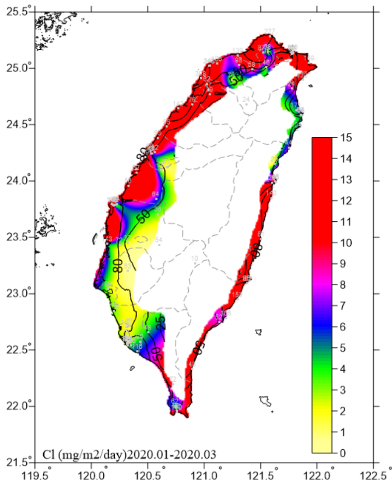
圖 4.1 2020.01-2020.03 氯鹽沉積速率圖
