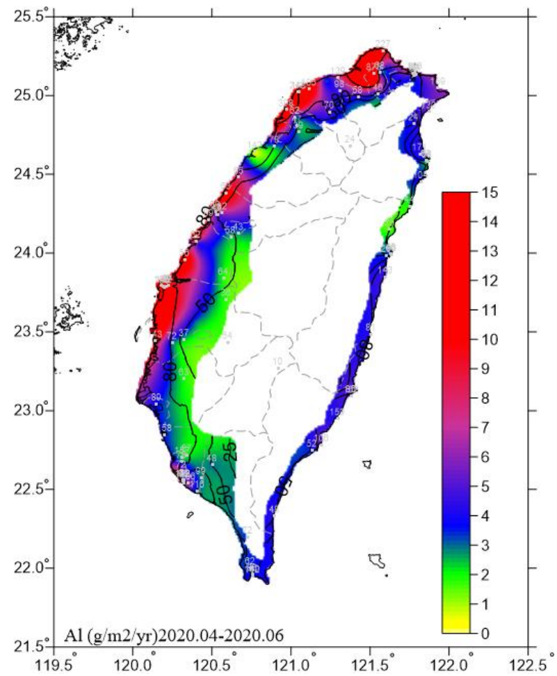
圖 6.22 2020.04-2020.06 鋁腐蝕速率圖
