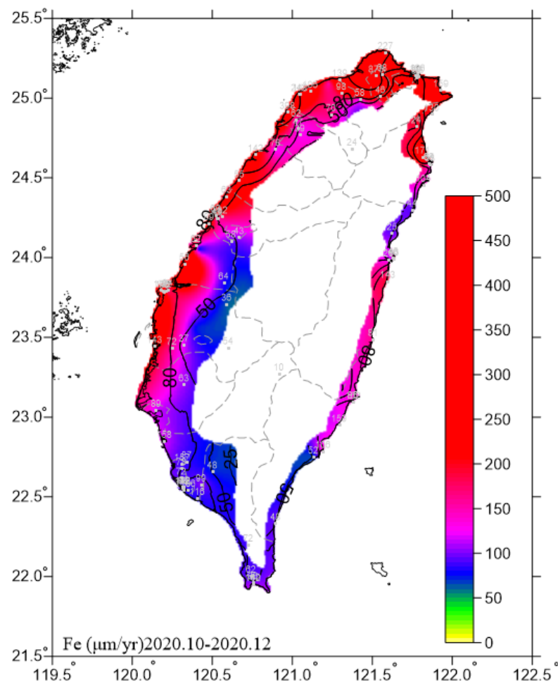
圖 6.12 2020.10-2020.12 碳鋼腐蝕速率圖
