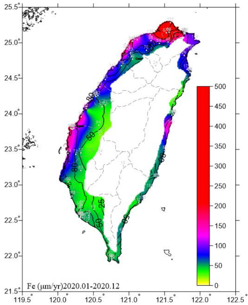
圖 6.25 2020 年一年期碳鋼腐蝕速率
