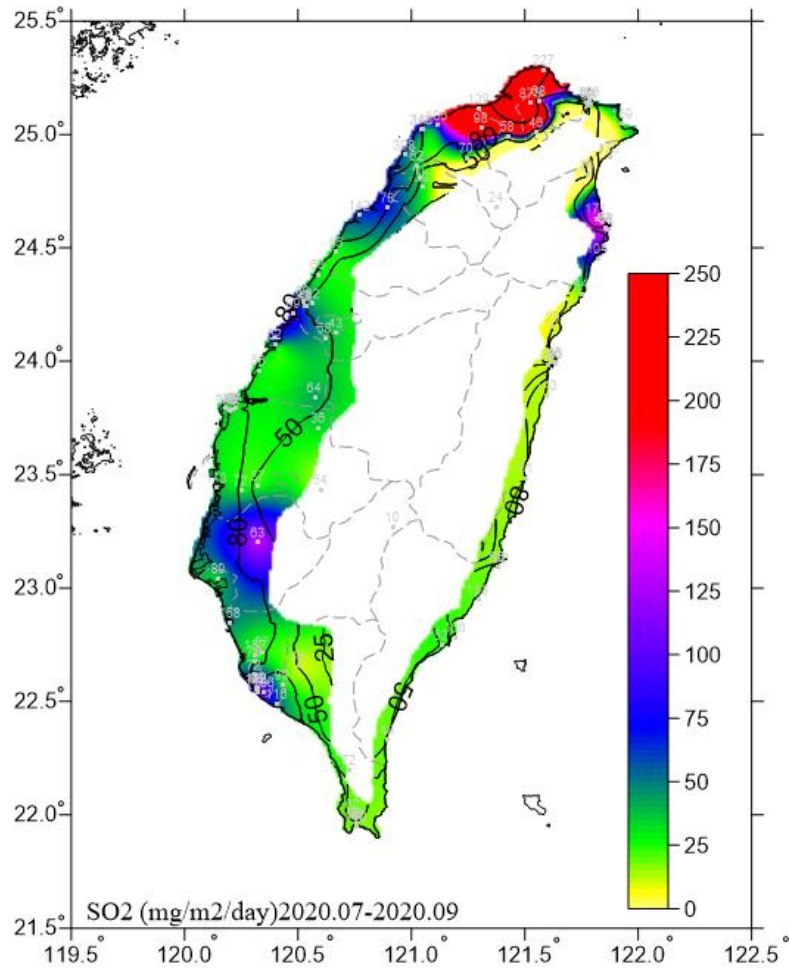
圖 5.3 2020.07-2020.09 二氧化硫沉積速率圖
