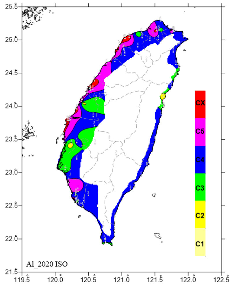
圖 6.32 2020 年鋁年腐蝕速率 ISO 分類圖
