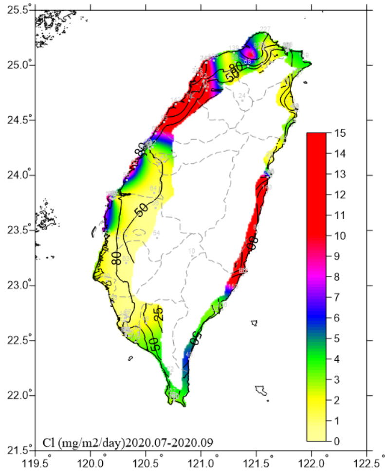
圖 4.3 2020.07-2020.09 氯鹽沉積速率圖
