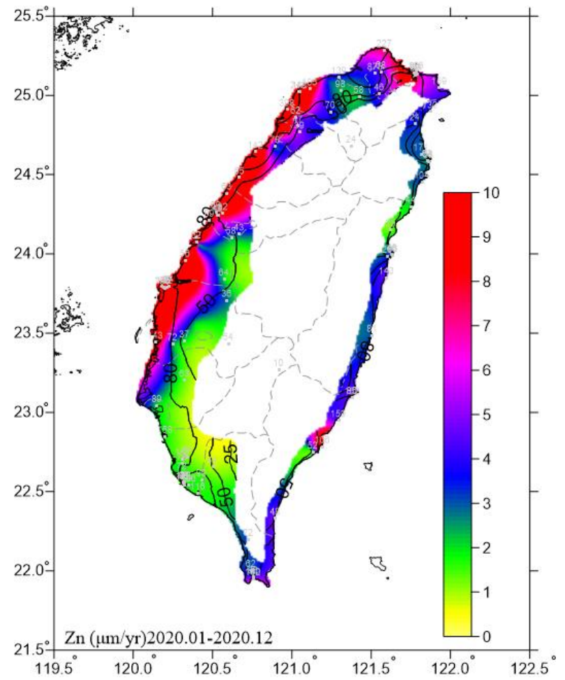
圖 6.26 2020 年一年期鋅腐蝕速率
