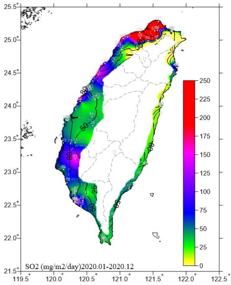
圖 5.5 2020 年二氧化硫沉積速率圖
