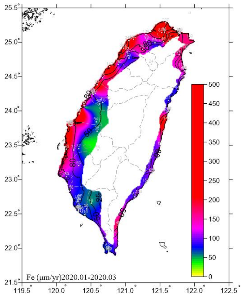
圖 6.9 2020.01-2020.03 碳鋼腐蝕速率圖
