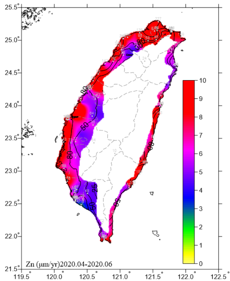
圖 6.14 2020.04-2020.06 鋅腐蝕速率圖
