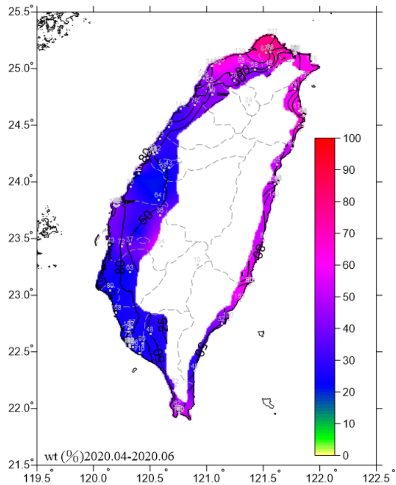
圖 3.2 2020.04-2020.06 濕潤時間圖
