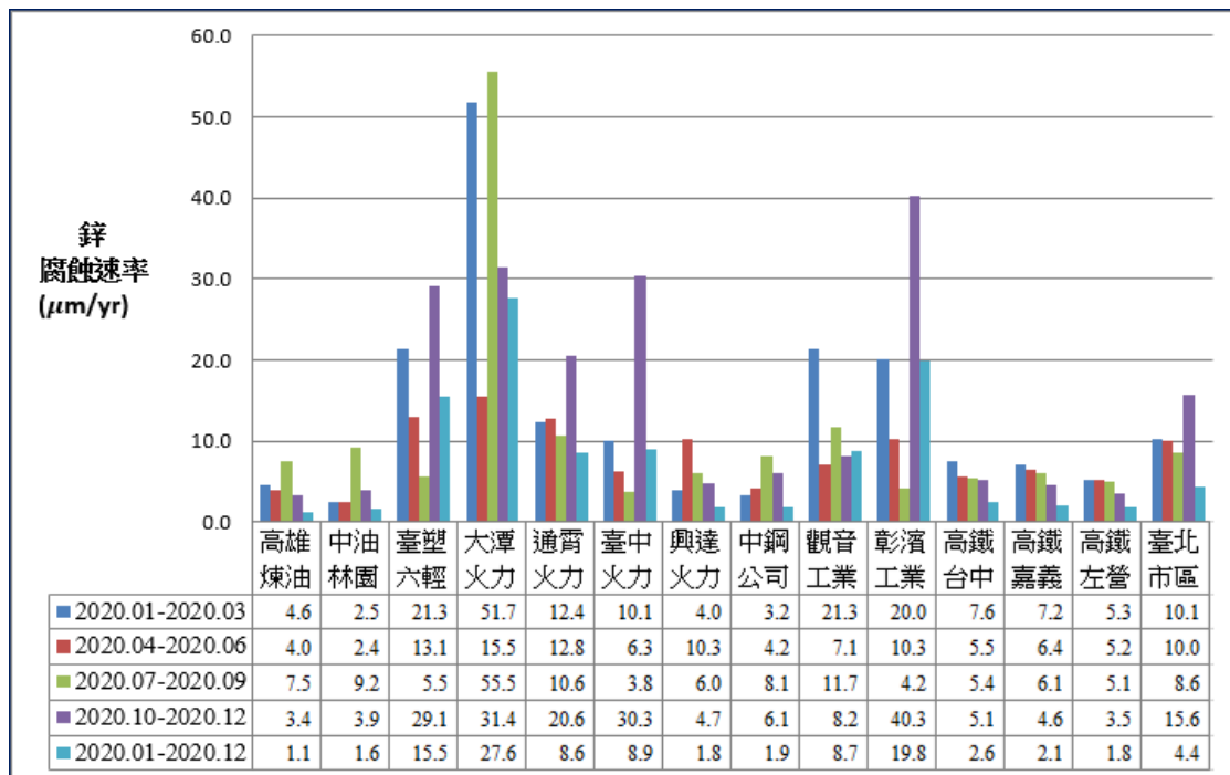
圖 6.5 特定測站碳鋼腐蝕速率比較圖
