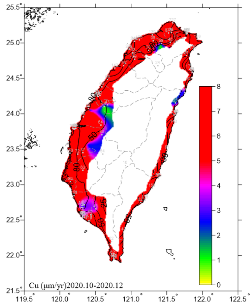
圖 6.20 2020.10-2020.12 銅腐蝕速率圖
