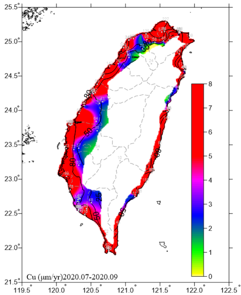
圖 6.19 2020.07-2020.09 銅腐蝕速率圖
