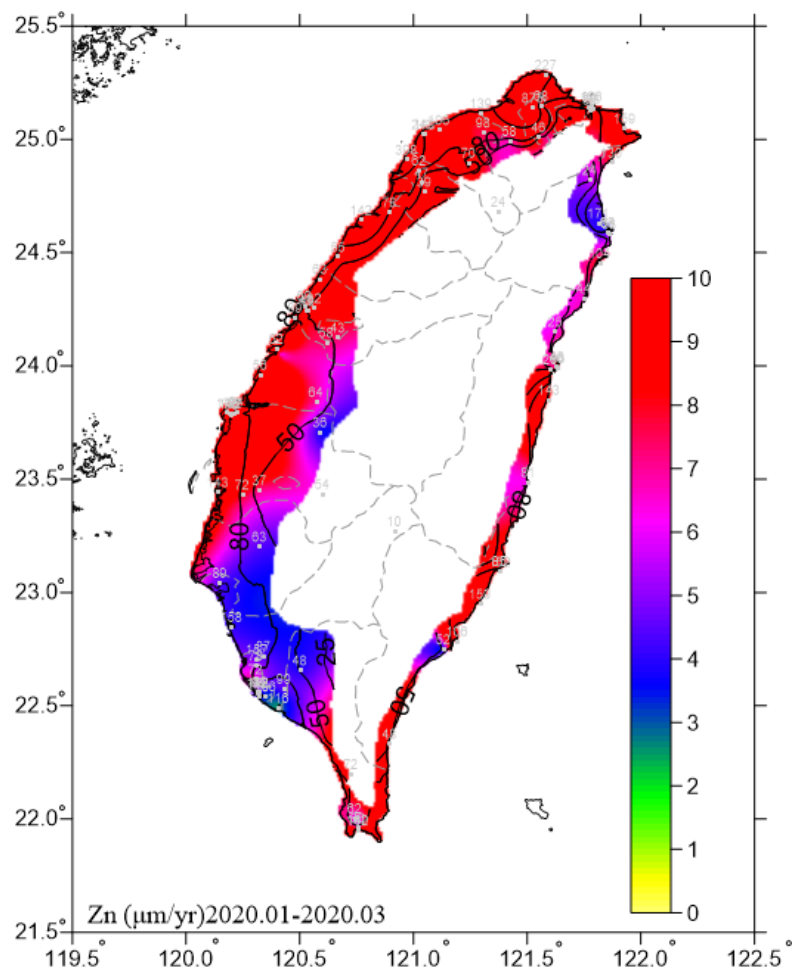
圖 6.13 2020.01-2020.03 鋅腐蝕速率圖
