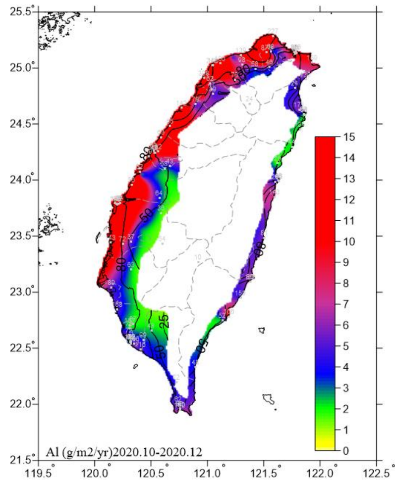
圖 6.24 2020.10-2020.12 鋁腐蝕速率圖
