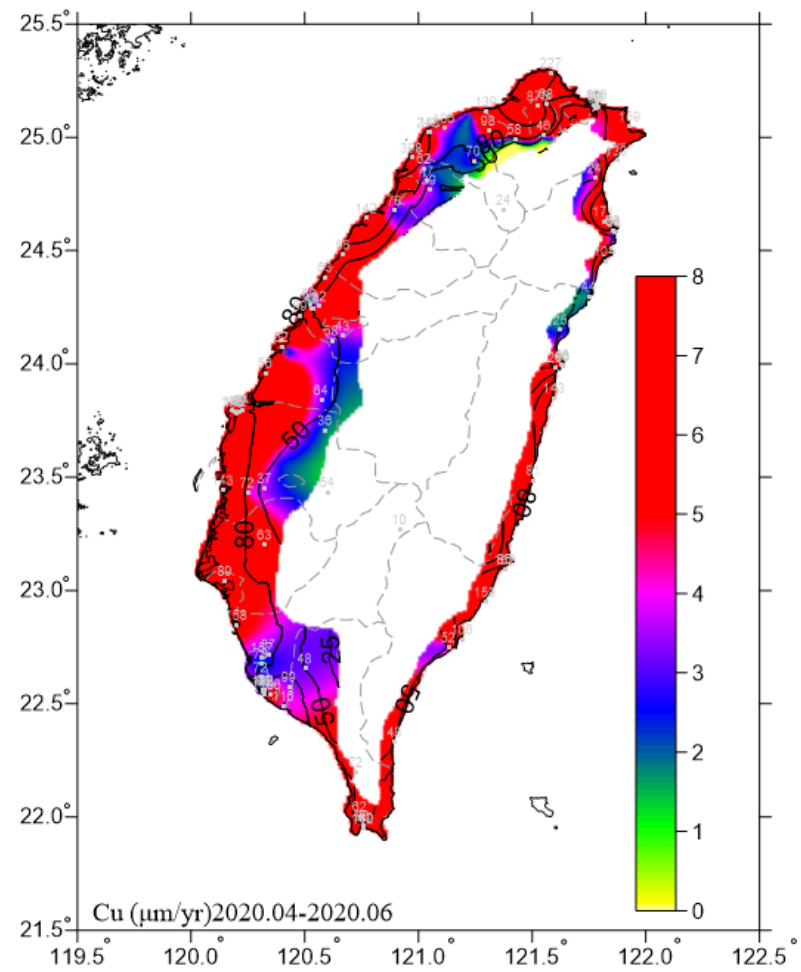
圖 6.18 2020.04-2020.06 銅腐蝕速率圖
