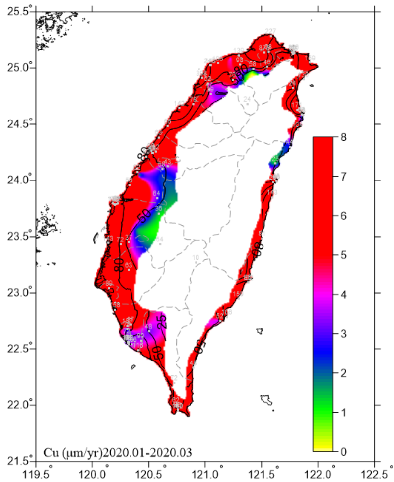
圖 6.17 2020.01-2020.03 銅腐蝕速率圖
