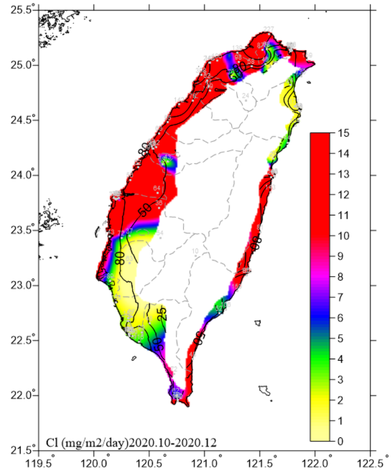
圖 4.4 2020.10-2020.12 氯鹽沉積速率圖
