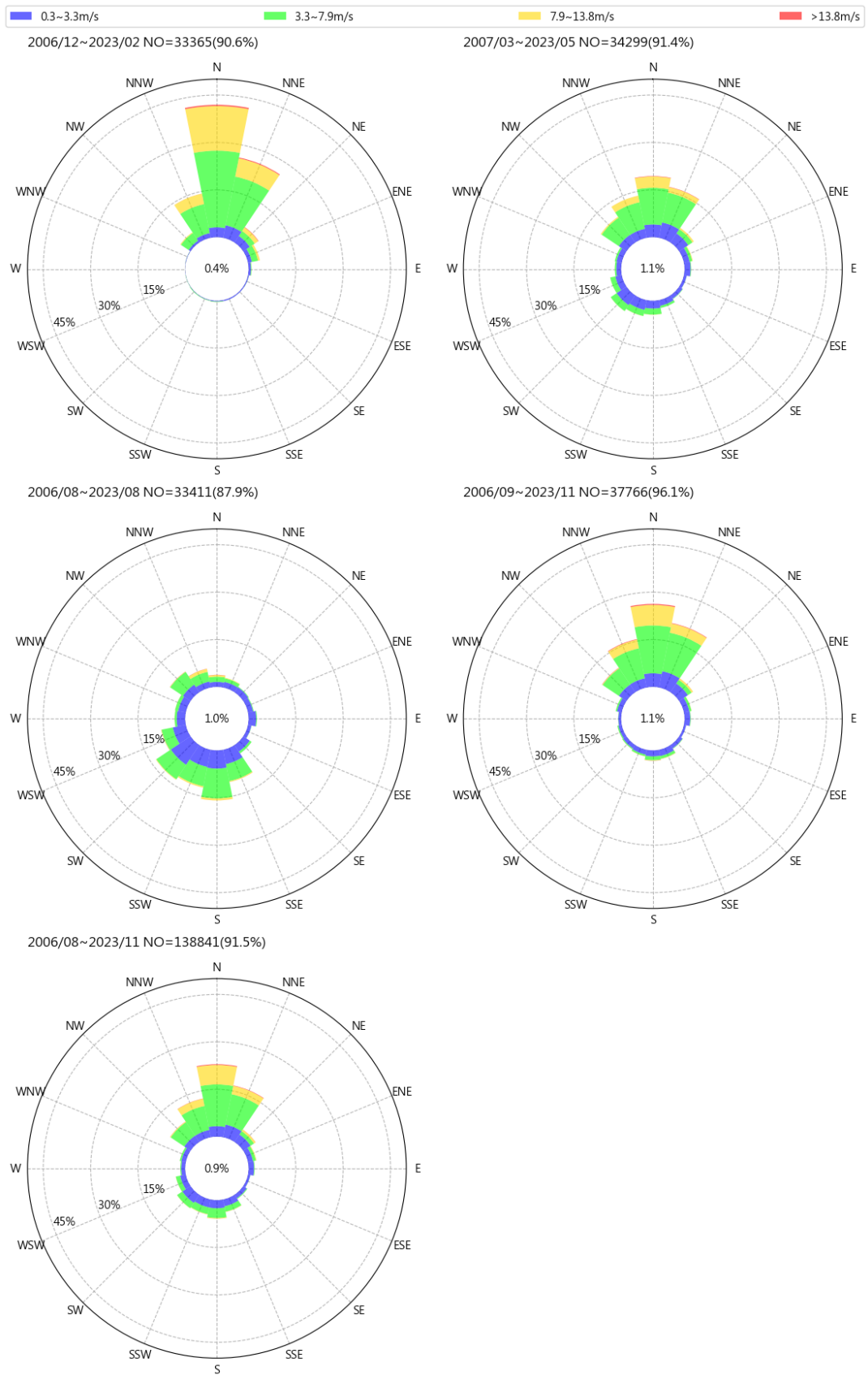
圖 8.8 歷年布袋港每季風速風向玫瑰圖
