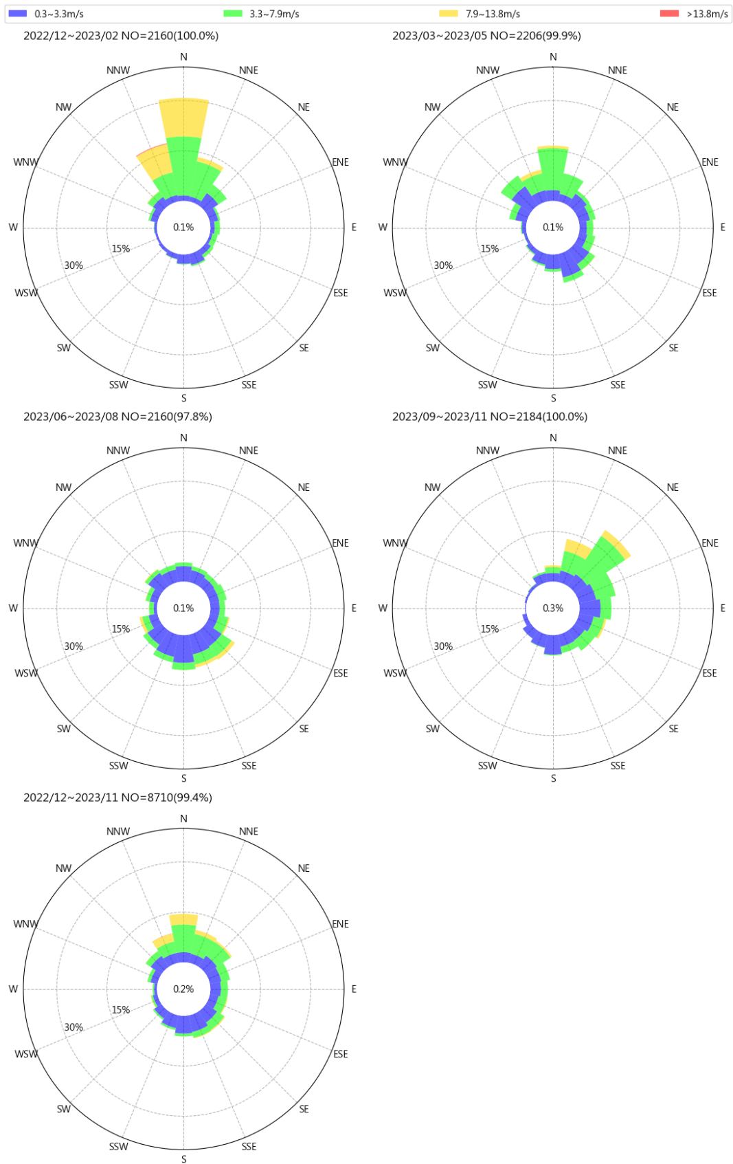
圖 3.6 2023 年基隆港每季風速風向玫瑰圖
