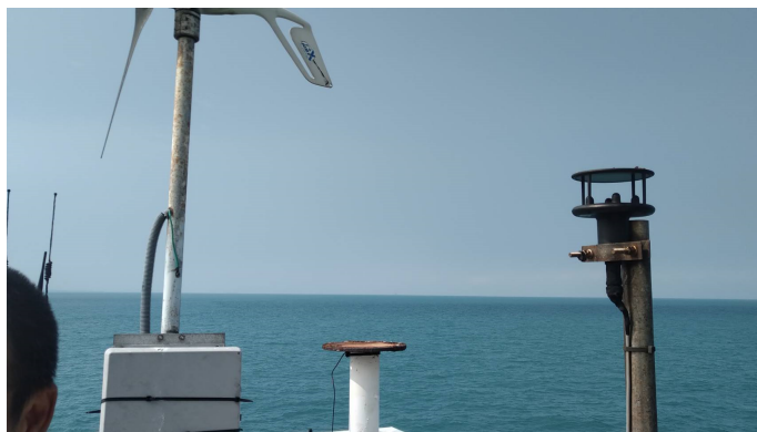
圖 2.2 臺北港風力觀測站現地照片
