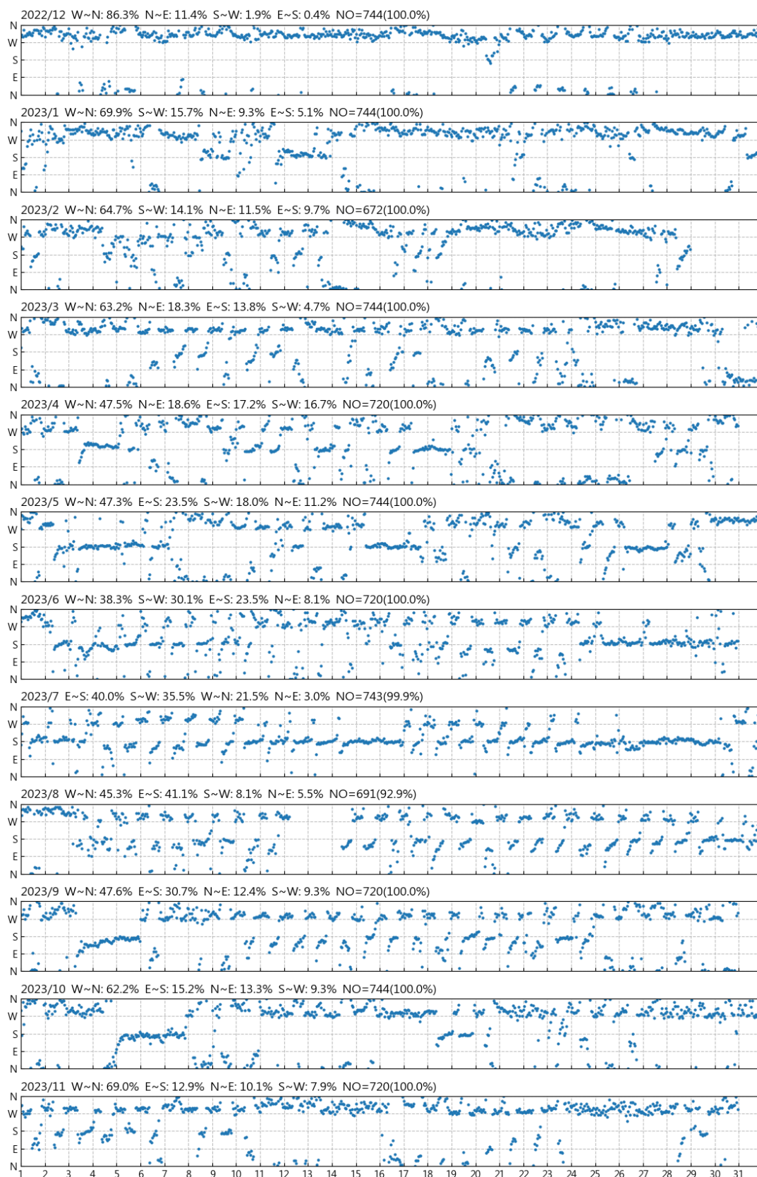
圖 4.4 2023 年蘇澳港每月風向歷線圖
