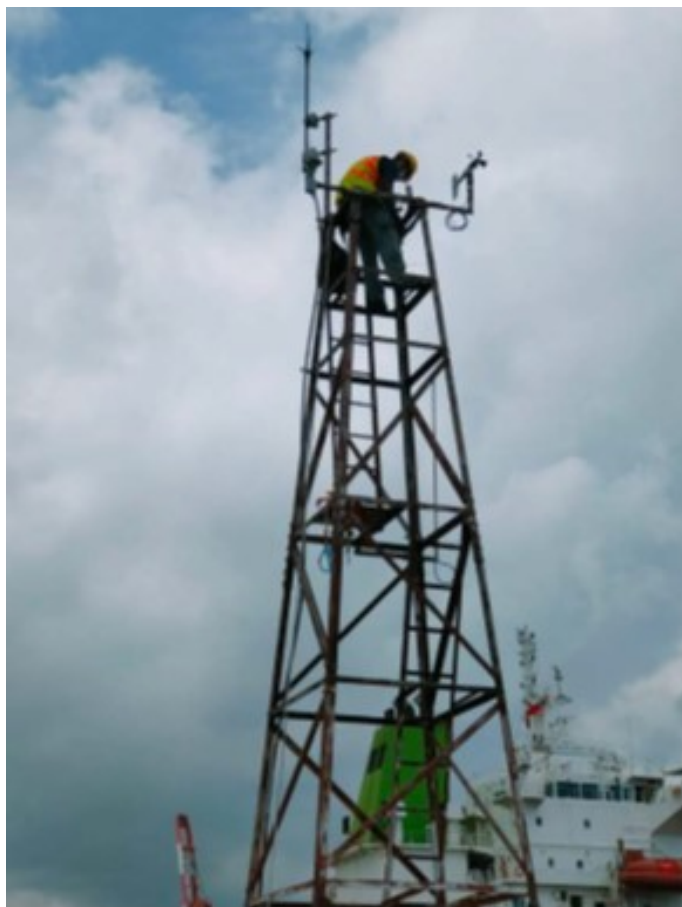
圖 3.2 基隆港風力觀測站現地照片
