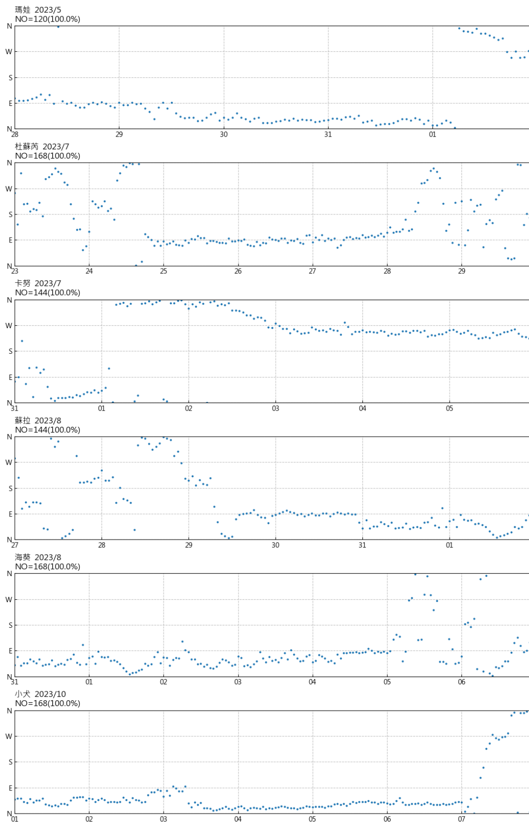
圖 2.10 2023 年臺北港颱風期間風向歷線圖
