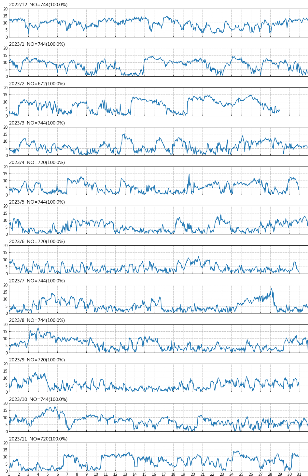
圖 2.3 2023 年臺北港每月風速歷線圖
