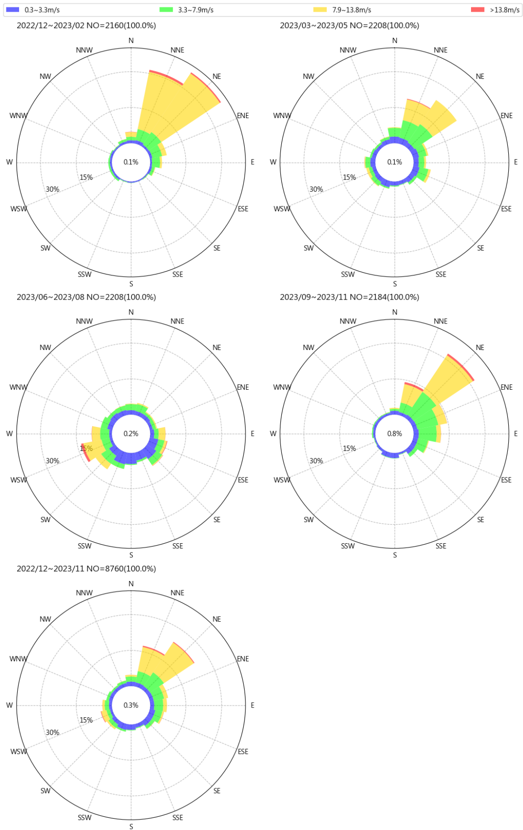
圖 2.6 2023 年臺北港每季風速風向玫瑰圖
