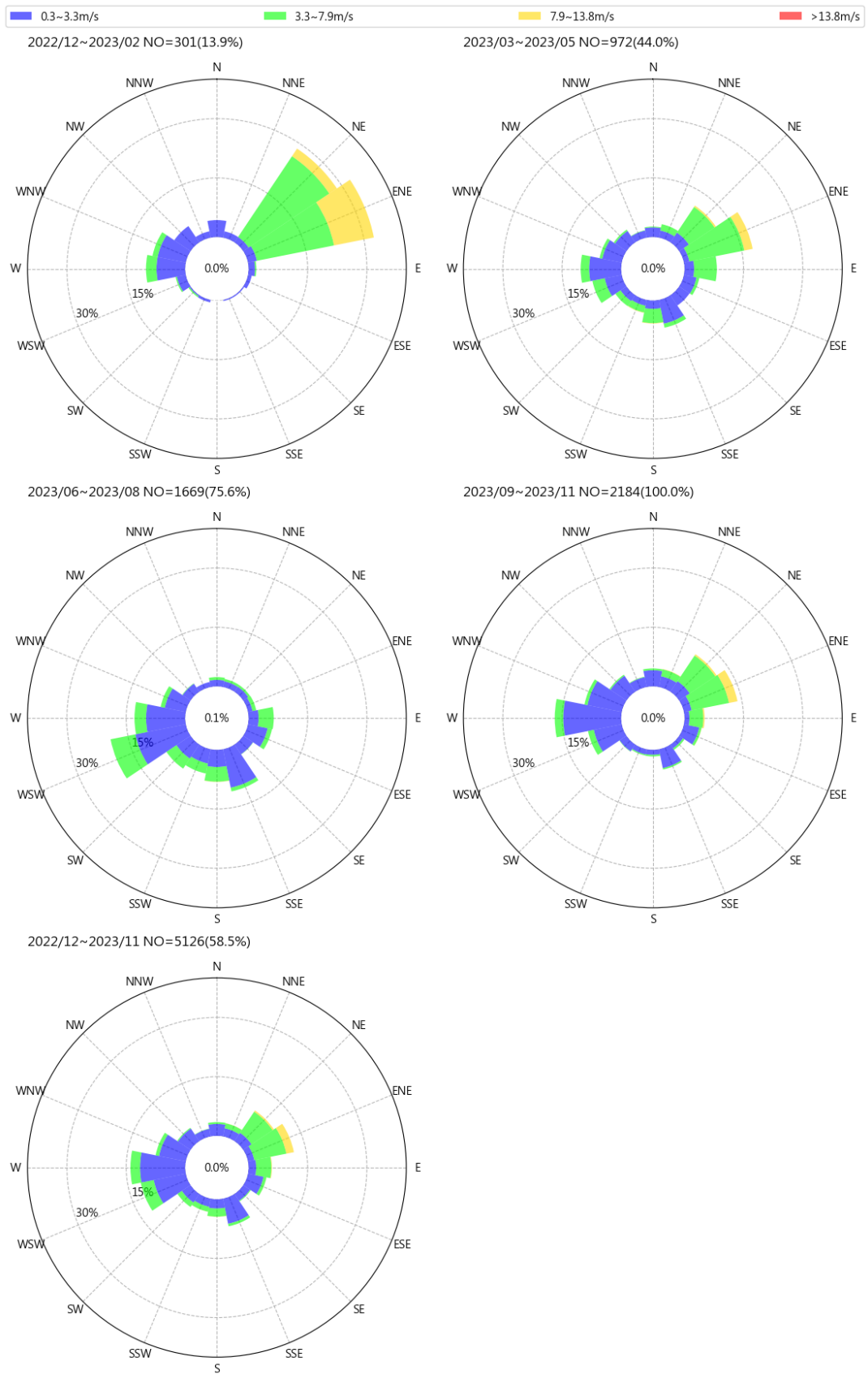
圖 5.6 2023 年花蓮港每季風速風向玫瑰圖
