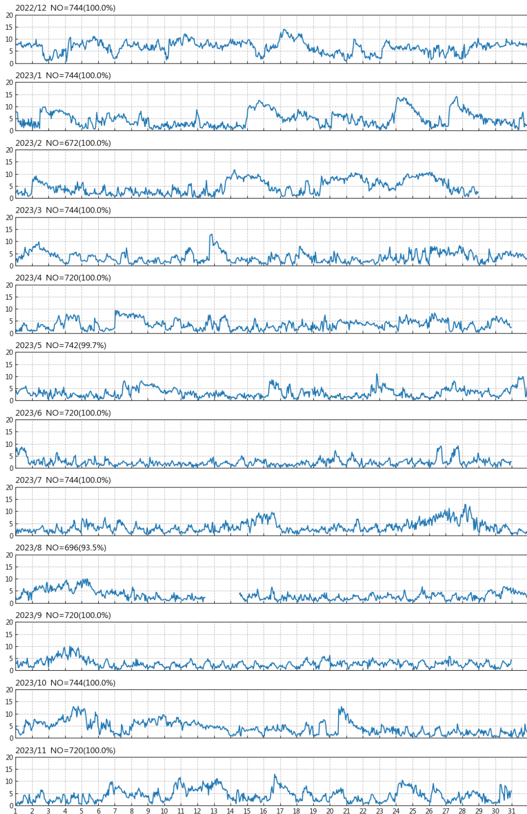
圖 3.3 2023 年基隆港每月風速歷線圖
