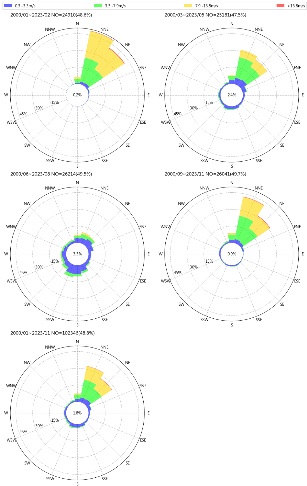
圖 10.8 歷年澎湖馬公港每季風速風向玫瑰圖
