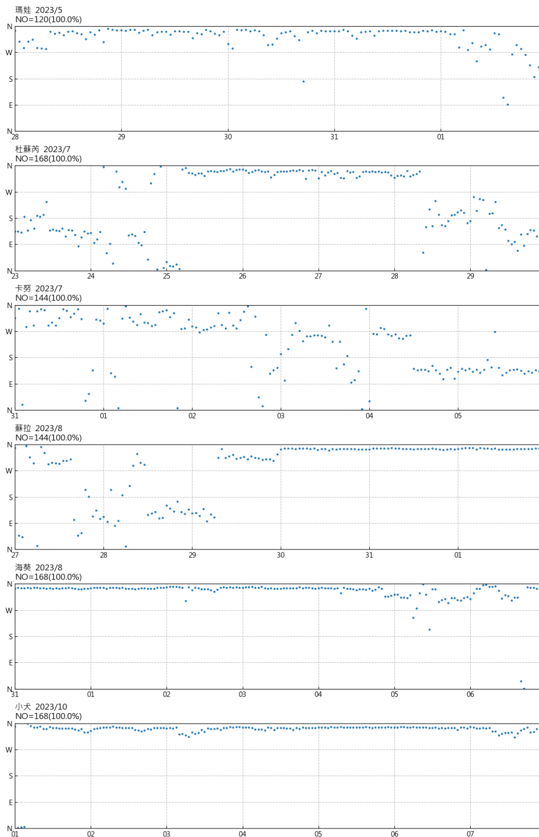
圖 11.10 2023 年馬祖南竿福澳港颱風期間風向歷線圖
