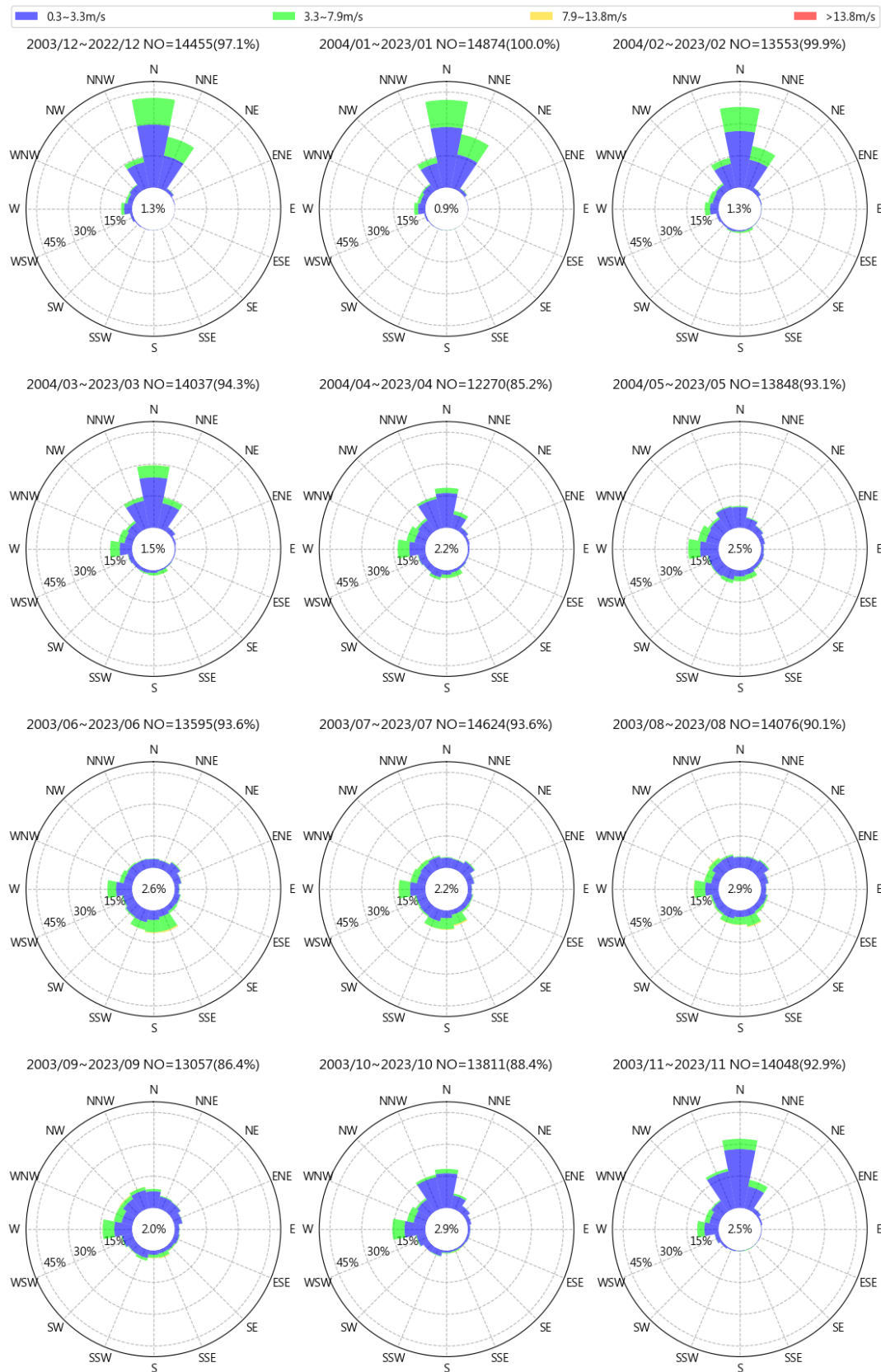
圖 6.7 歷年高雄港每月風速風向玫瑰圖
