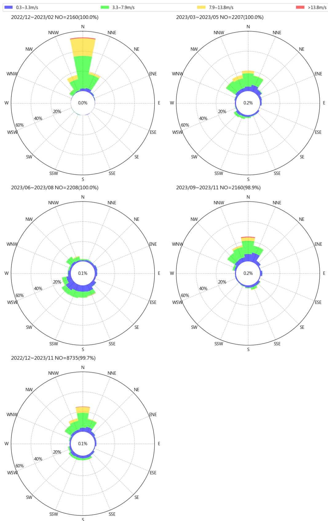
圖 8.6 2023 年布袋港每季風速風向玫瑰圖
