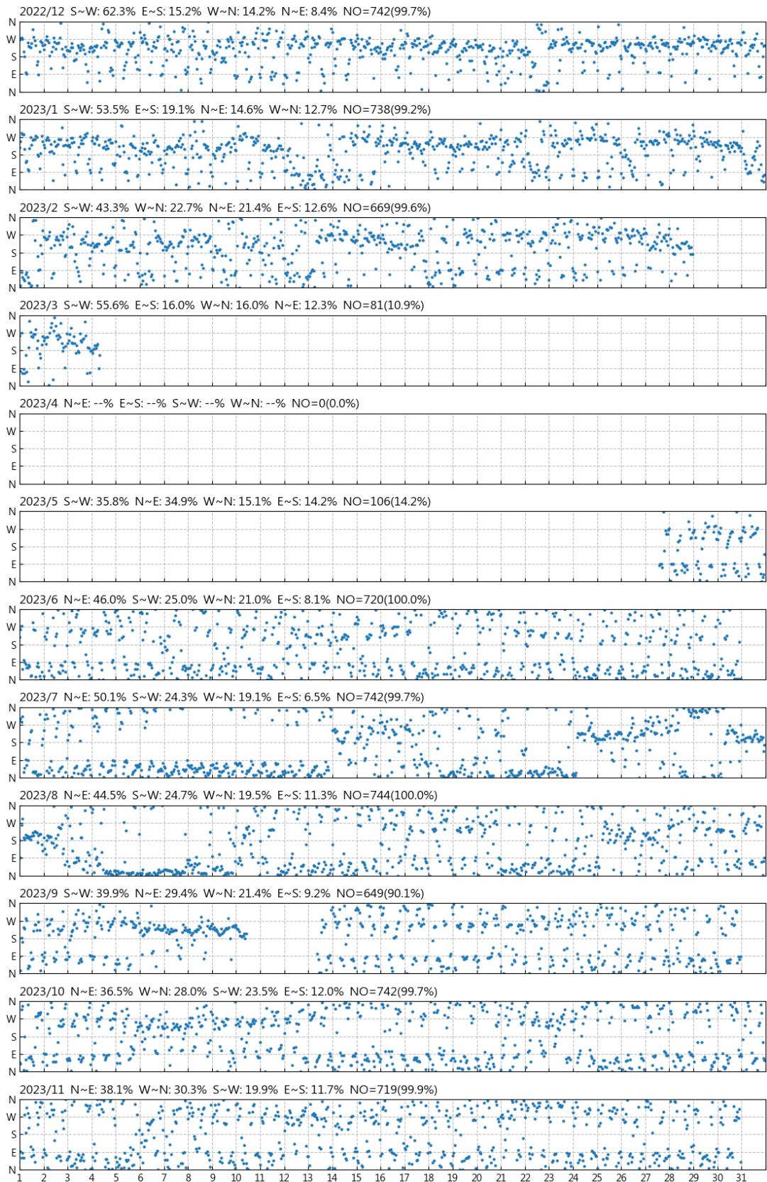
圖 12.4 2023 年馬祖南竿福澳港每月流向歷線圖
