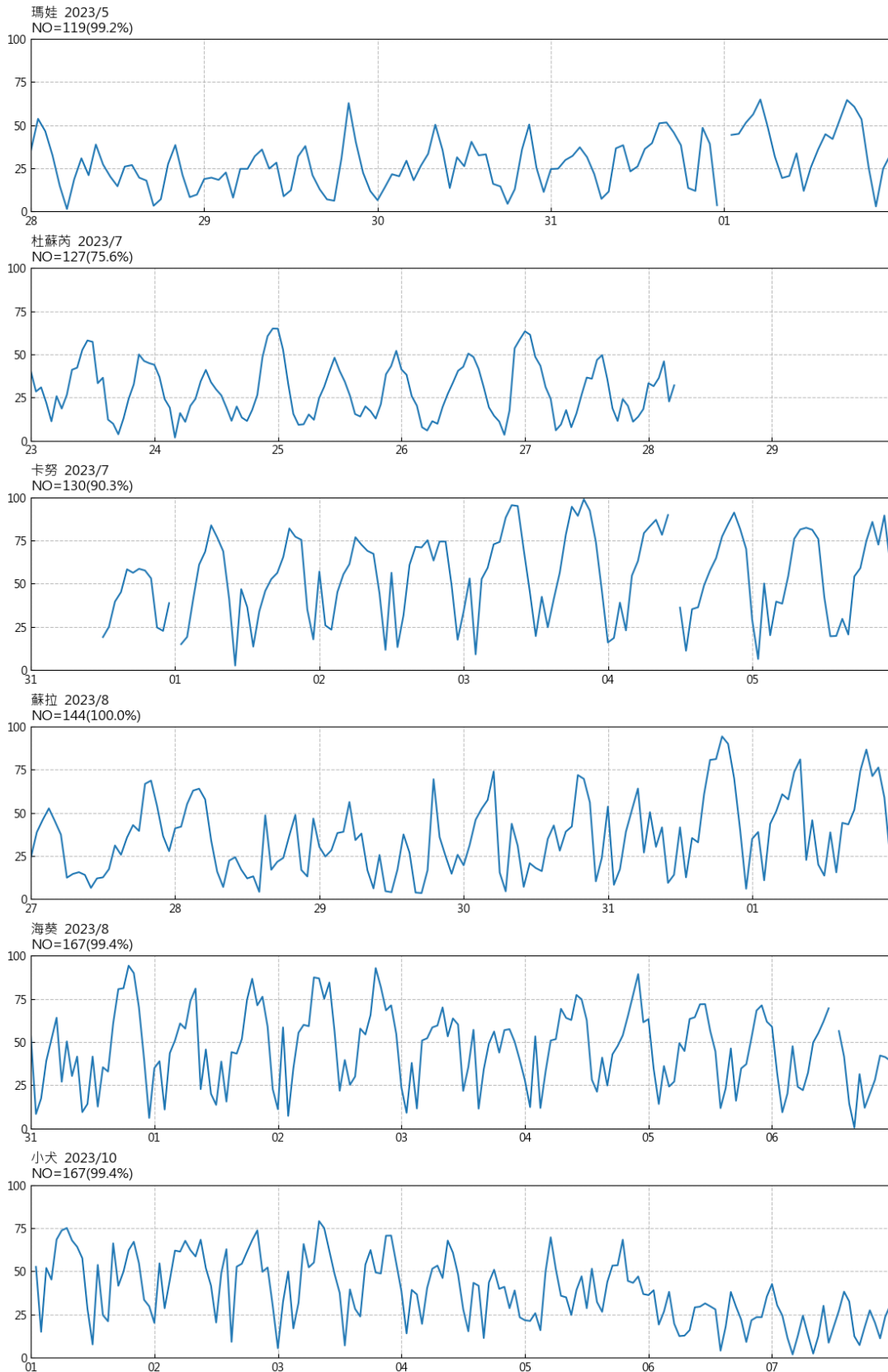
圖 10.9 2023 年澎湖龍門尖山港颱風期間流速歷線圖
