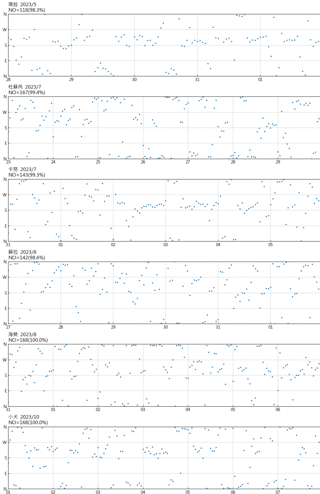
圖 4.10 2023 年蘇澳港颱風期間流向歷線圖
