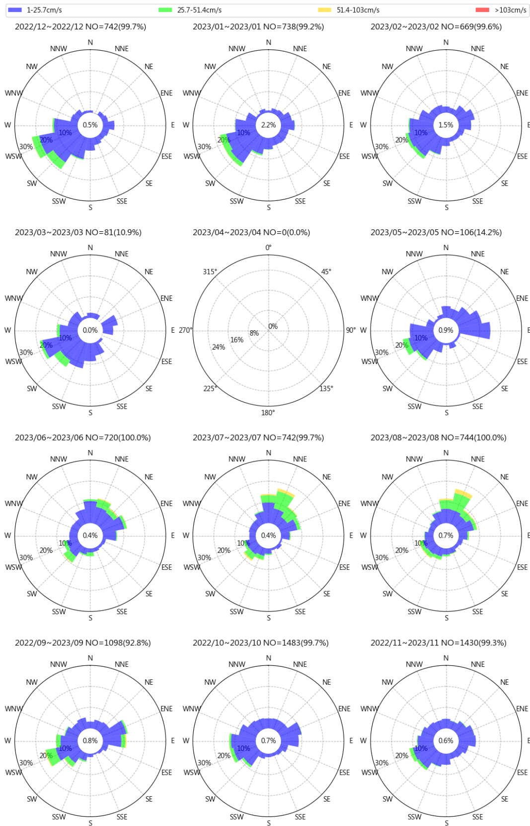
圖 12.7 歷年馬祖南竿福澳港每月流速流向玫瑰圖
