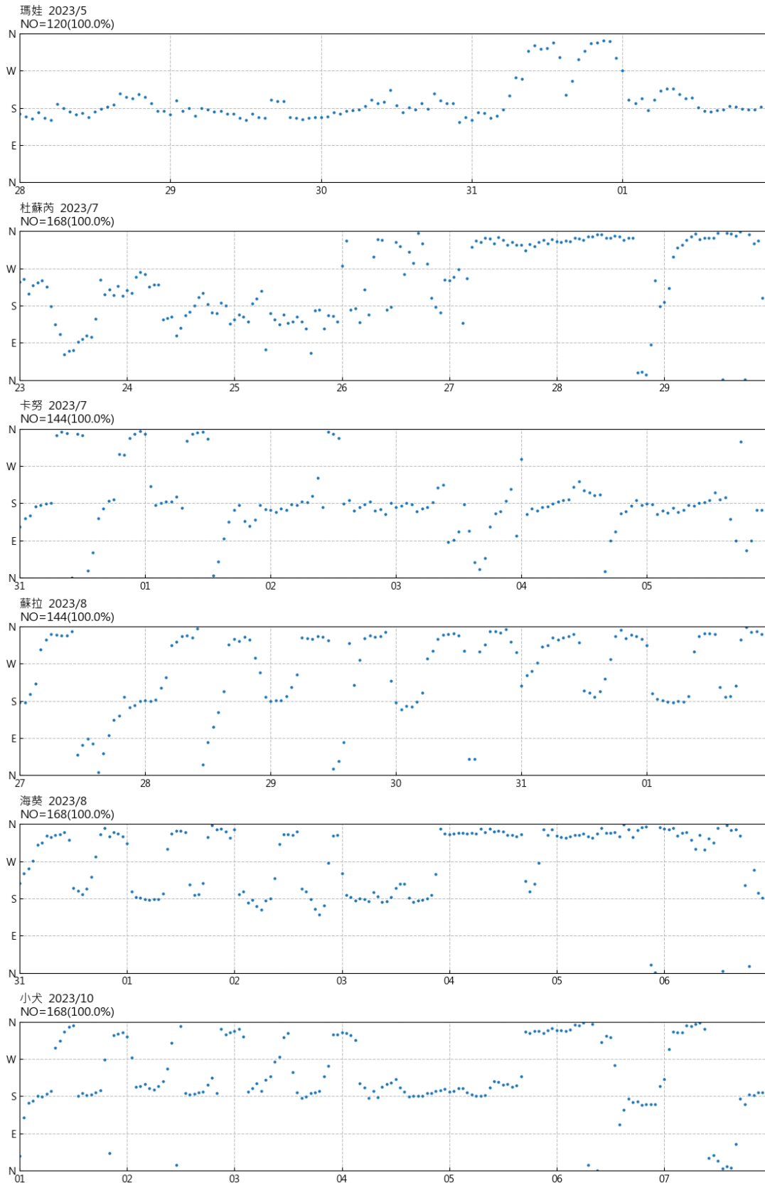
圖 6.10 2023 年高雄港颱風期間流向歷線圖
