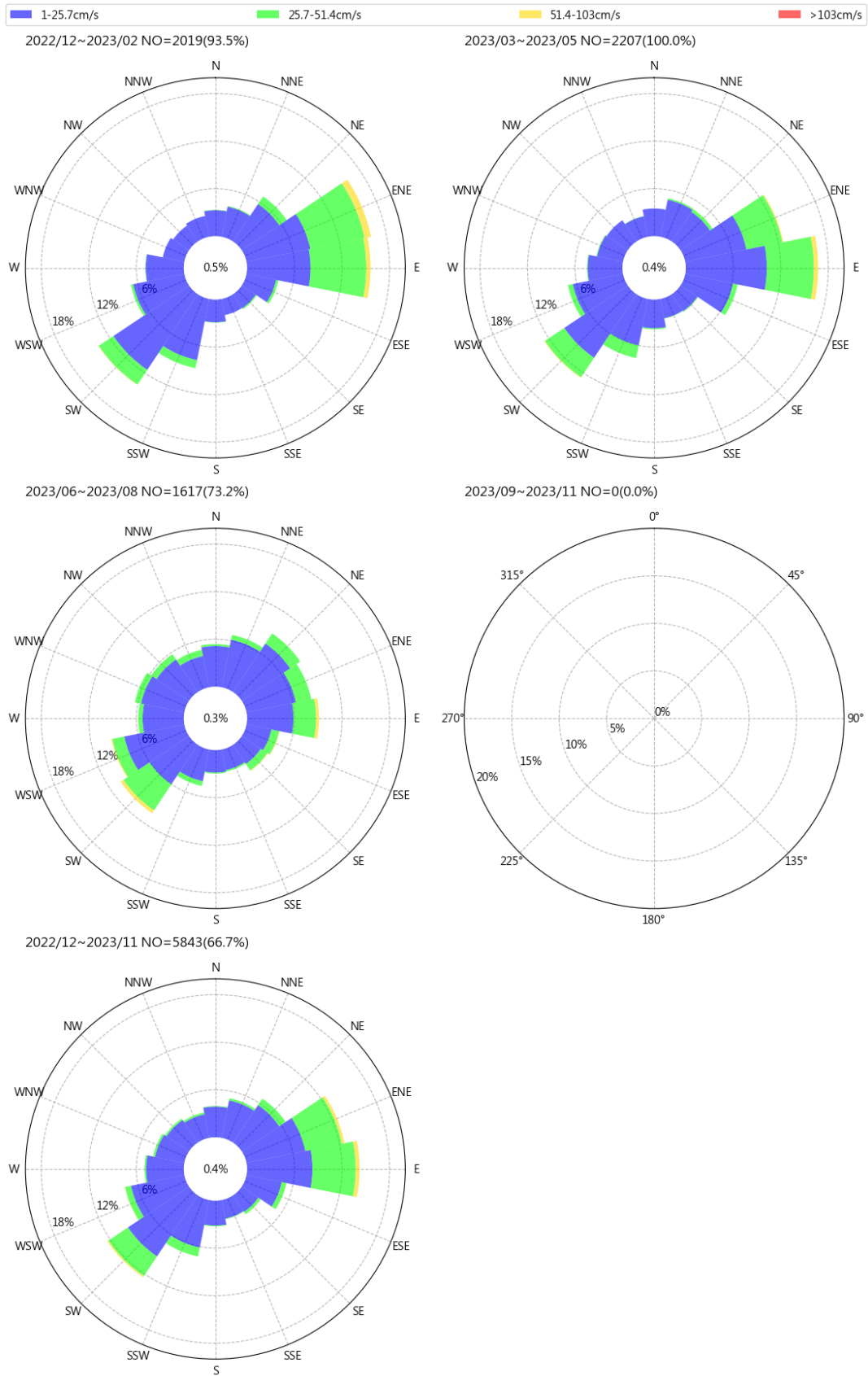
圖 3.6 2023 年基隆港每季流速流向玫瑰圖
