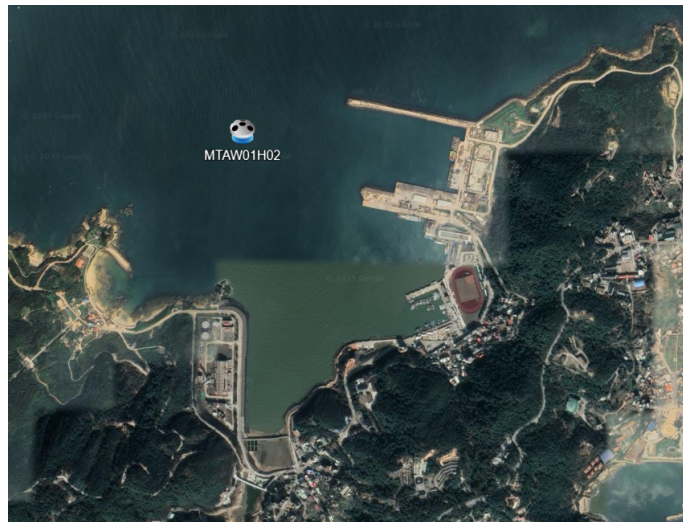
圖 12.1 馬祖南竿福澳港海流觀測站位置示意圖
