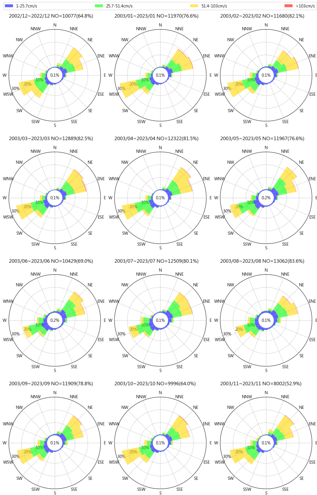
圖 2.7 歷年臺北港每月流速流向玫瑰圖
