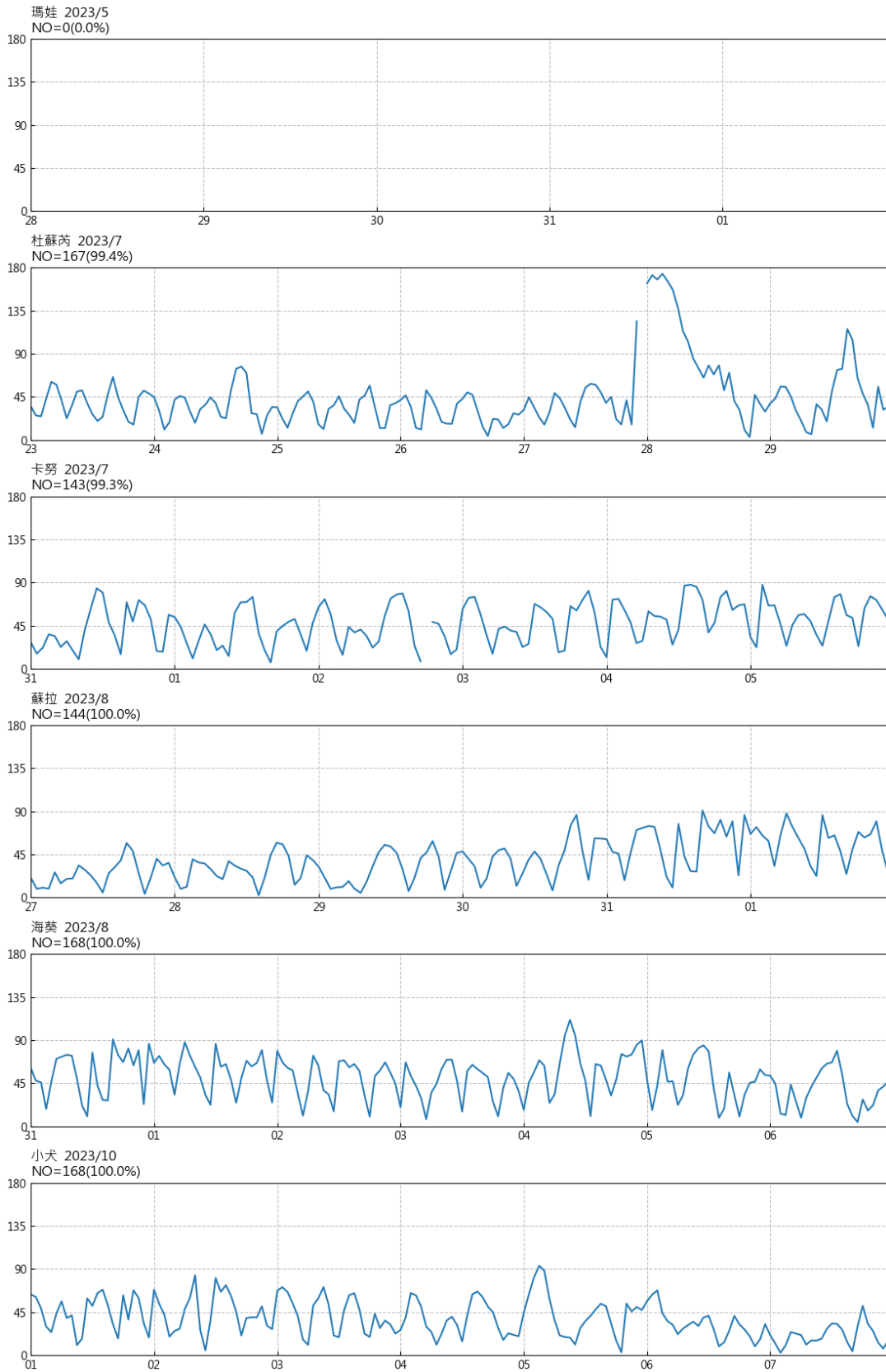
圖 7.9 2023 年安平港颱風期間流速歷線圖
