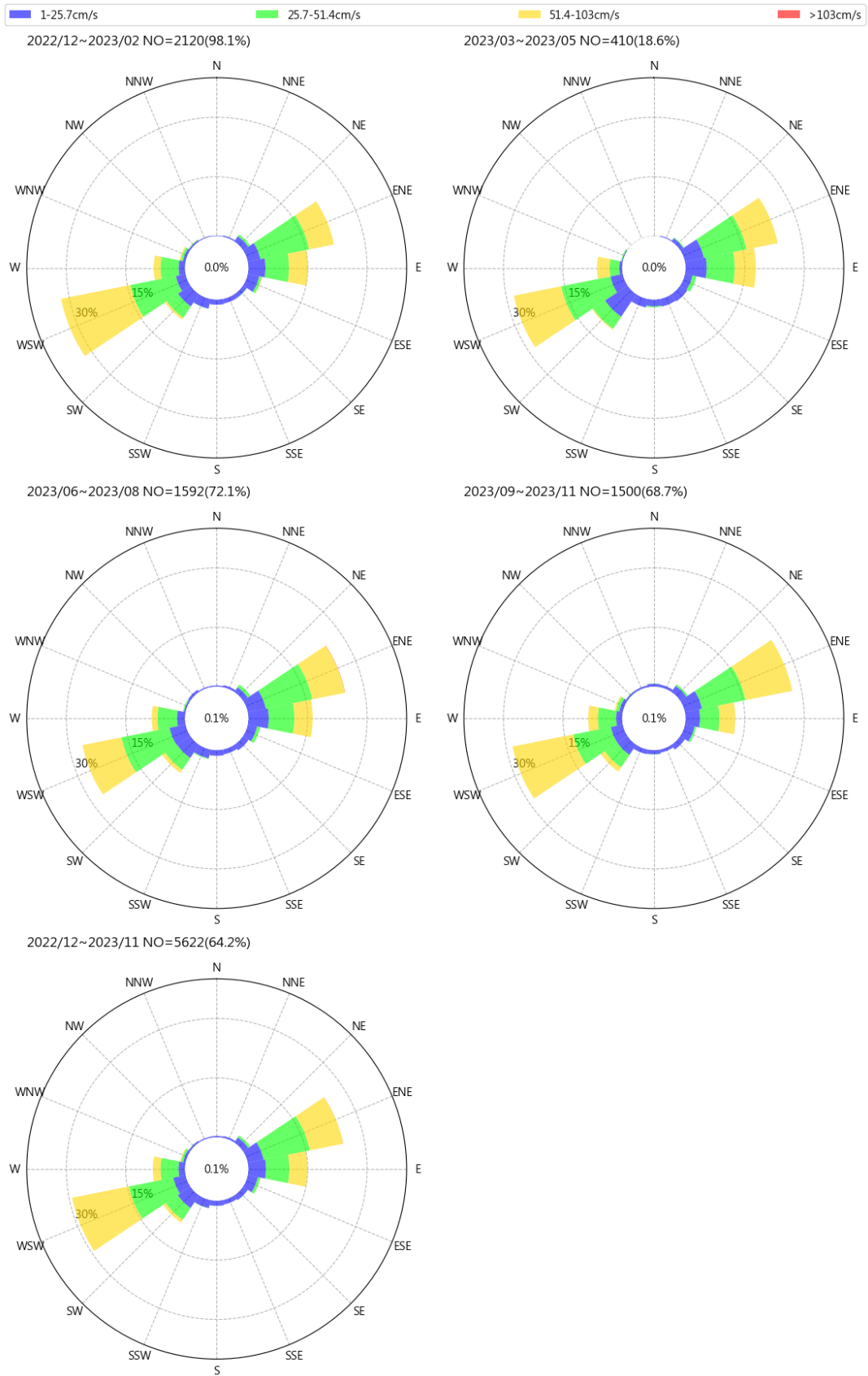
圖 2.6 2023 年臺北港每季流速流向玫瑰圖
