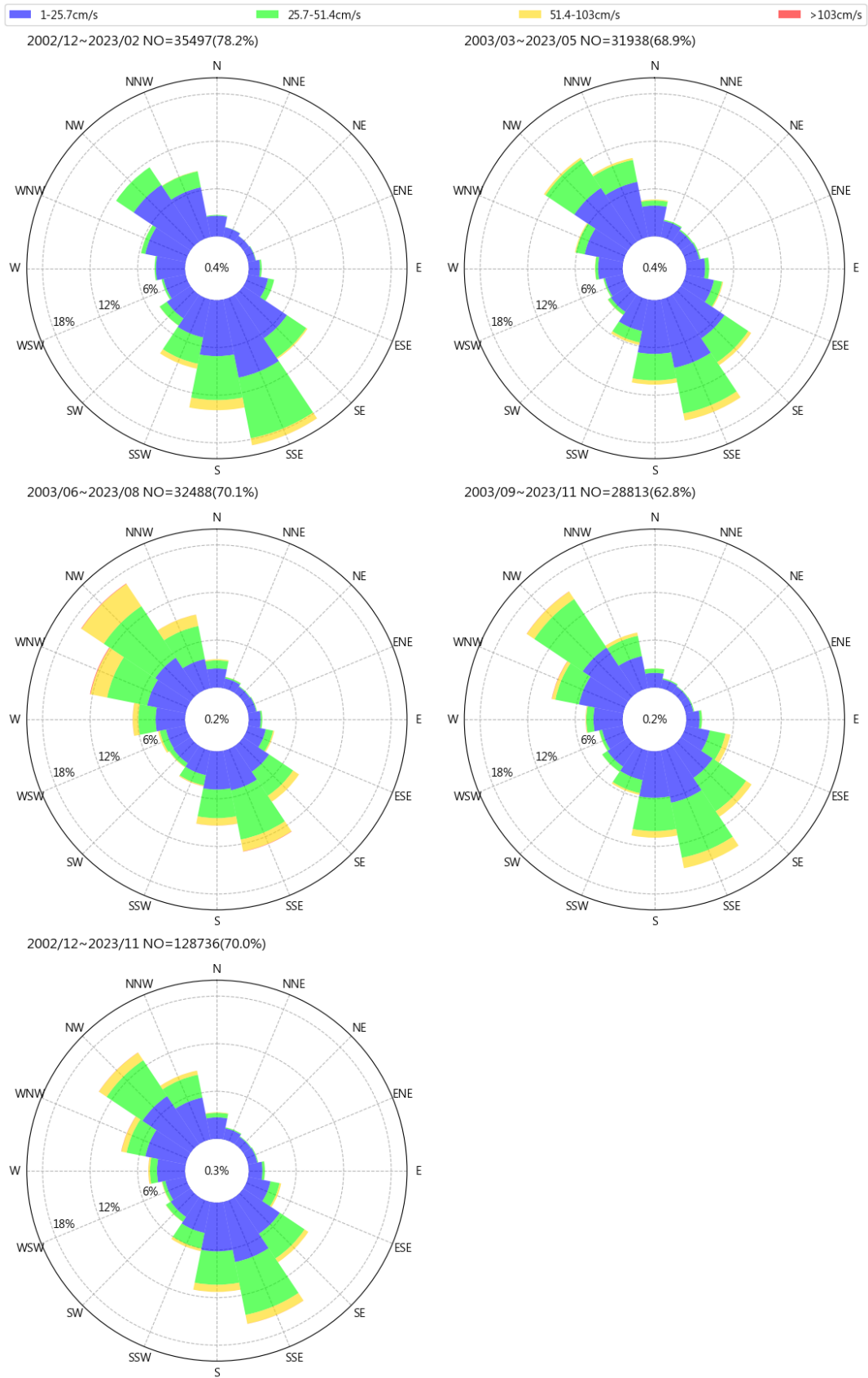
圖 7.8 歷年安平港每季流速流向玫瑰圖
