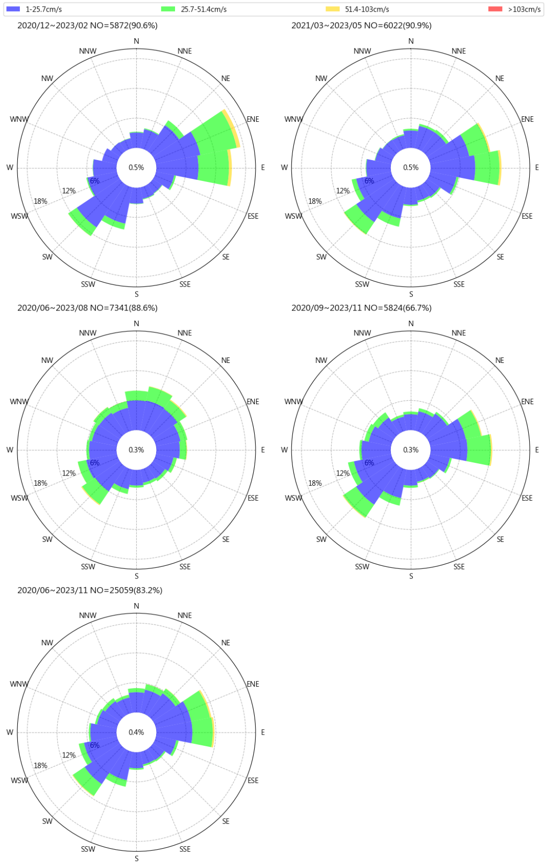
圖 3.8 歷年基隆港每季流速流向玫瑰圖
