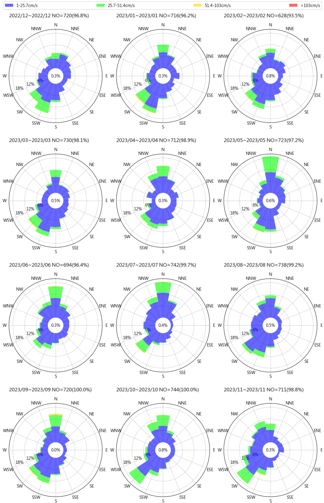
圖 4.5 2023 年蘇澳港每月流速流向玫瑰圖
