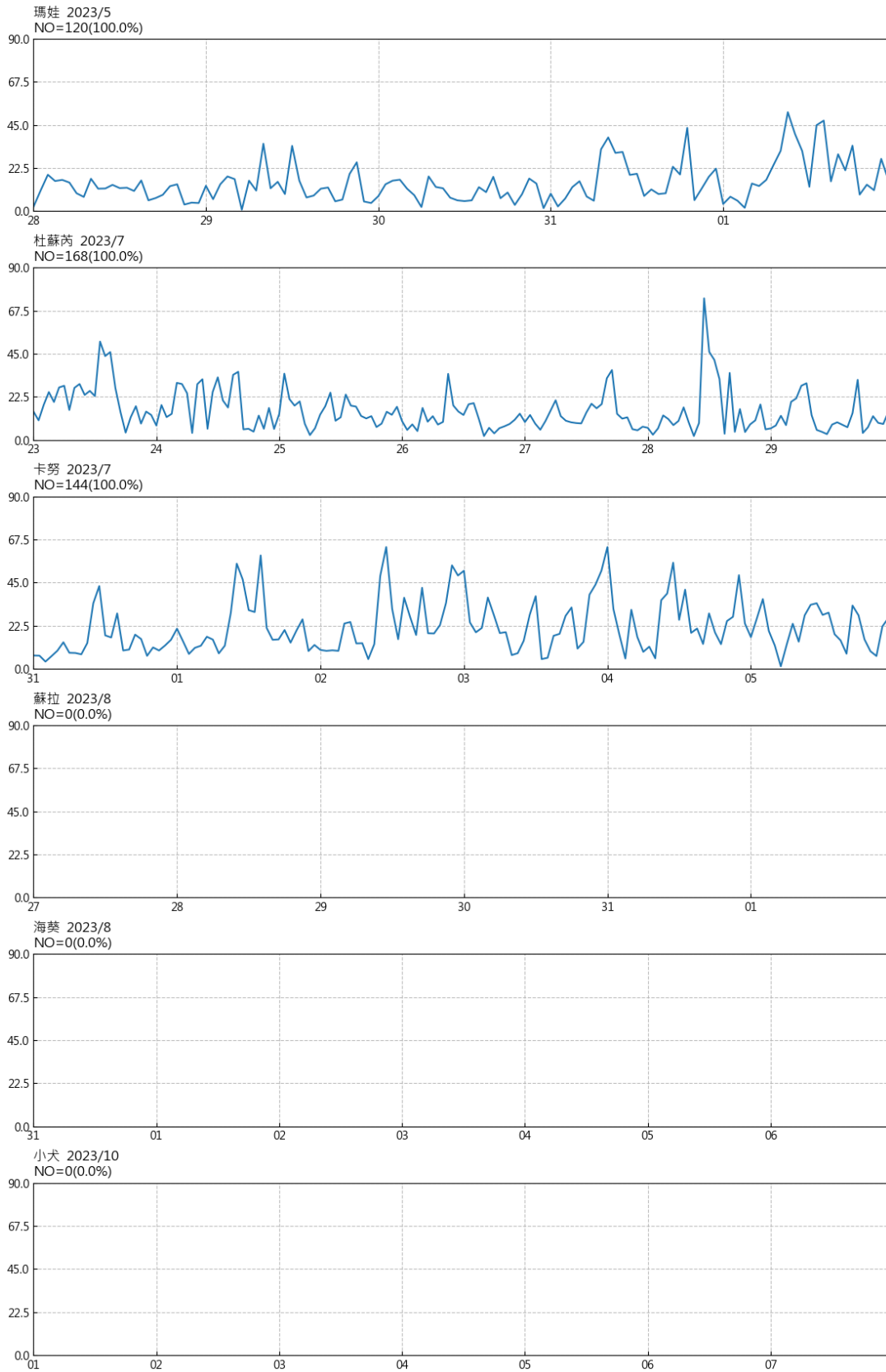
圖 3.9 2023 年基隆港颱風期間流速歷線圖
