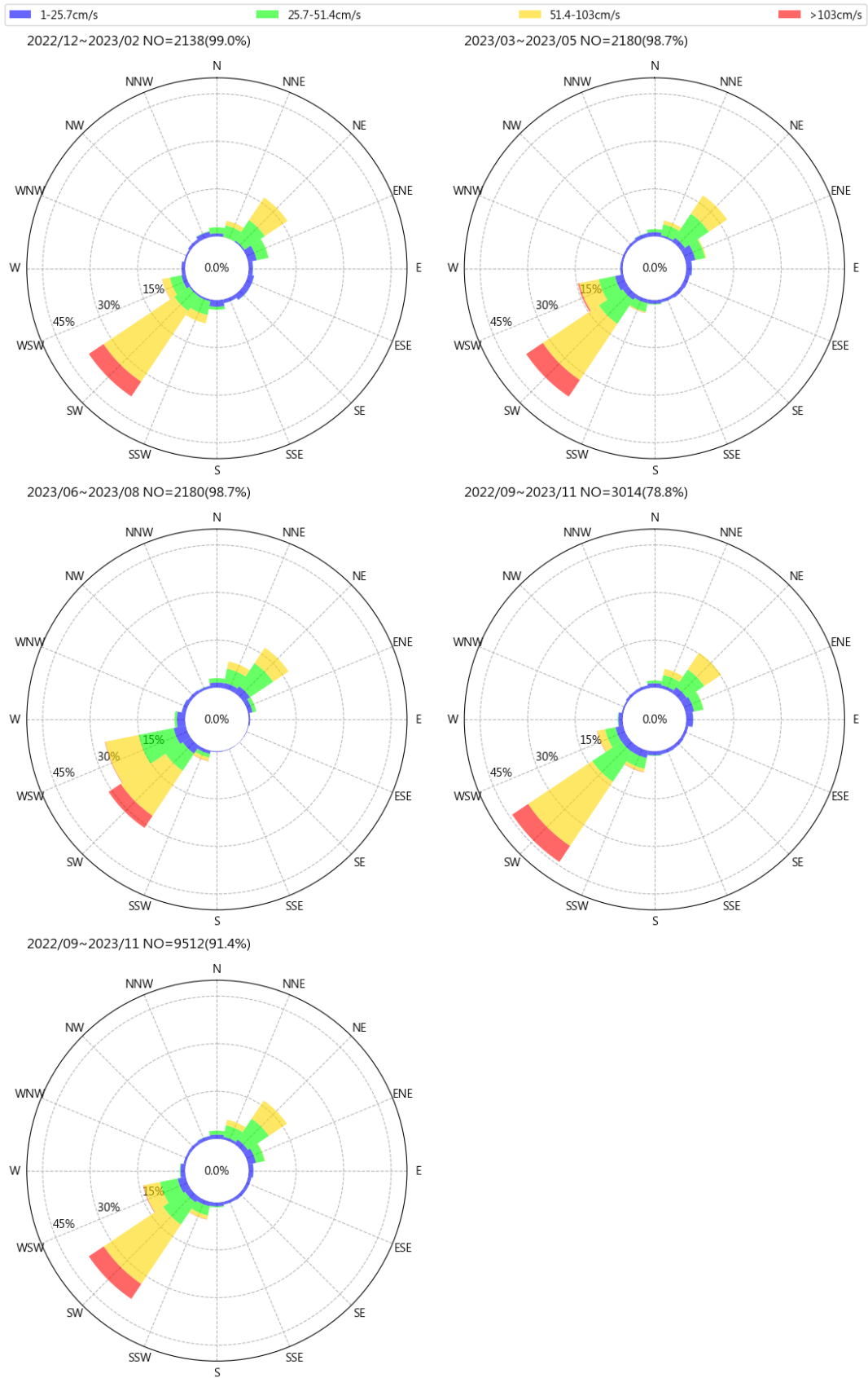
圖 11.8 歷年金門水頭港每季流速流向玫瑰圖
