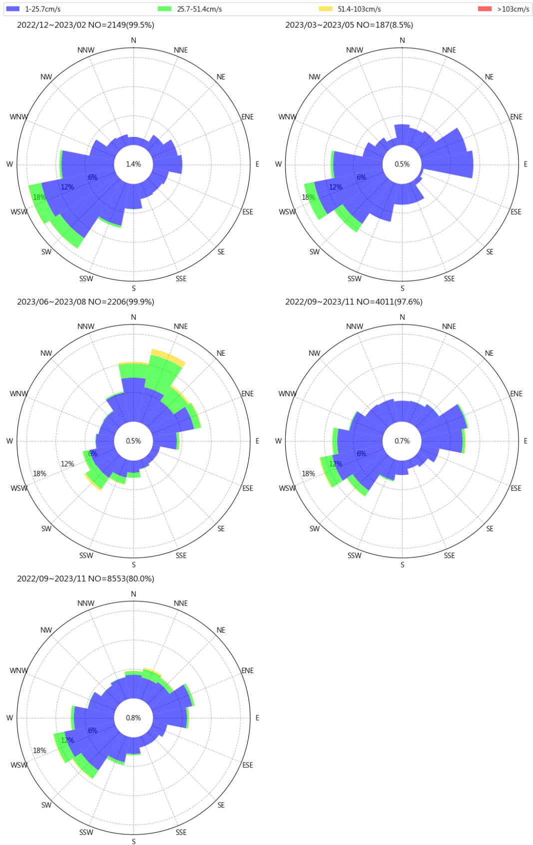
圖 12.8 歷年馬祖南竿福澳港每季流速流向玫瑰圖
