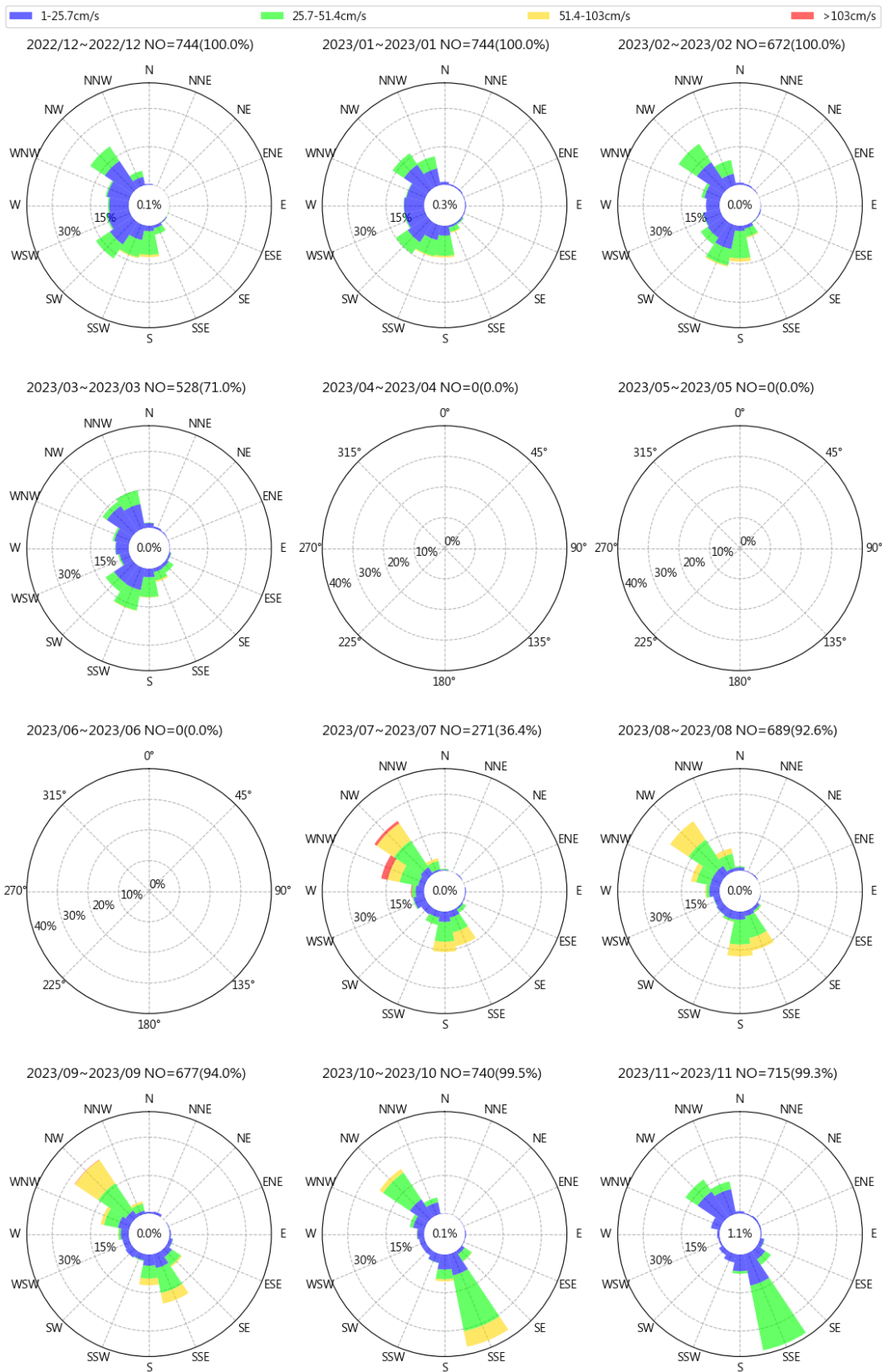
圖 7.5 2023 年安平港每月流速流向玫瑰圖
