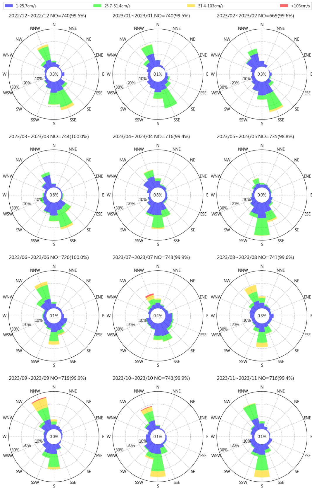
圖 6.5 2023 年高雄港每月流速流向玫瑰圖
