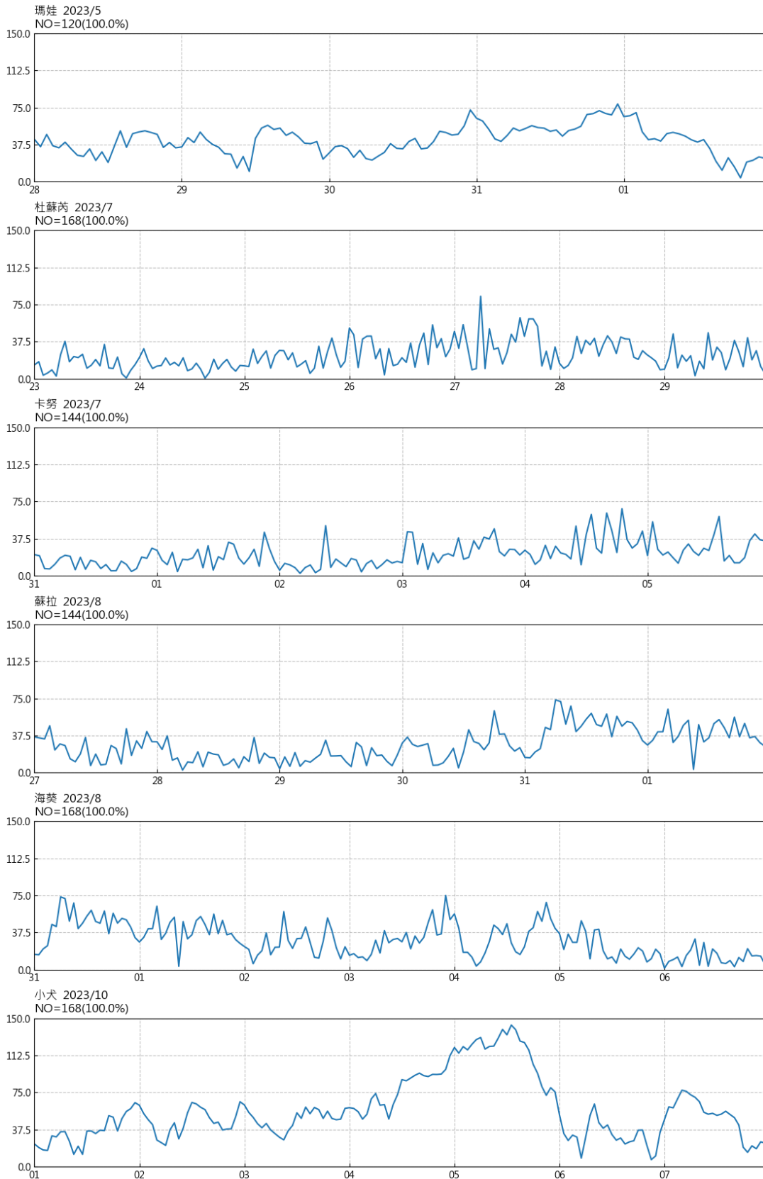
圖 9.9 2023 年臺中港颱風期間流速歷線圖
