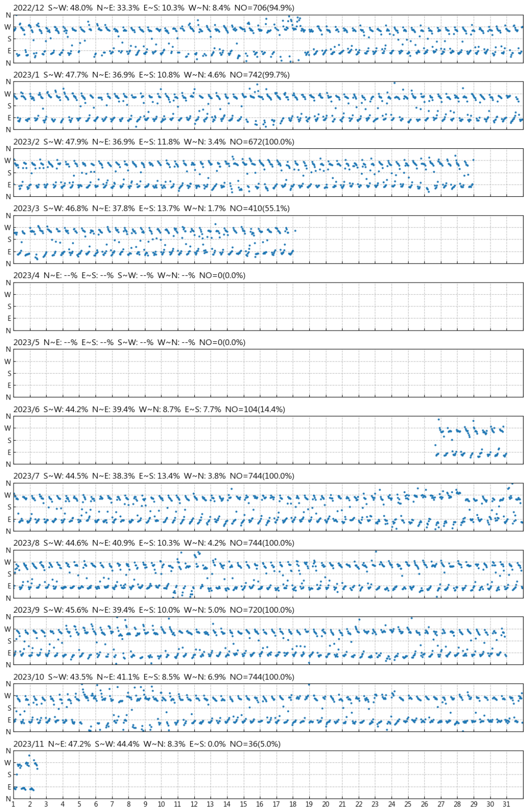
圖 2.4 2023 年臺北港每月流向歷線圖
