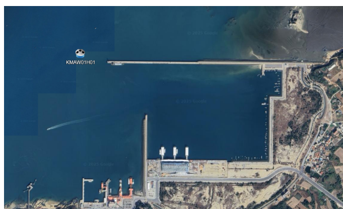
圖 11.1 金門水頭港海流觀測站位置示意圖
