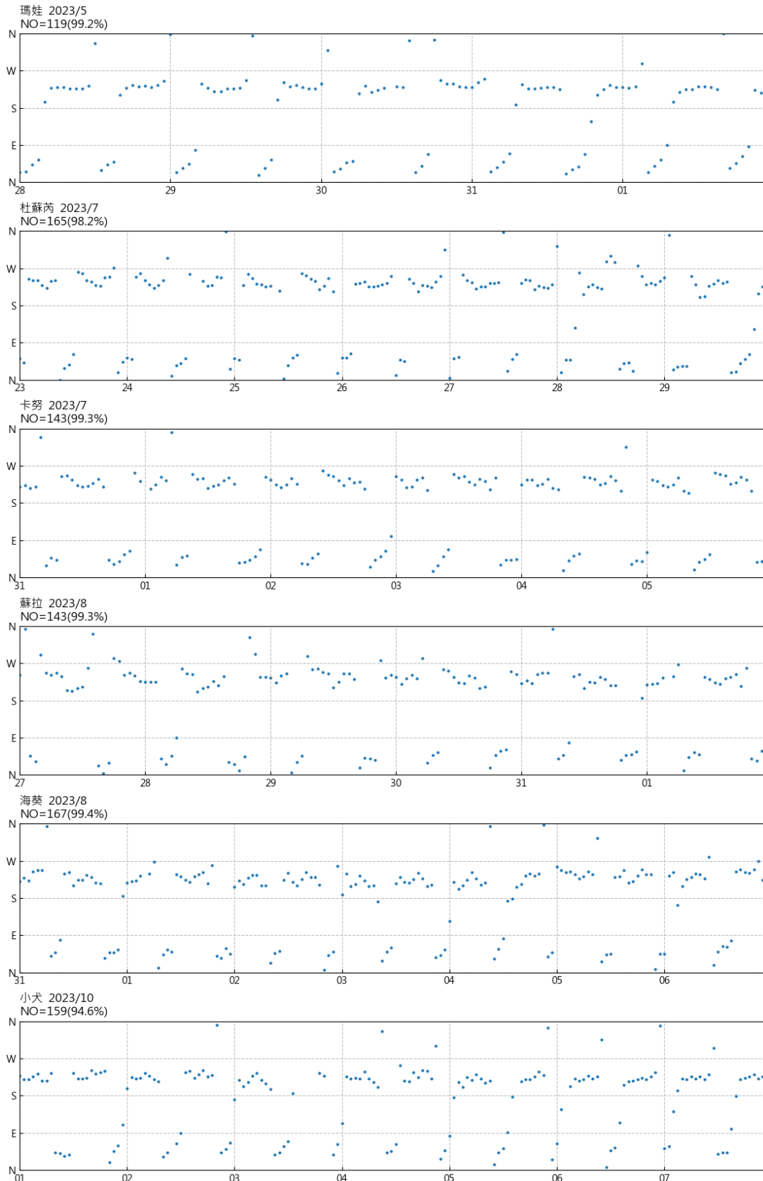
圖 11.10 2023 年金門水頭港颱風期間流向歷線圖
