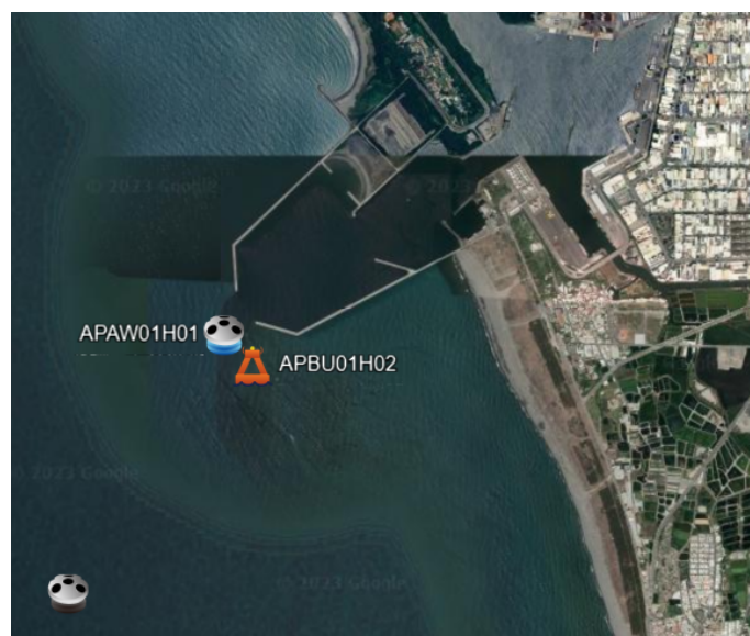
圖 7.1 安平港海流觀測站位置示意圖
