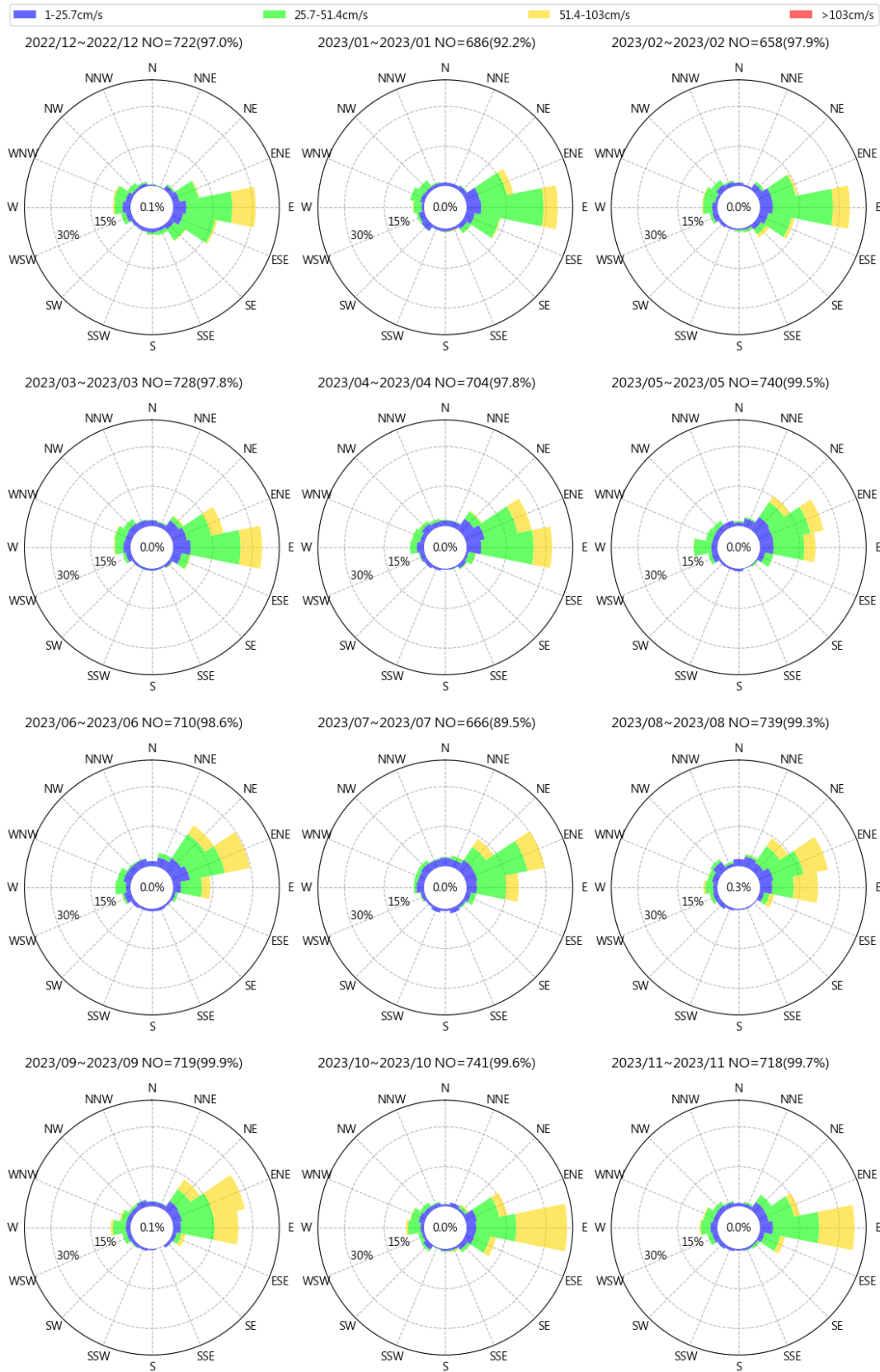
圖 10.5 2023 年澎湖龍門尖山港每月流速流向玫瑰圖
