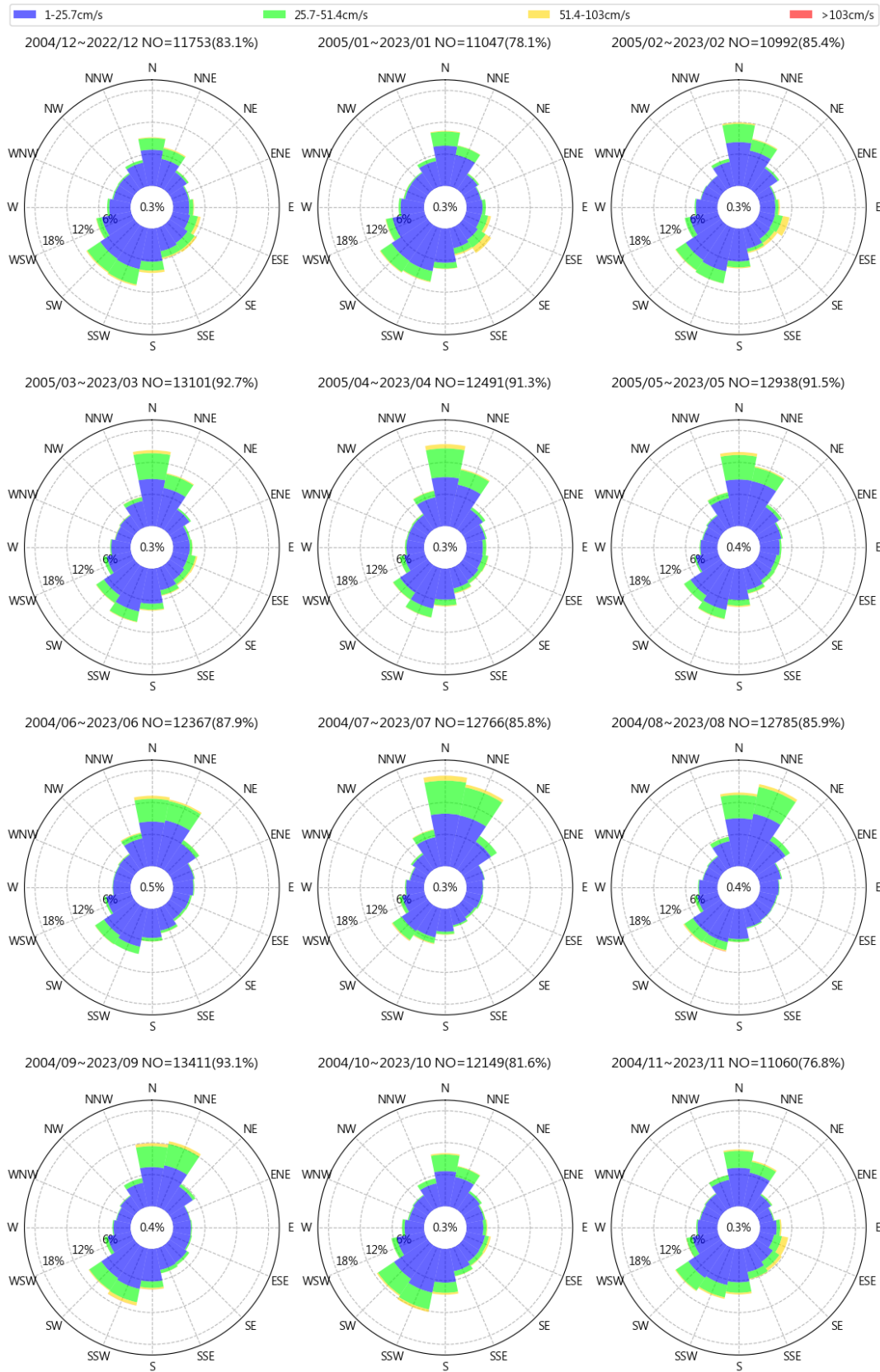
圖 4.7 歷年蘇澳港每月流速流向玫瑰圖
