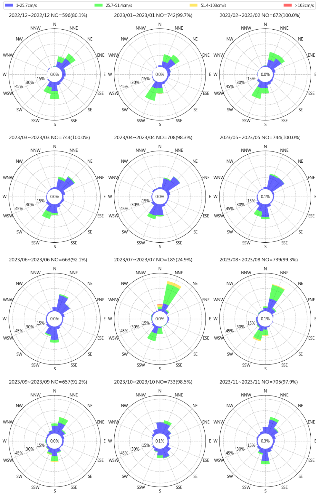
圖 8.5 2023 年布袋港每月流速流向玫瑰圖
