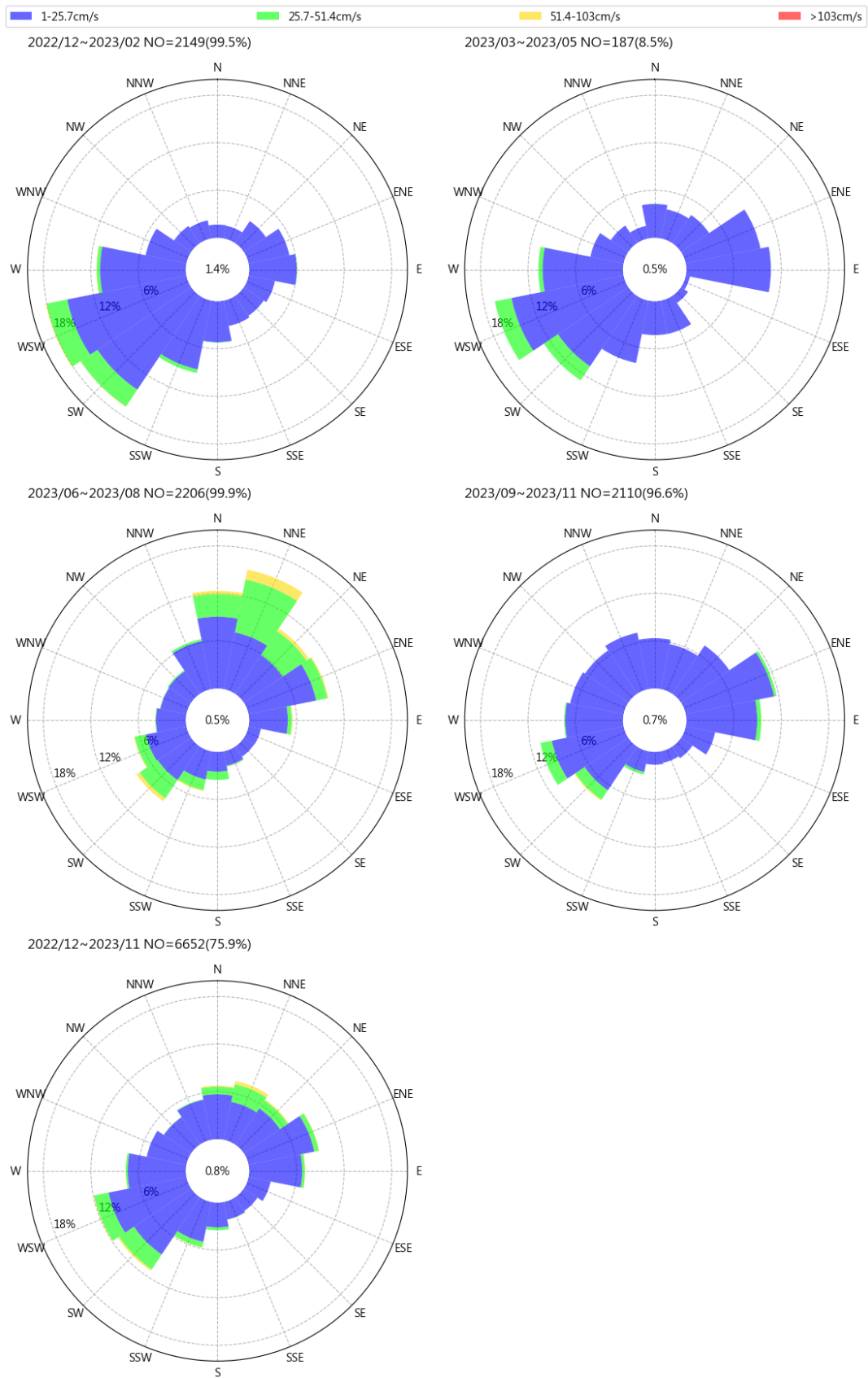
圖 12.6 2023 年馬祖南竿福澳港每季流速流向玫瑰圖
