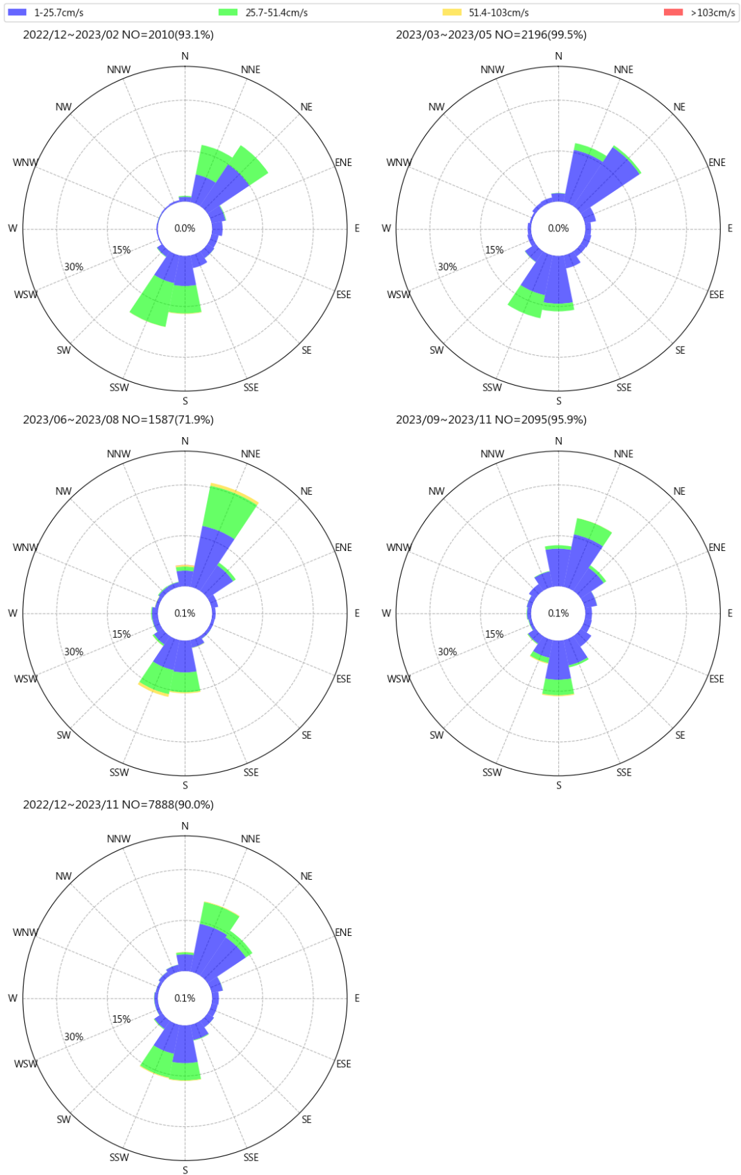
圖 8.6 2023 年布袋港每季流速流向玫瑰圖
