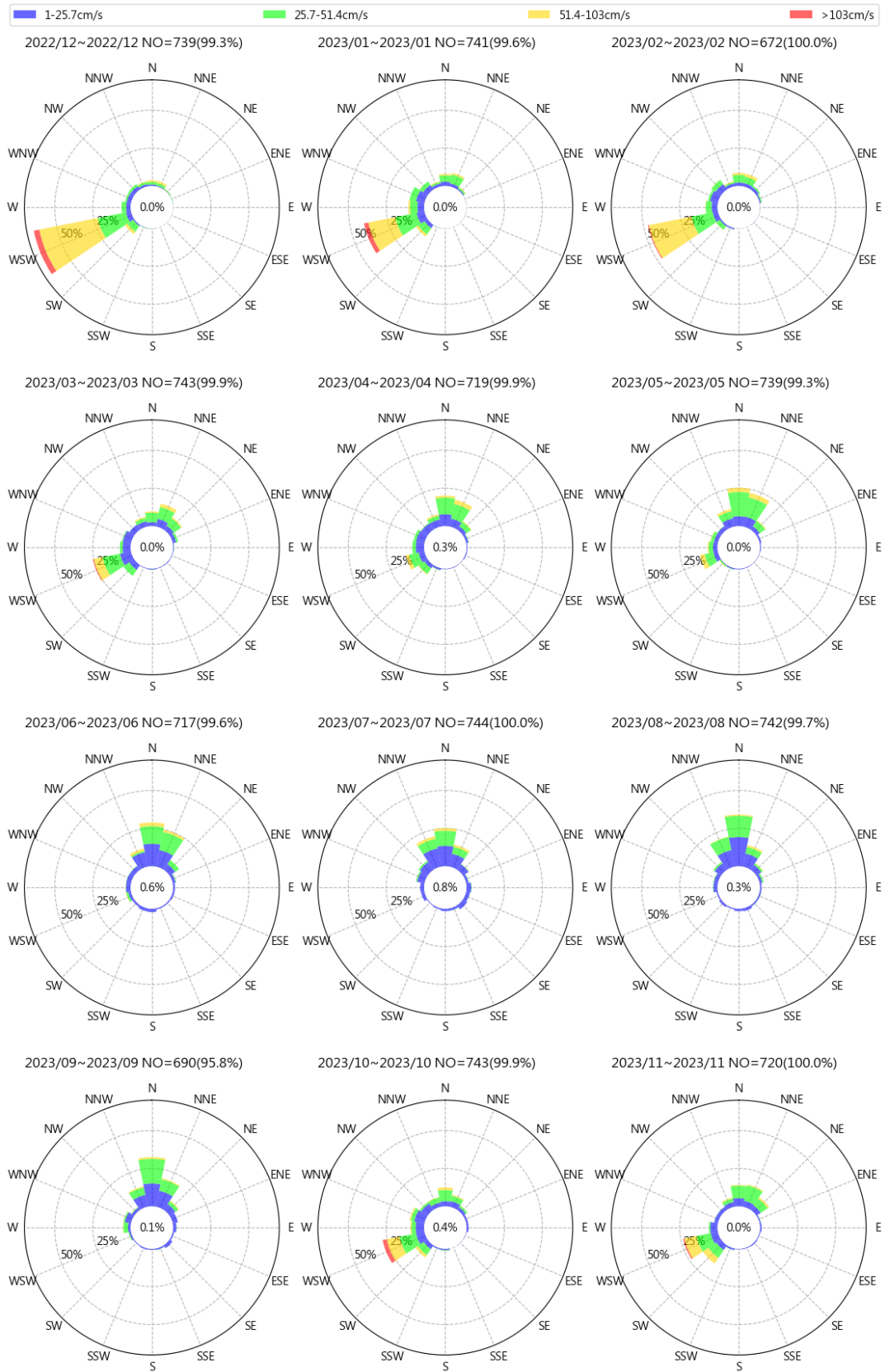
圖 9.5 2023 年臺中港每月流速流向玫瑰圖
