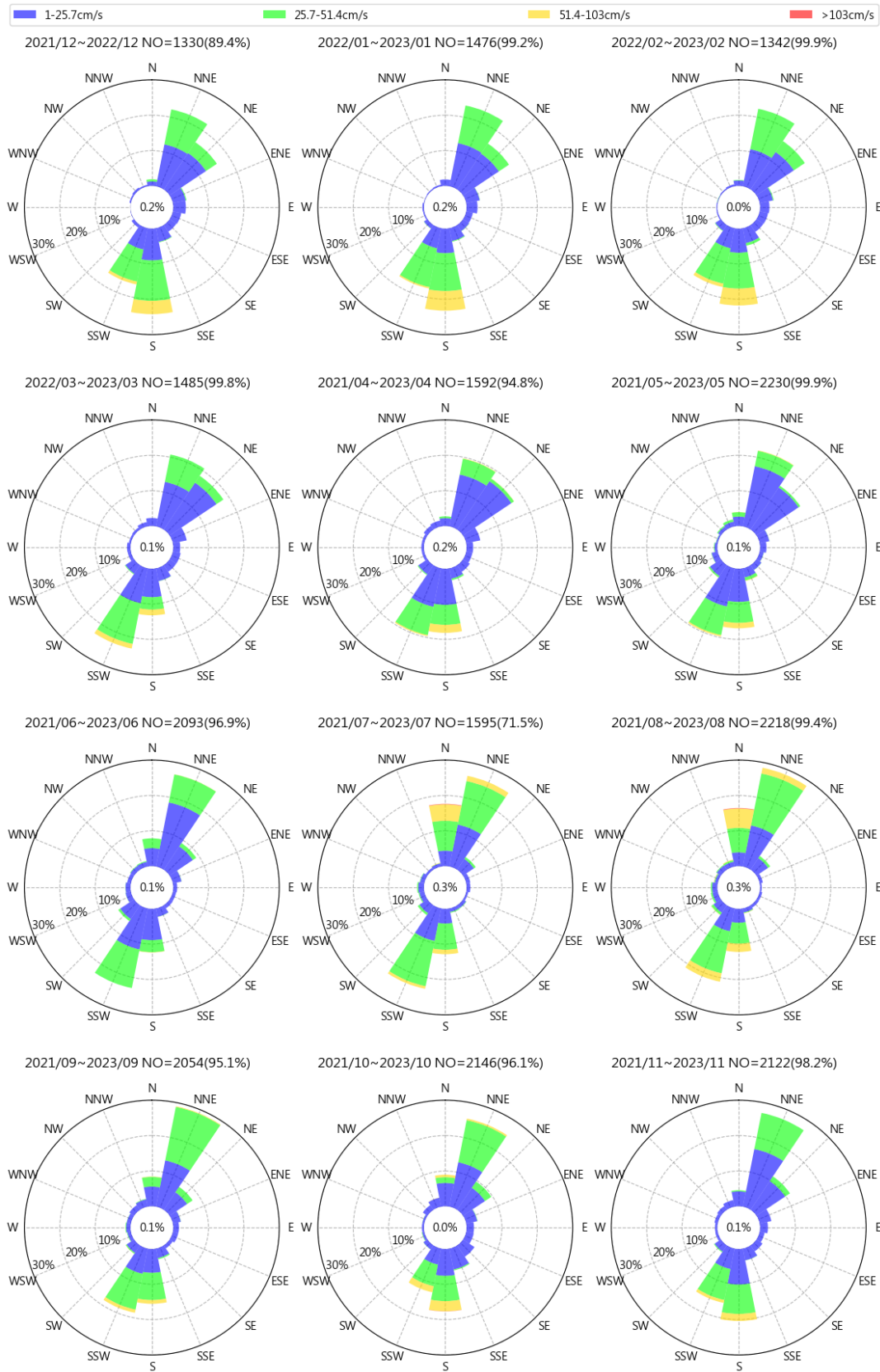
圖 8.7 歷年布袋港每月流速流向玫瑰圖
