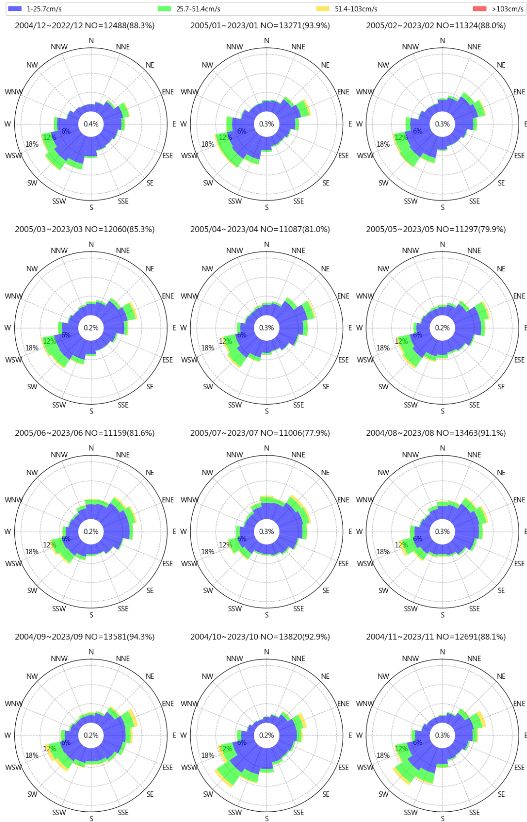
圖 5.7 歷年花蓮港每月流速流向玫瑰圖
