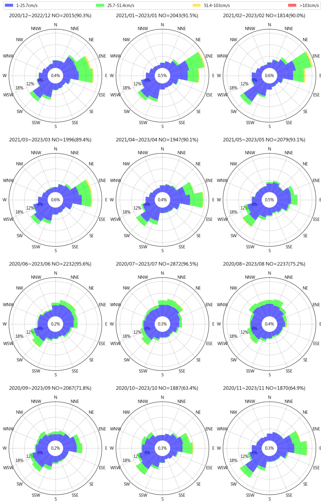
圖 3.7 歷年基隆港每月流速流向玫瑰圖
