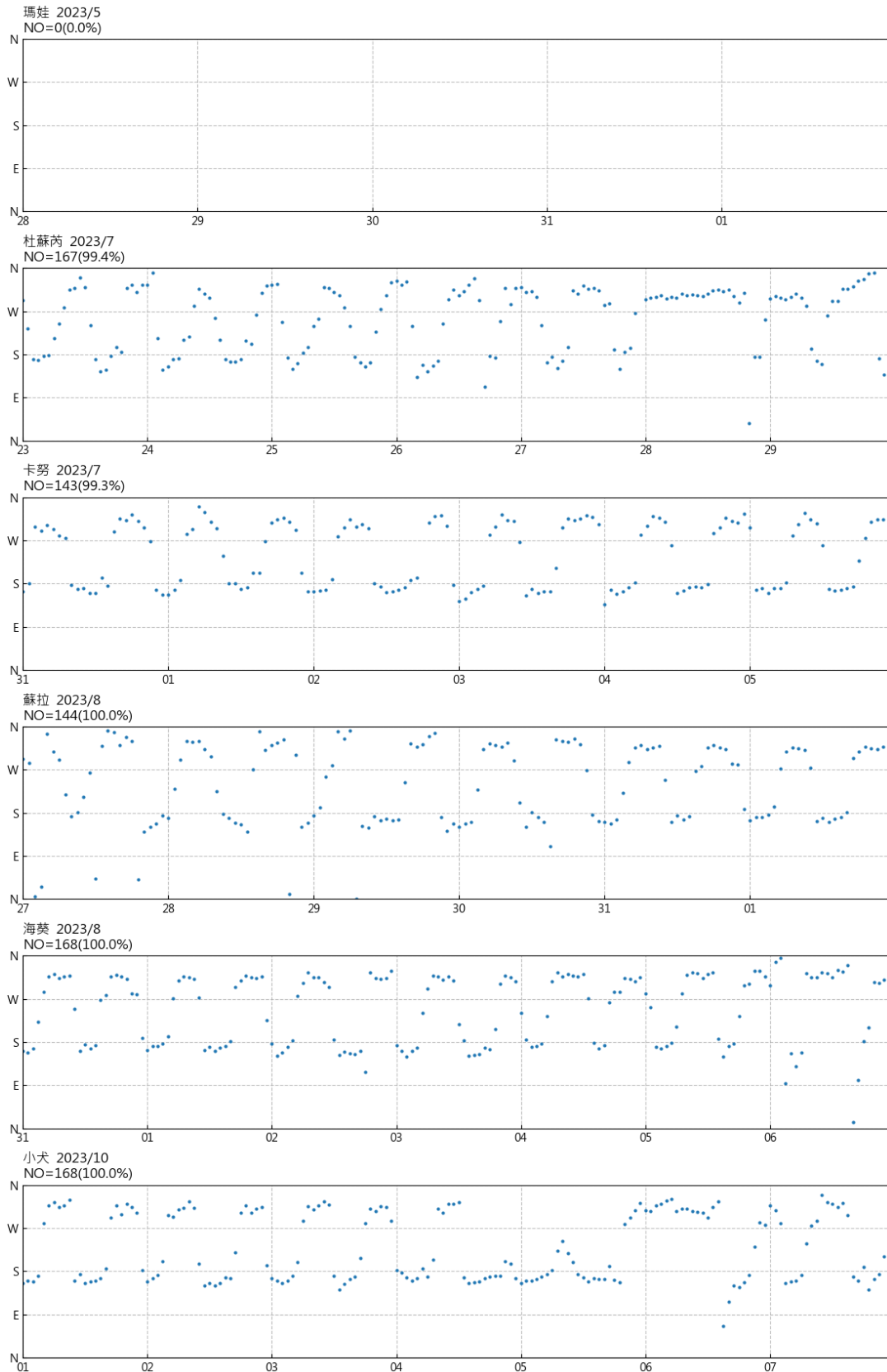
圖 7.10 2023 年安平港颱風期間流向歷線圖
