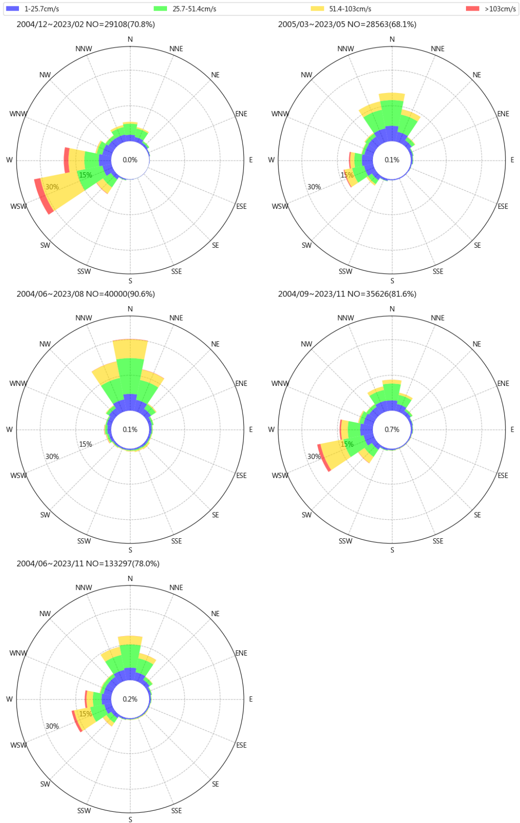
圖 9.8 歷年臺中港每季流速流向玫瑰圖
