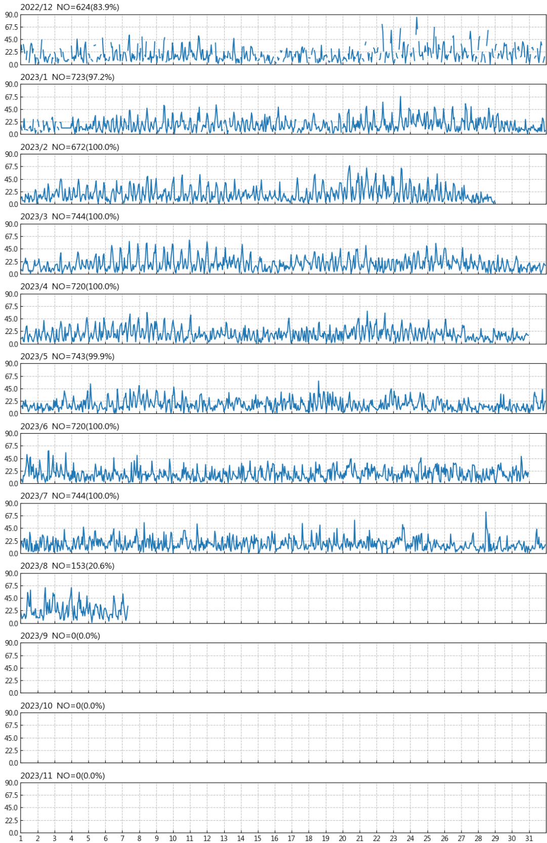
圖 3.3 2023 年基隆港每月流速歷線圖
