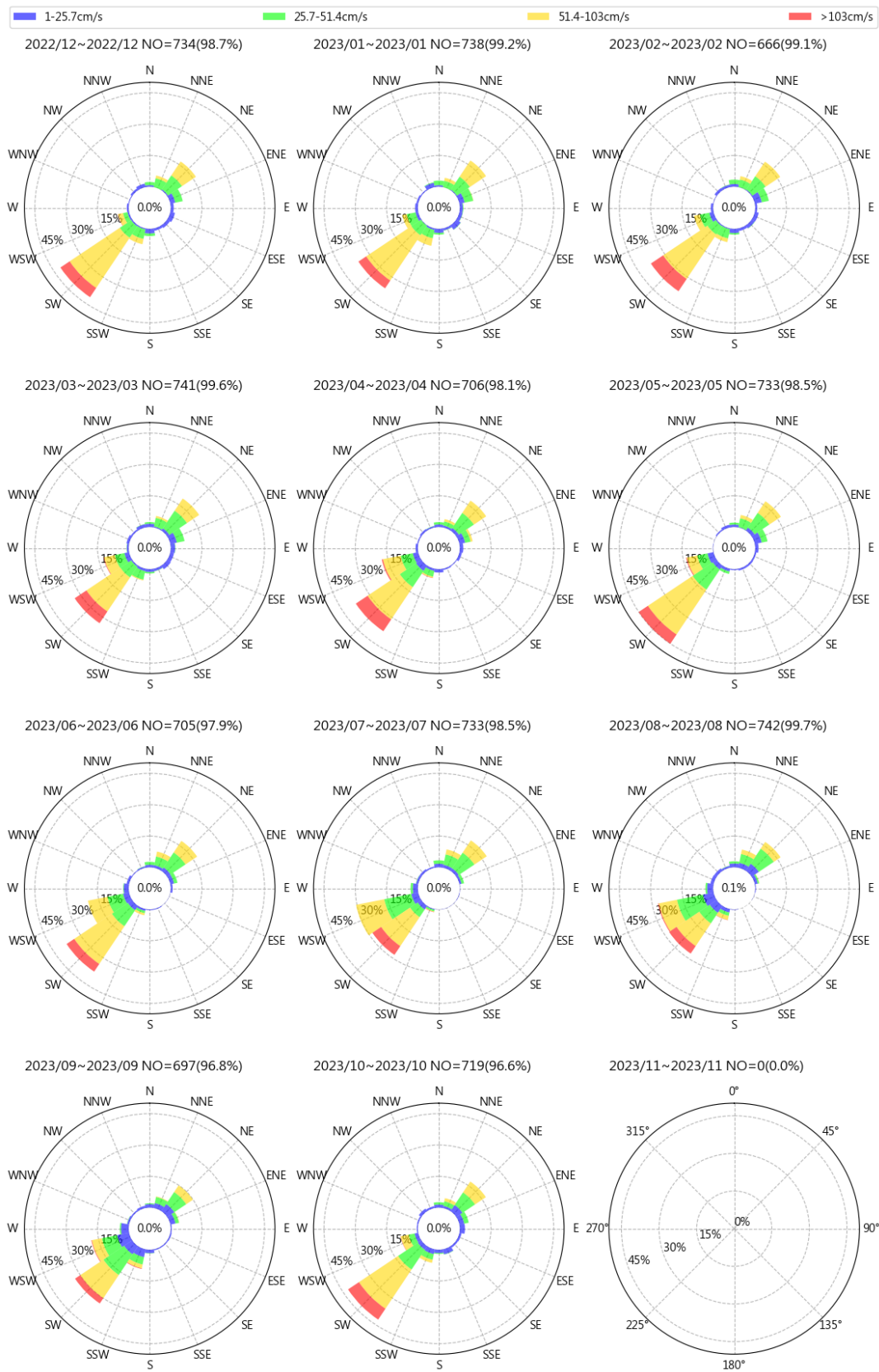
圖 11.5 2023 年金門水頭港每月流速流向玫瑰圖
