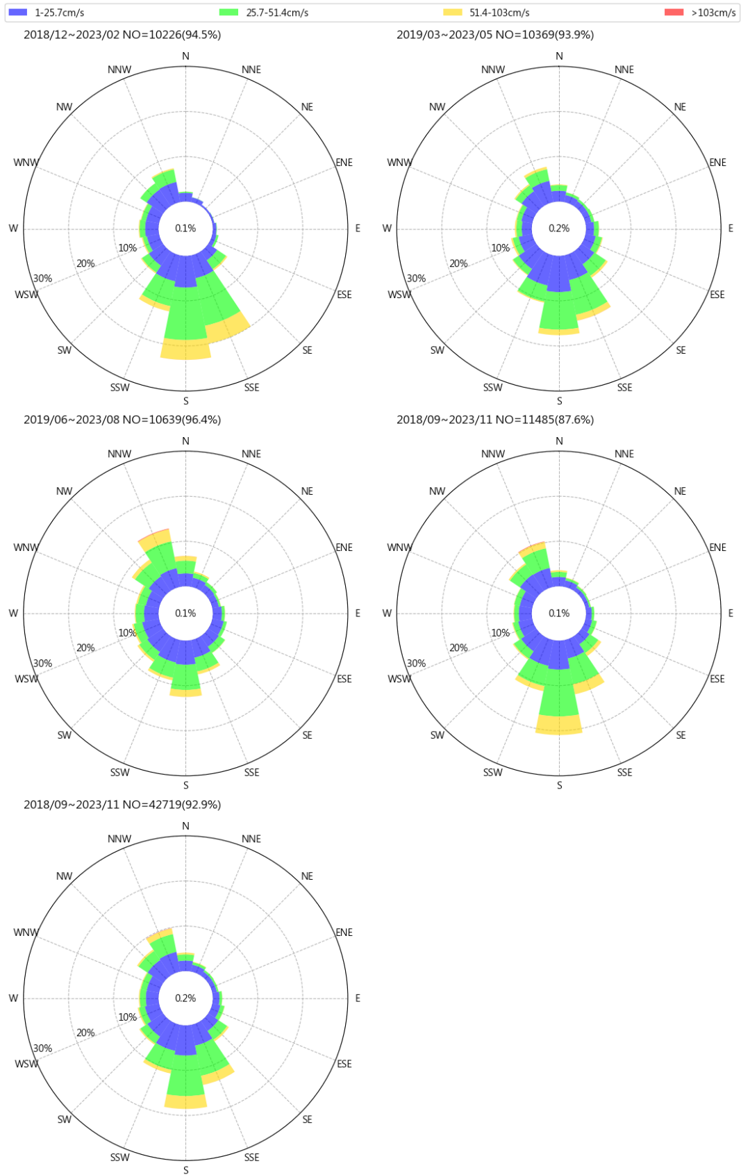
圖 6.8 歷年高雄港每季流速流向玫瑰圖
