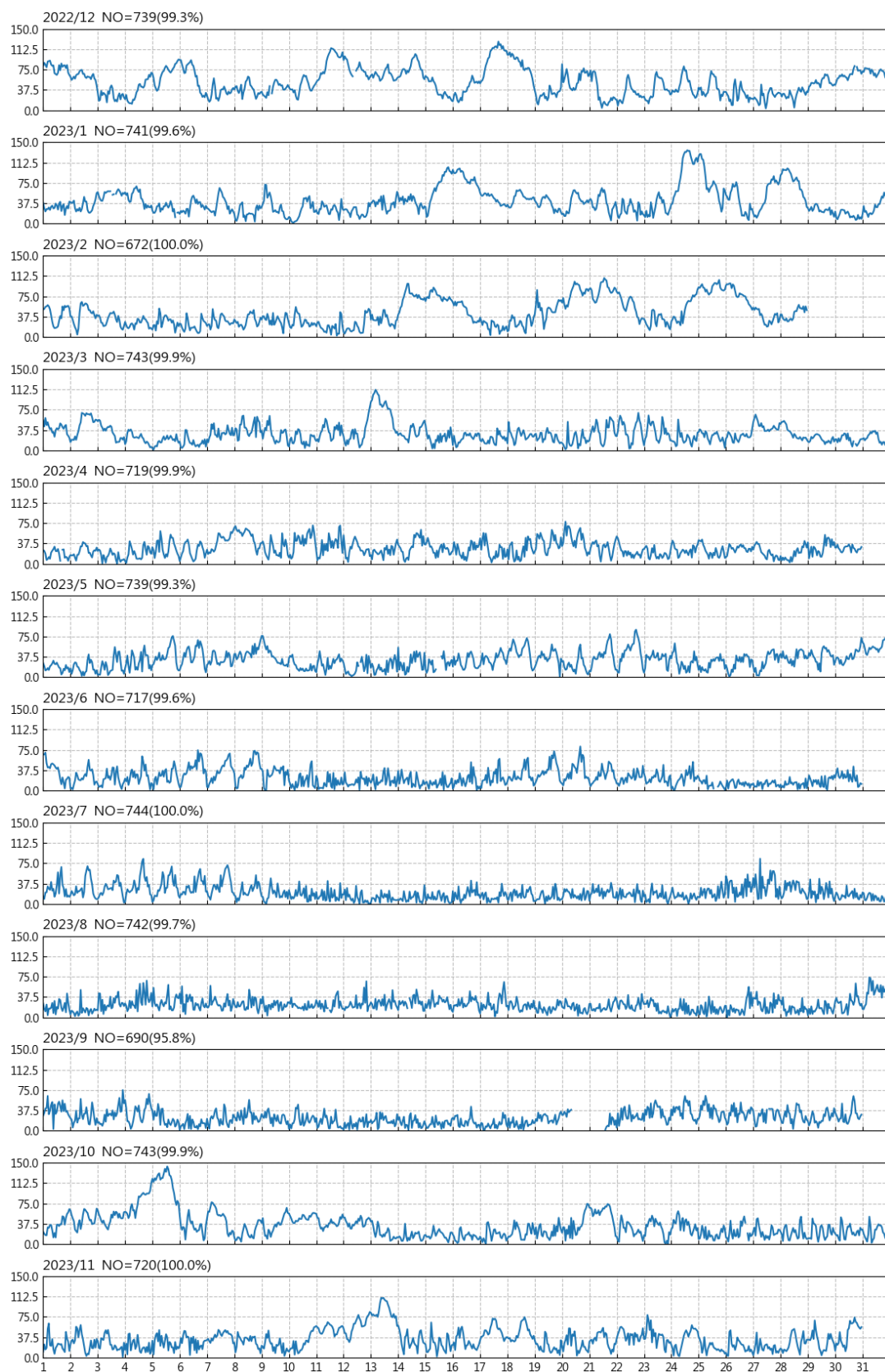
圖 9.3 2023 年臺中港每月流速歷線圖
