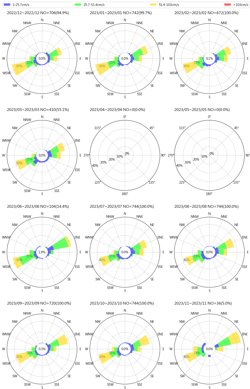
圖 2.5 2023 年臺北港每月流速流向玫瑰圖
