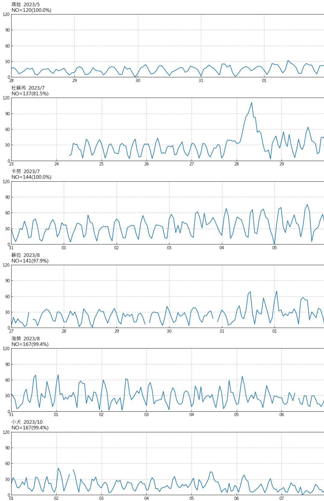
圖 8.9 2023 年布袋港颱風期間流速歷線圖
