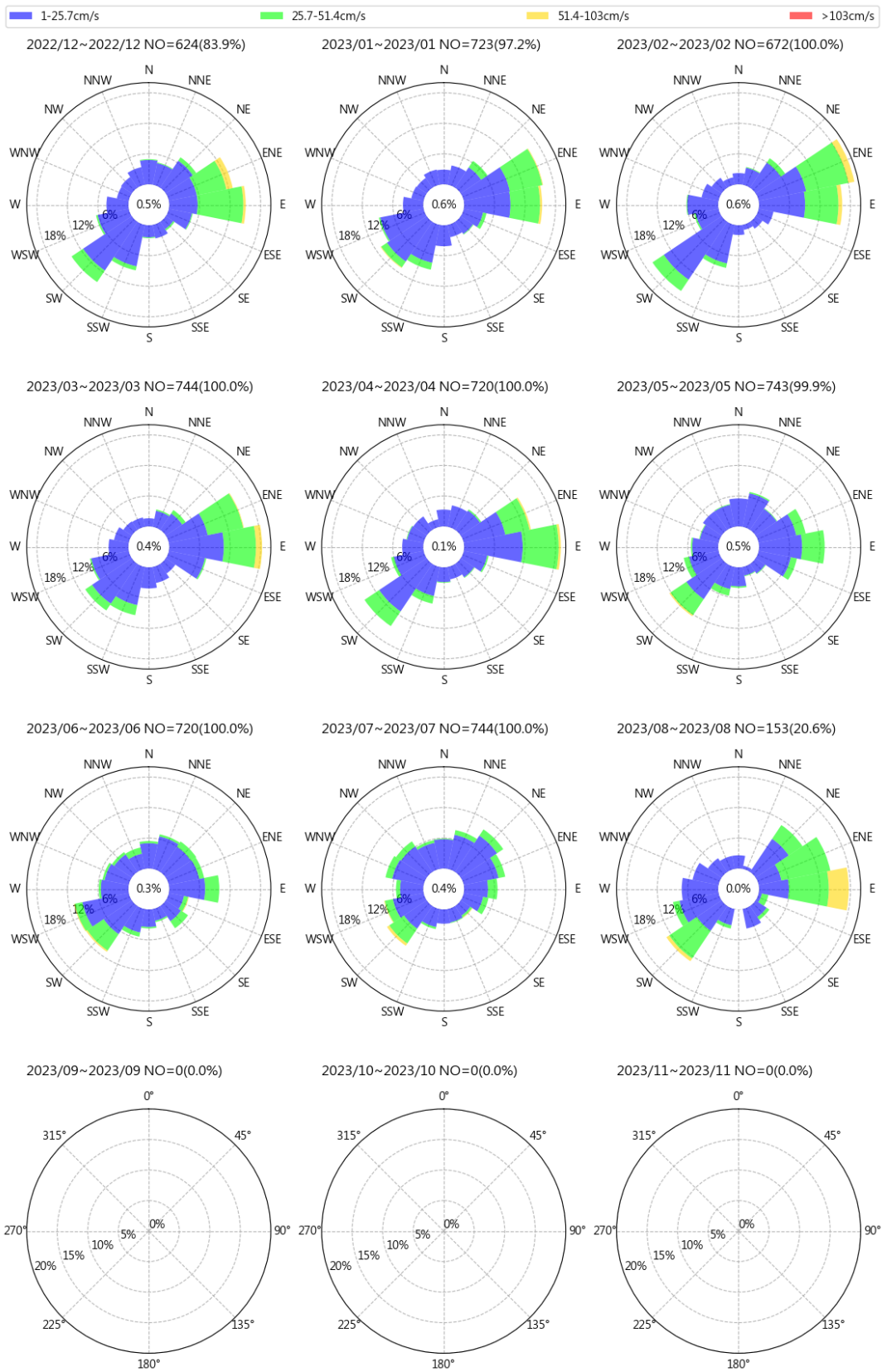
圖 3.5 2023 年基隆港每月流速流向玫瑰圖
