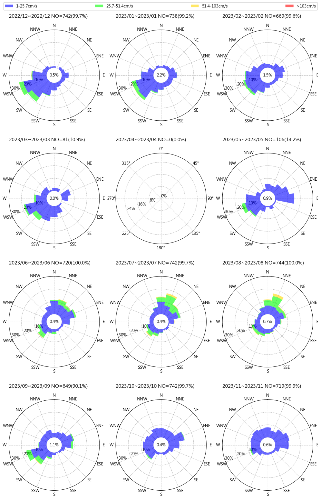
圖 12.5 2023 年馬祖南竿福澳港每月流速流向玫瑰圖
