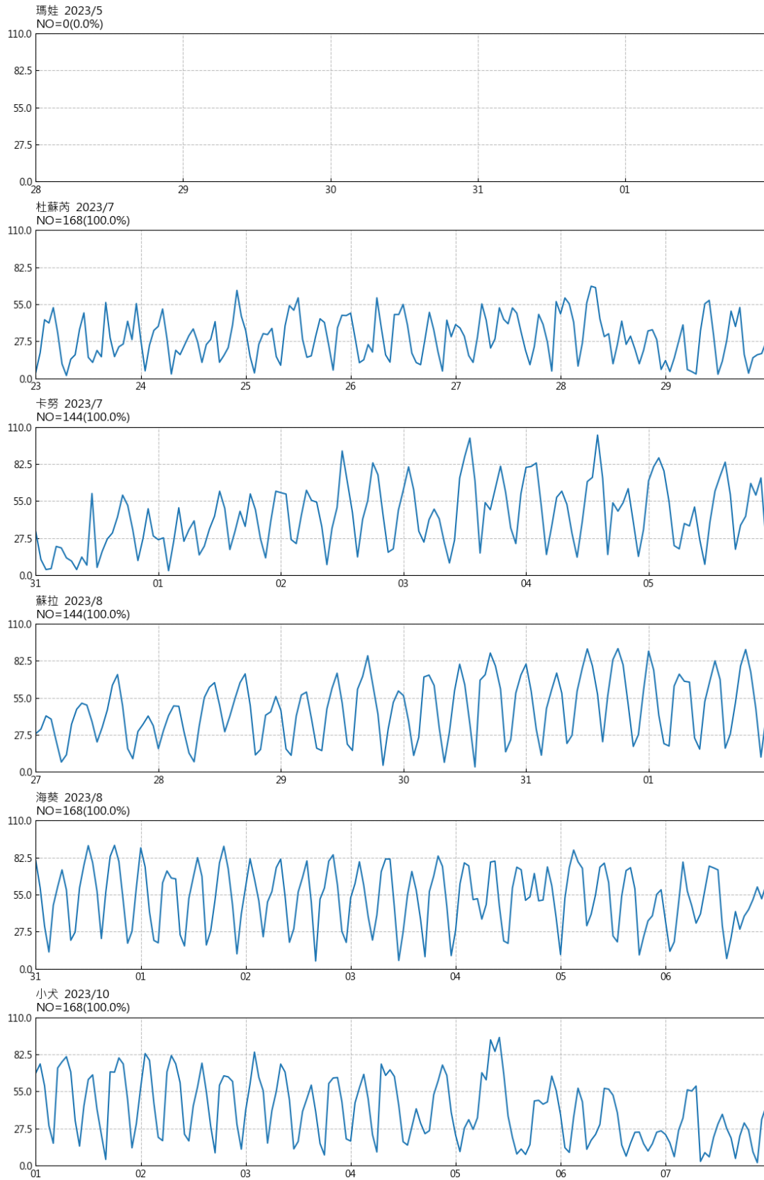
圖 2.9 2023 年臺北港颱風期間流速歷線圖
