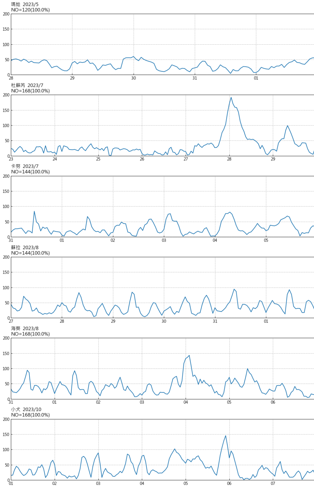
圖 6.9 2023 年高雄港颱風期間流速歷線圖
