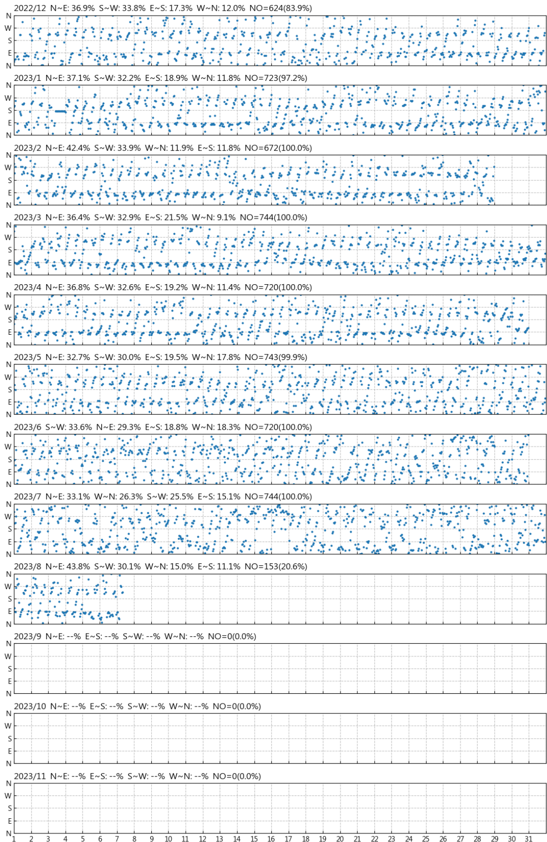
圖 3.4 2023 年基隆港每月流向歷線圖
