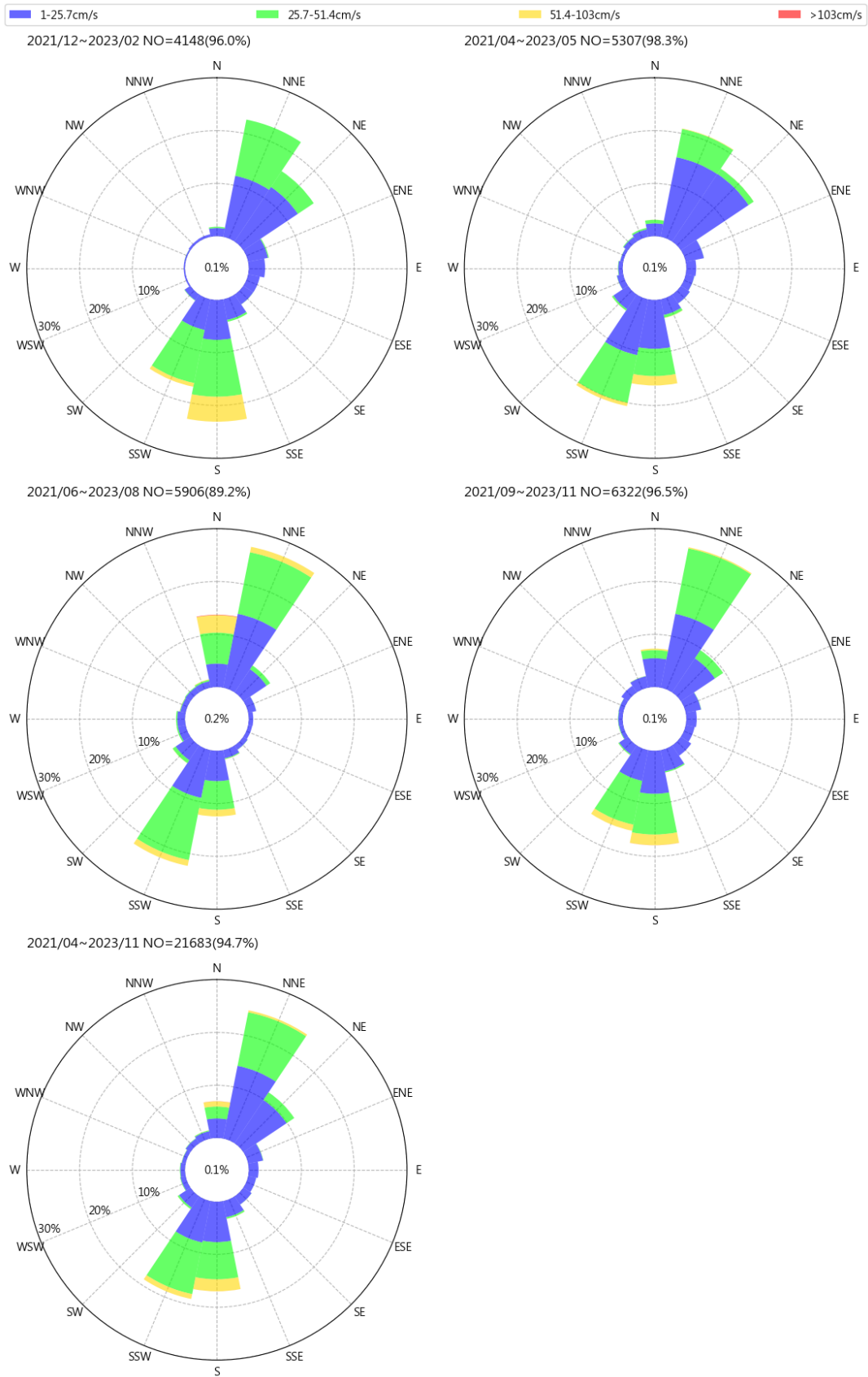
圖 8.8 歷年布袋港每季流速流向玫瑰圖
