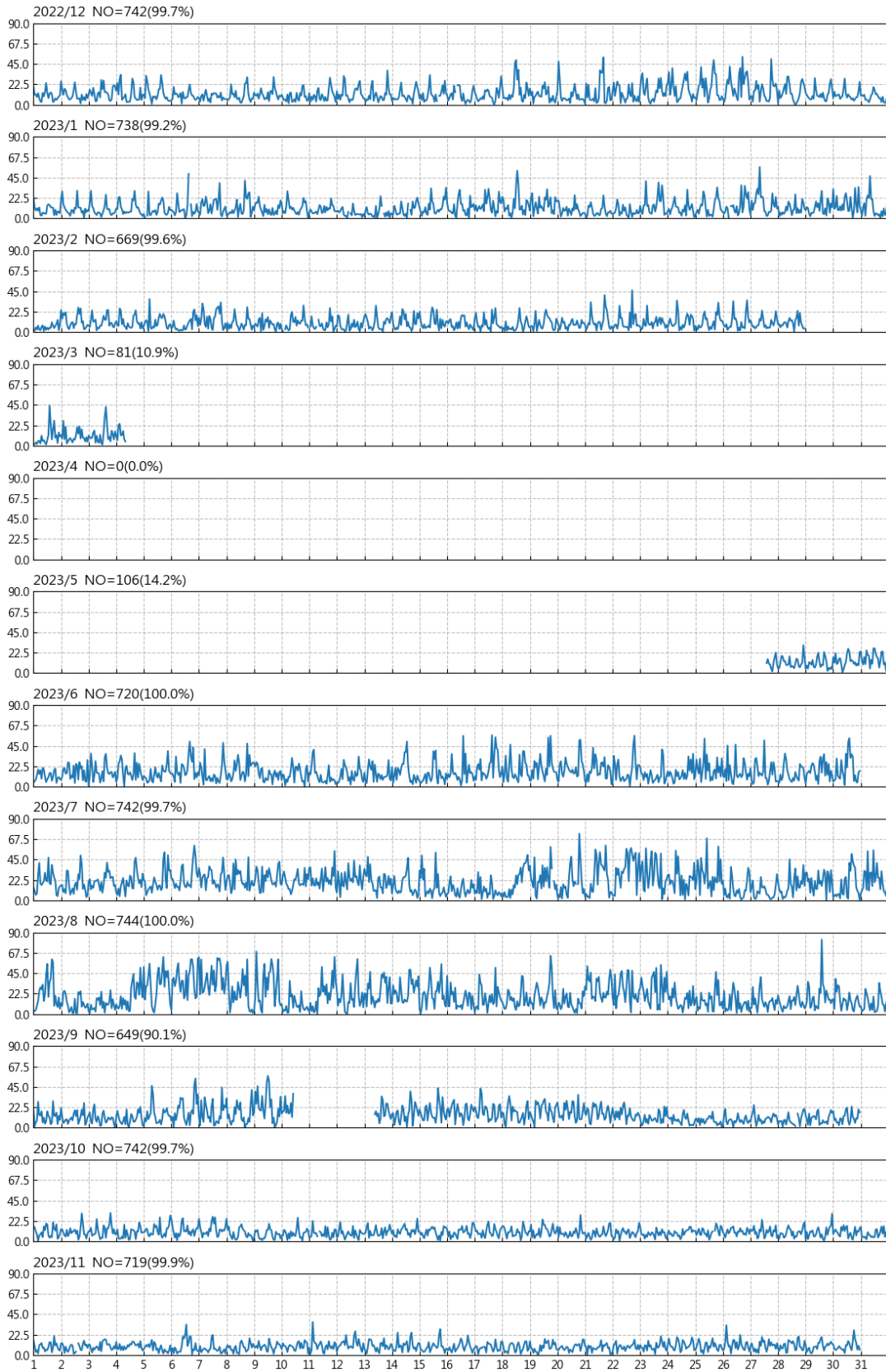
圖 12.3 2023 年馬祖南竿福澳港每月流速歷線圖
