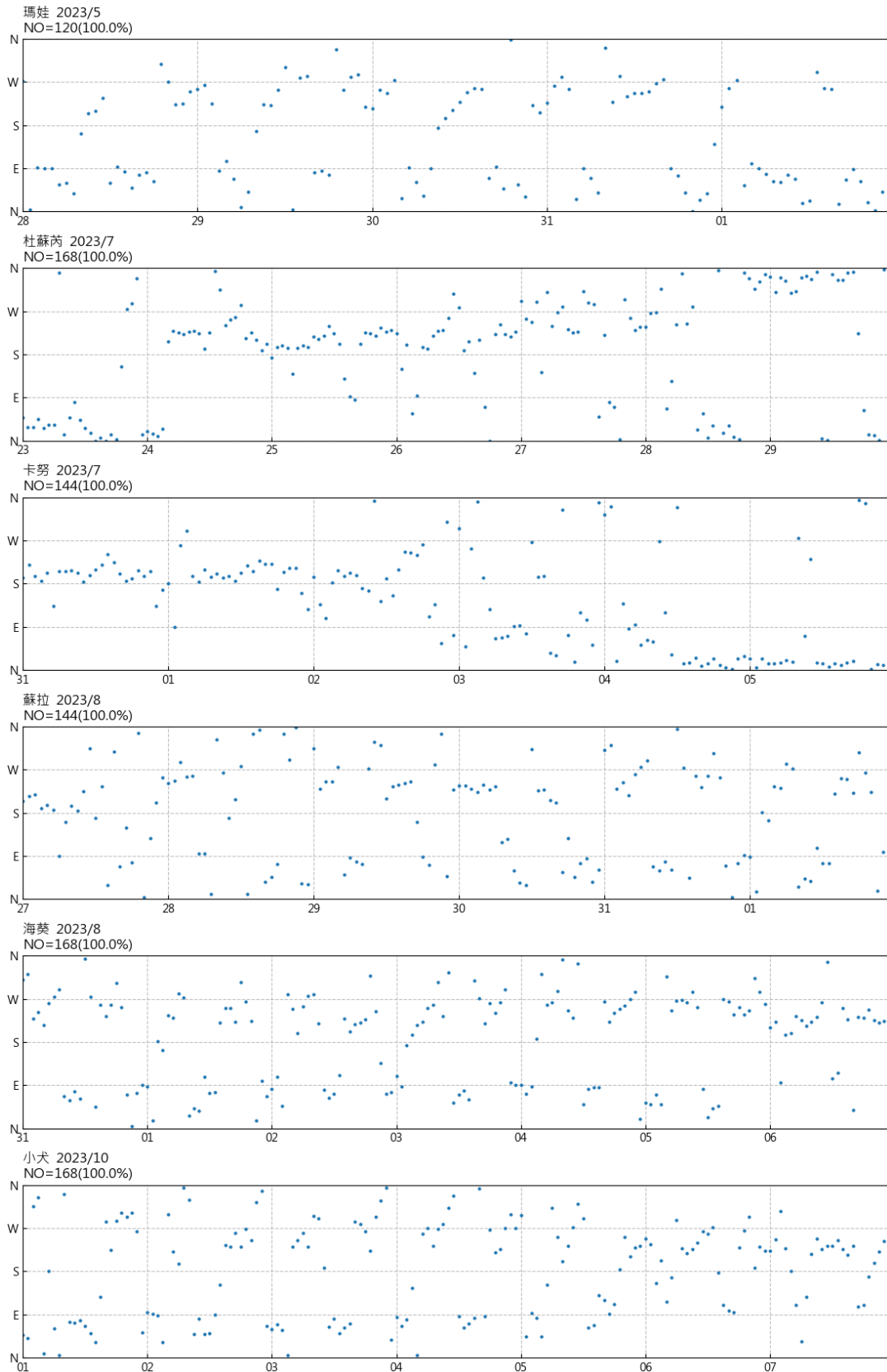
圖 12.10 2023 年馬祖南竿福澳港颱風期間流向歷線圖
