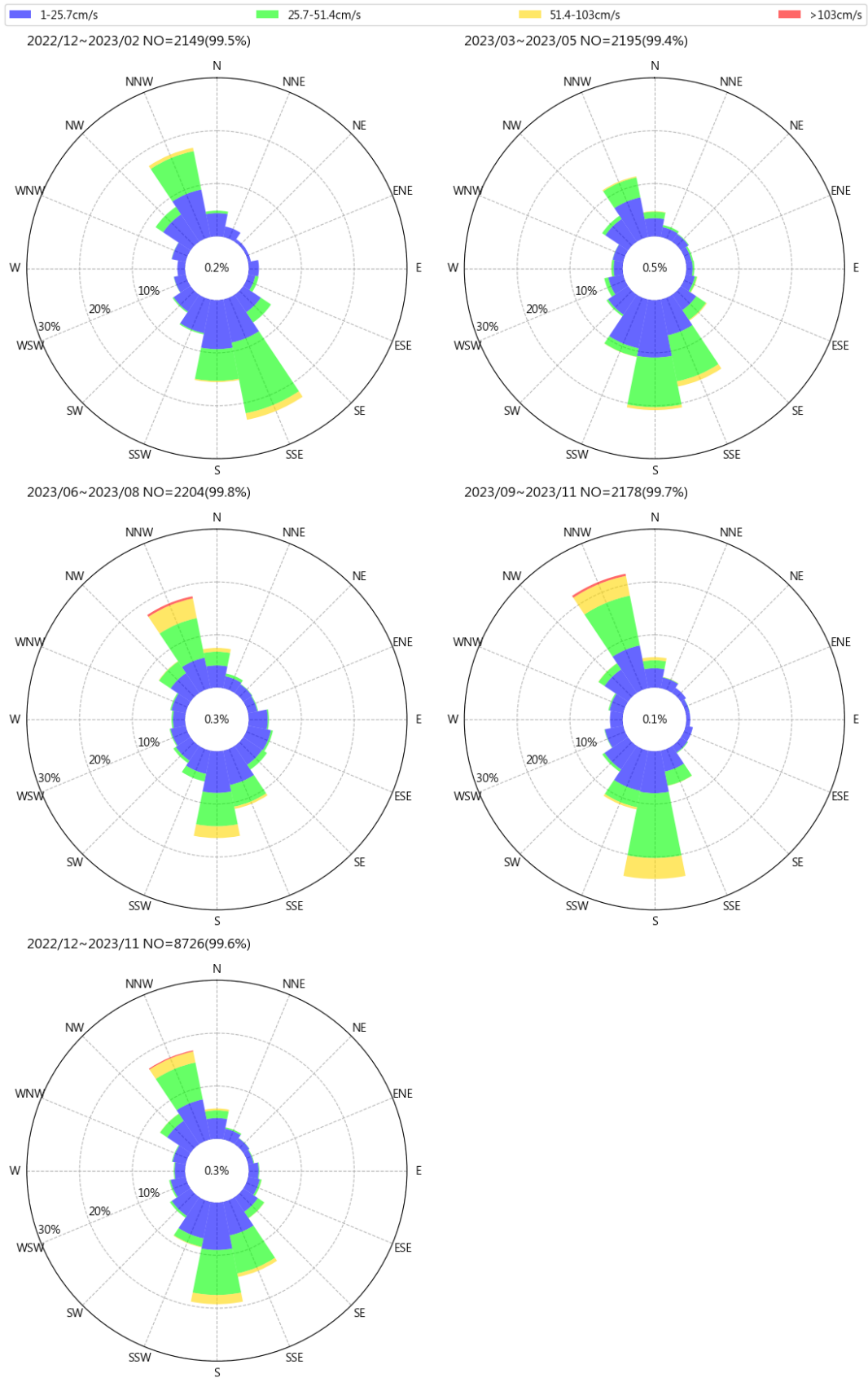
圖 6.6 2023 年高雄港每季流速流向玫瑰圖
