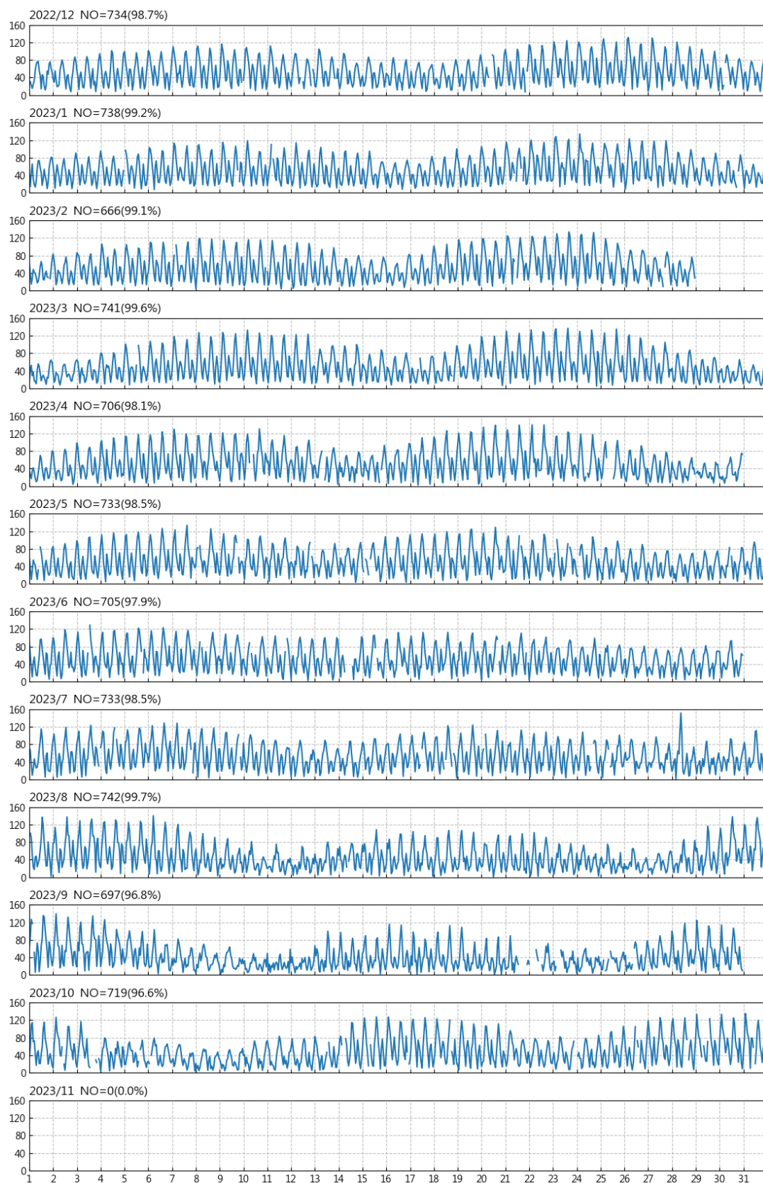
圖 11.3 2023 年金門水頭港每月流速歷線圖
