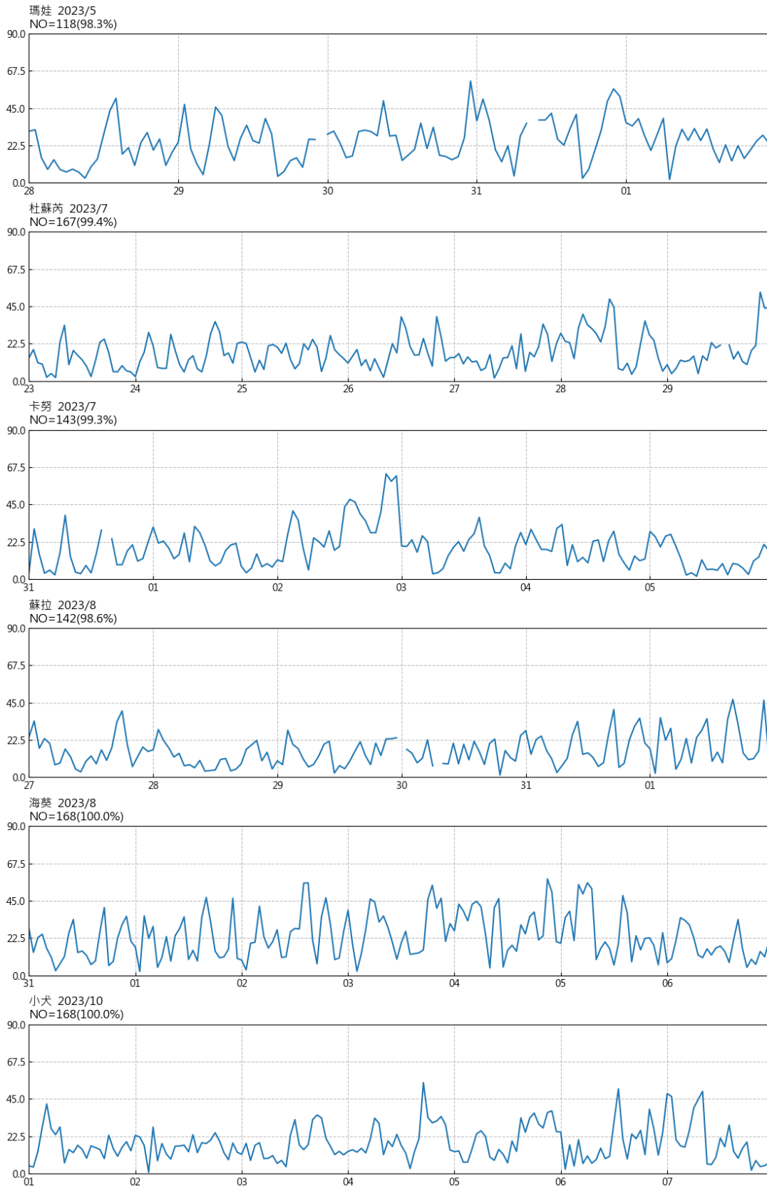
圖 4.9 2023 年蘇澳港颱風期間流速歷線圖
