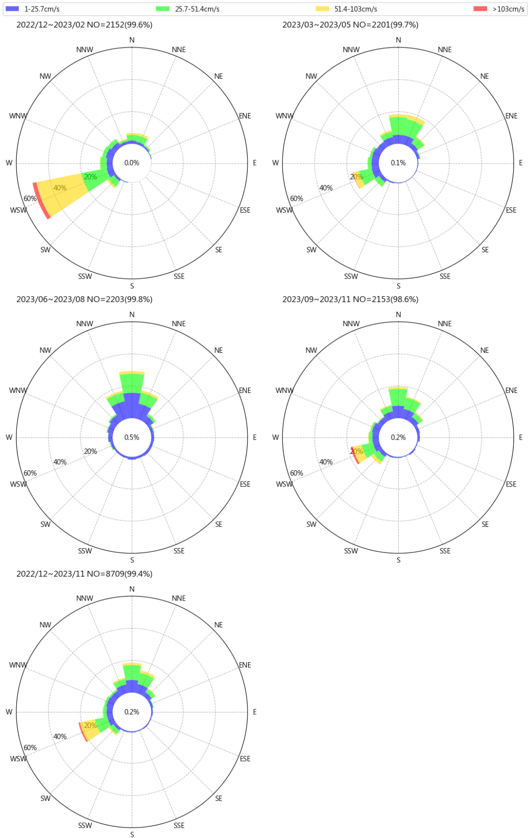
圖 9.6 2023 年臺中港每季流速流向玫瑰圖
