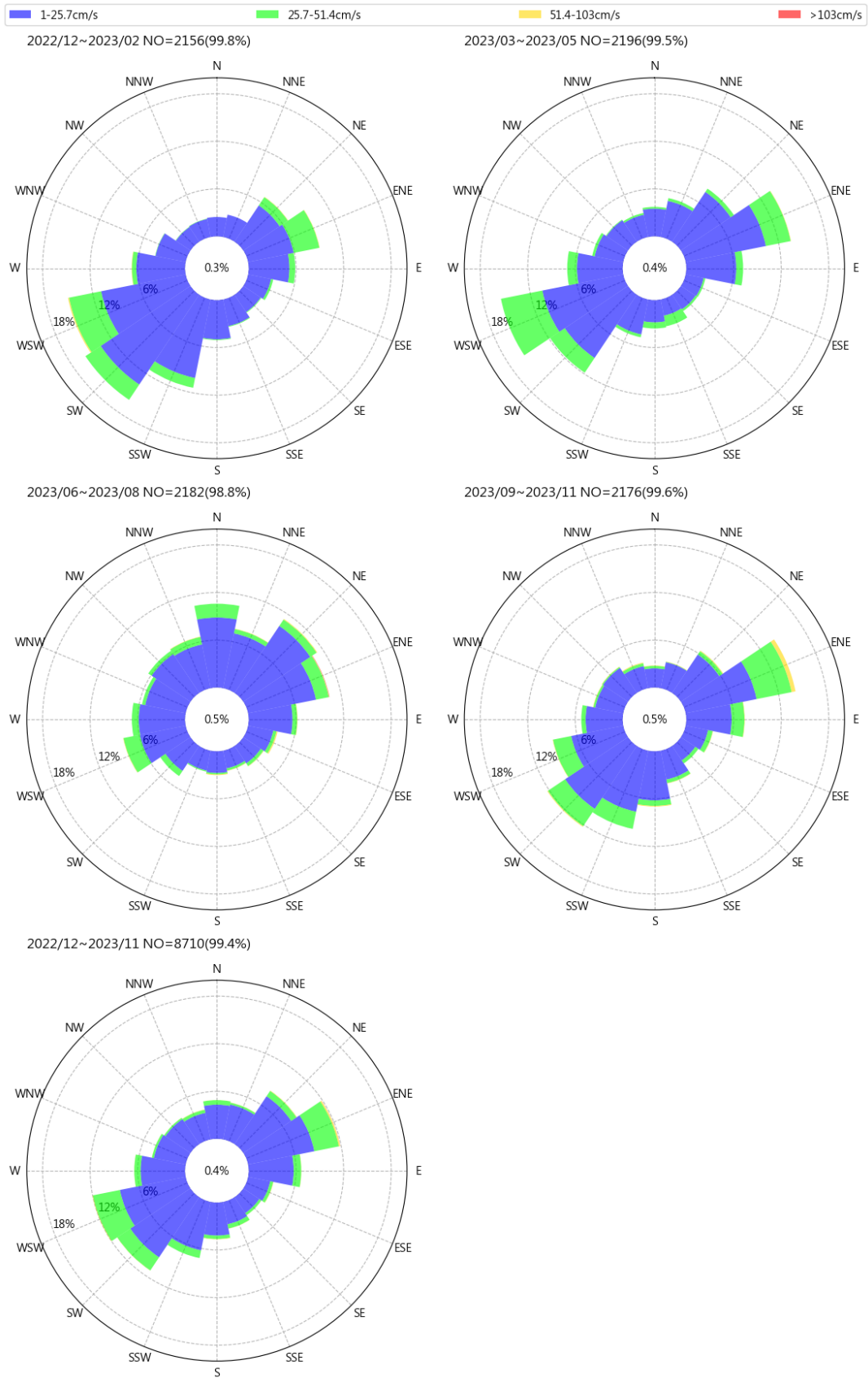
圖 5.6 2023 年花蓮港每季流速流向玫瑰圖
