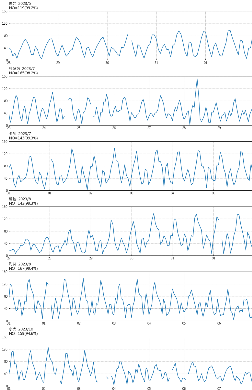
圖 11.9 2023 年金門水頭港颱風期間流速歷線圖
