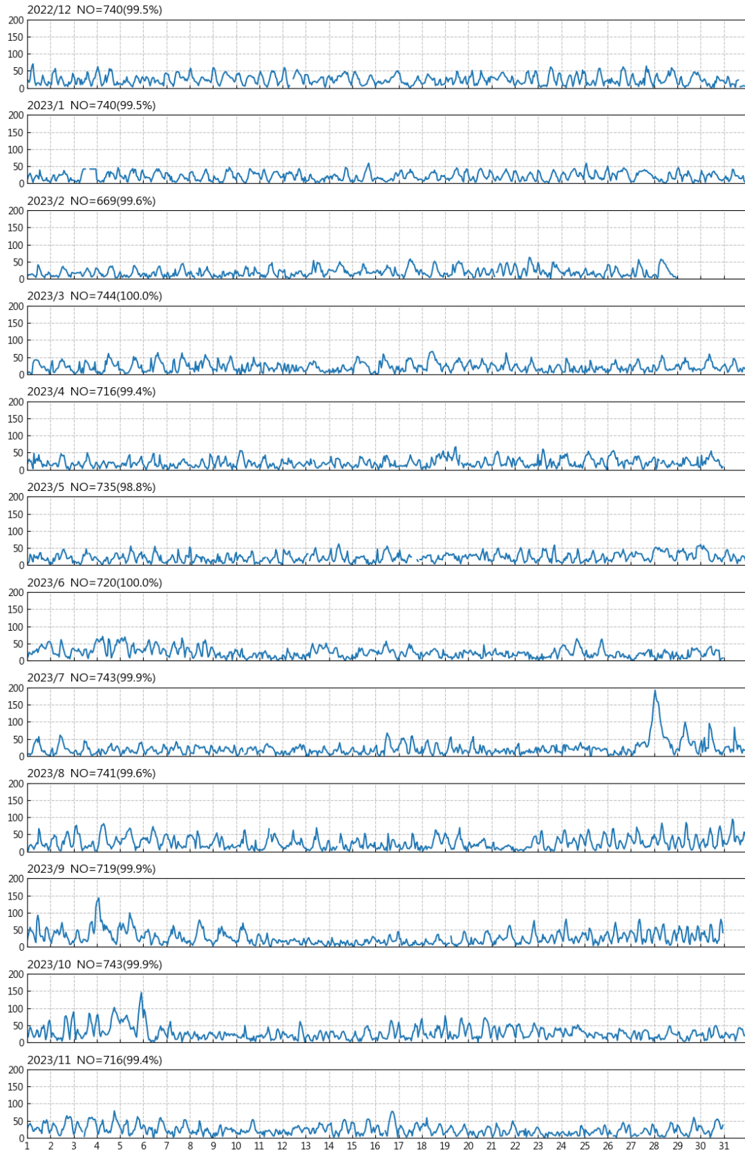
圖 6.3 2023 年高雄港每月流速歷線圖
