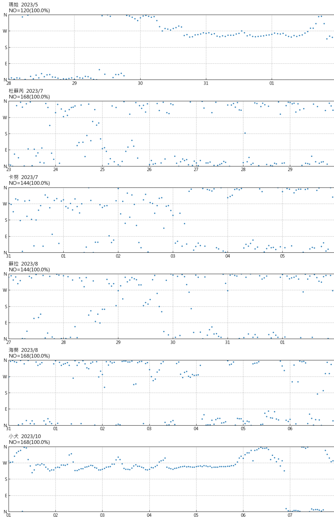
圖 9.10 2023 年臺中港颱風期間流向歷線圖
