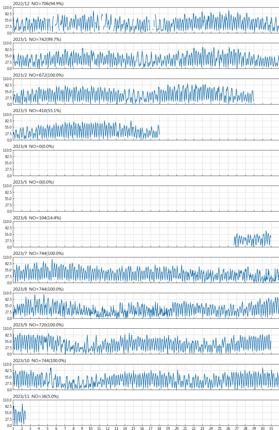
圖 2.3 2023 年臺北港每月流速歷線圖
