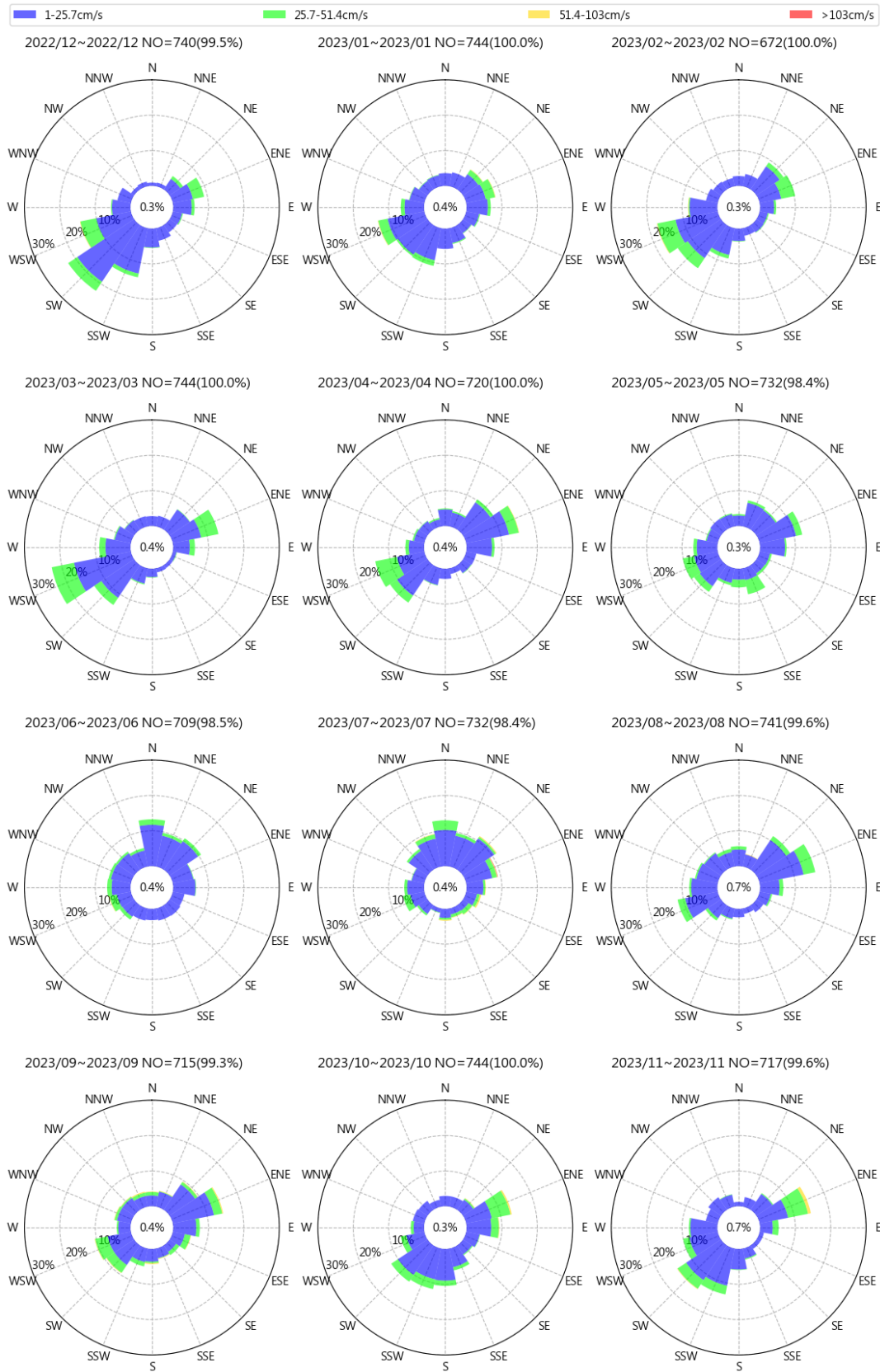
圖 5.5 2023 年花蓮港每月流速流向玫瑰圖
