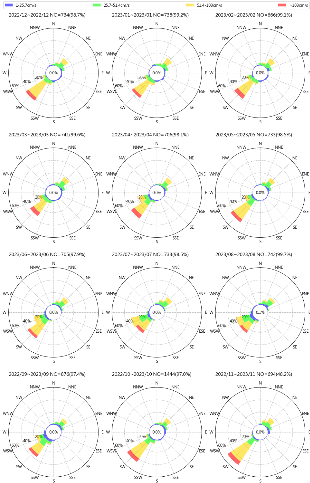
圖 11.7 歷年金門水頭港每月流速流向玫瑰圖
