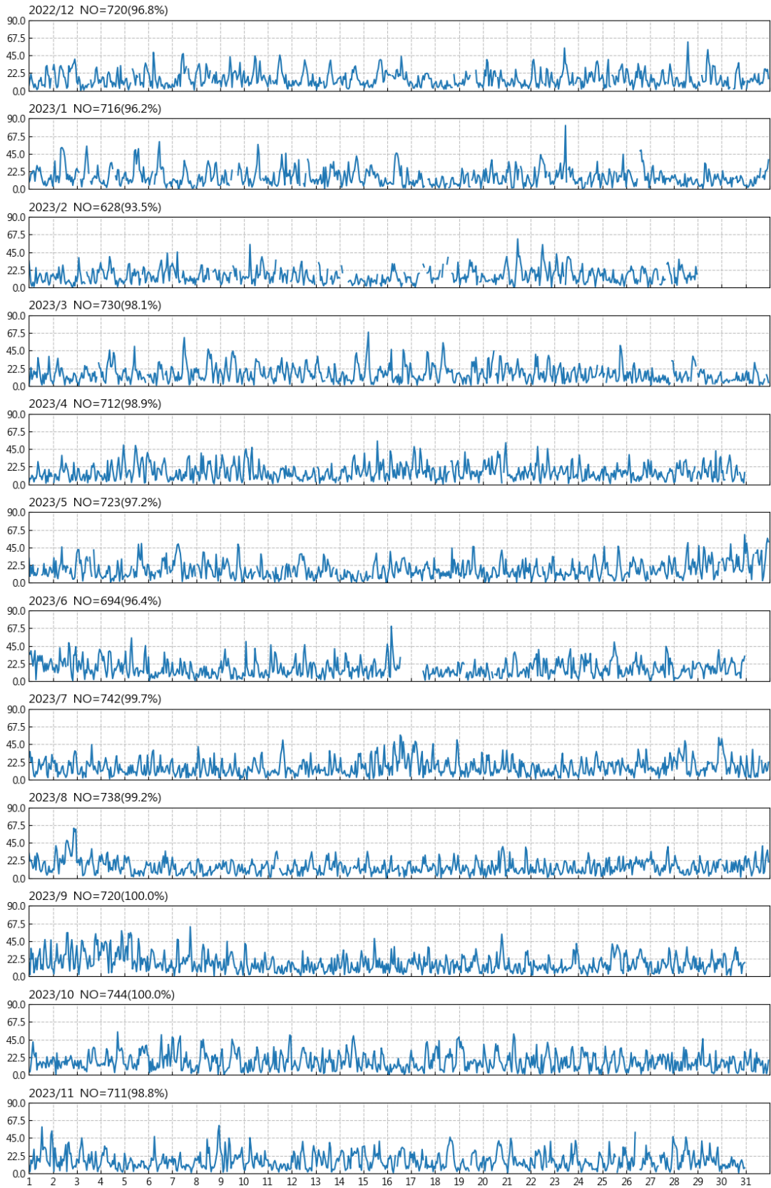
圖 4.3 2023 年蘇澳港每月流速歷線圖
