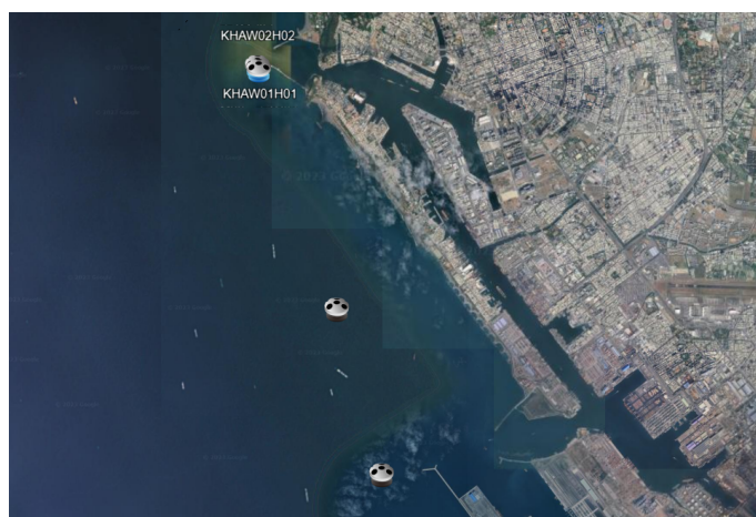
圖 6.1 高雄港海流觀測站位置示意圖
