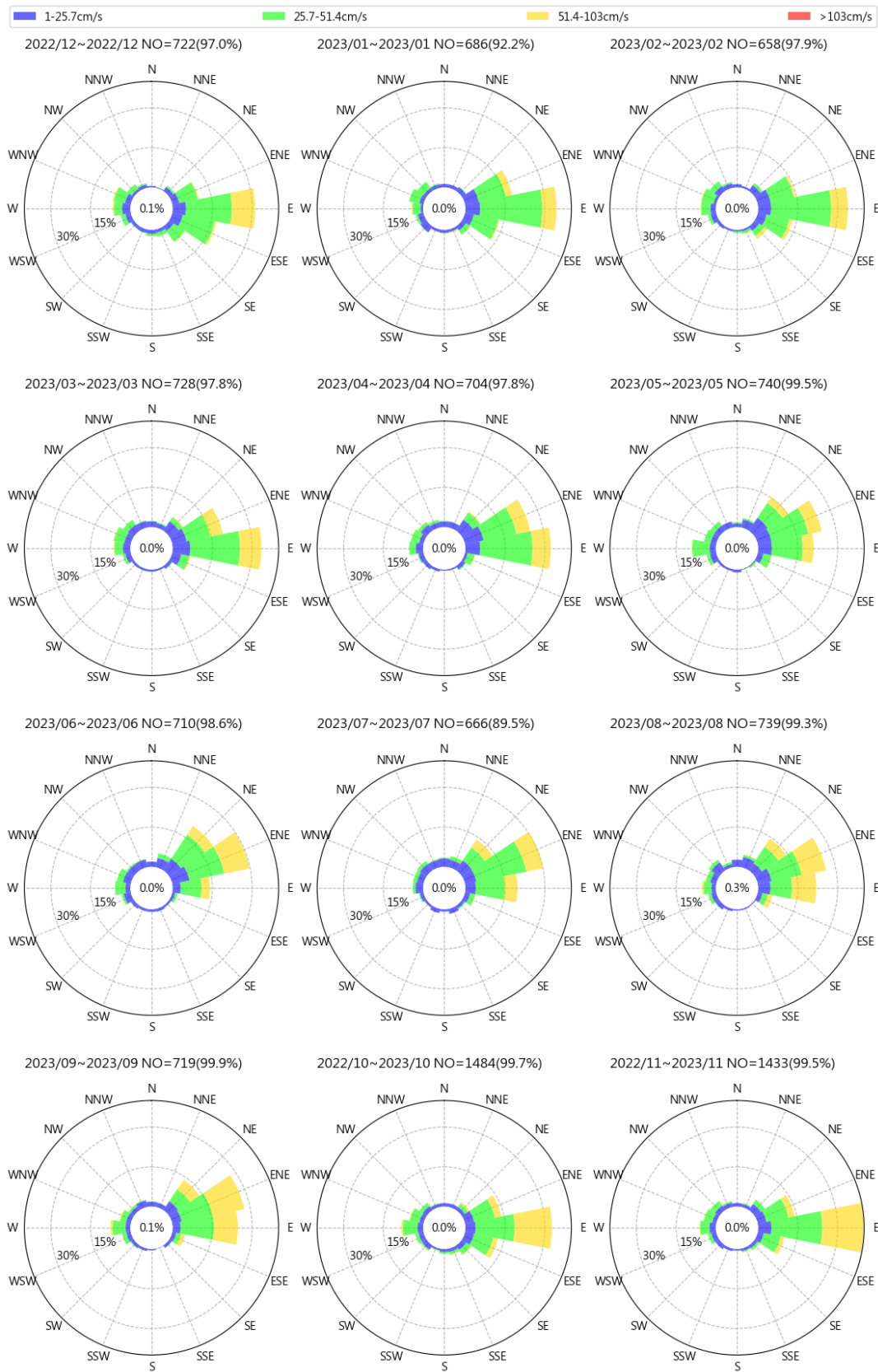
圖 10.7 歷年澎湖龍門尖山港每月流速流向玫瑰圖
