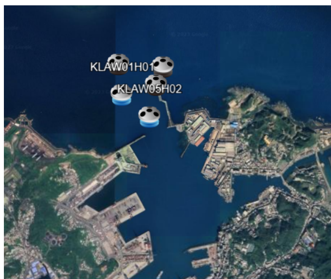
圖 3.1 基隆港海流觀測站位置示意圖
