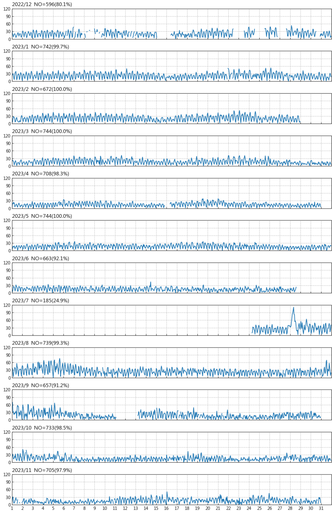
圖 8.3 2023 年布袋港每月流速歷線圖
