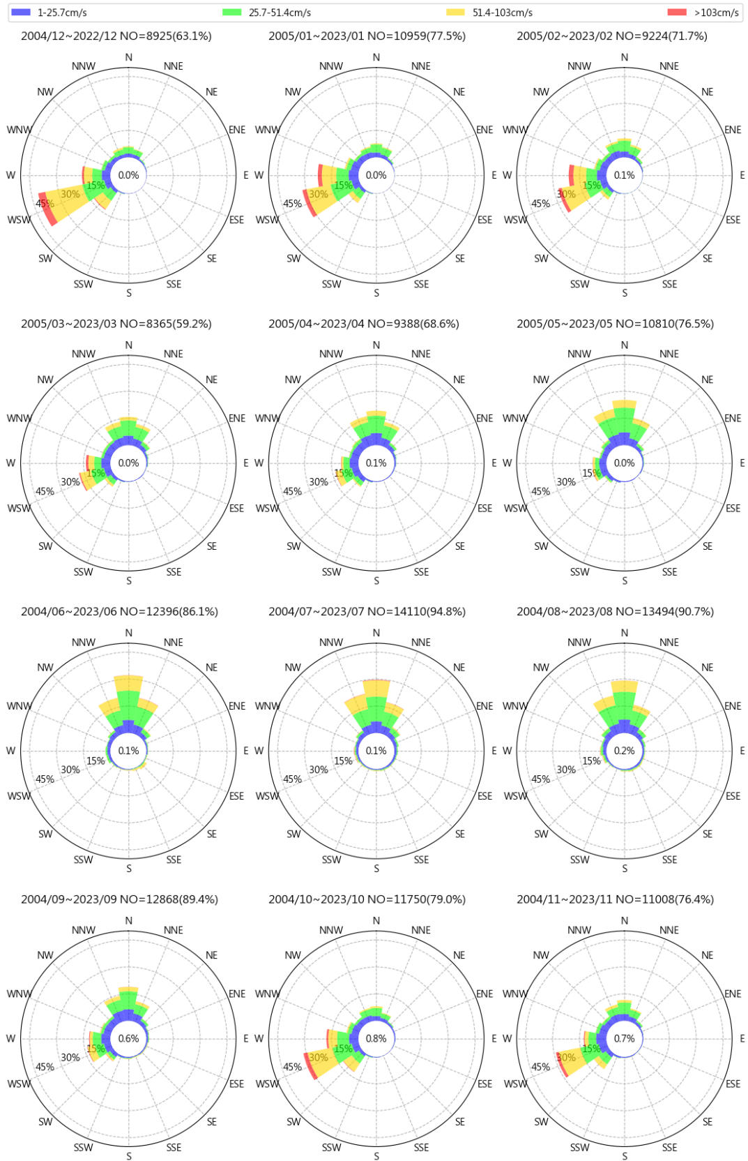
圖 9.7 歷年臺中港每月流速流向玫瑰圖
