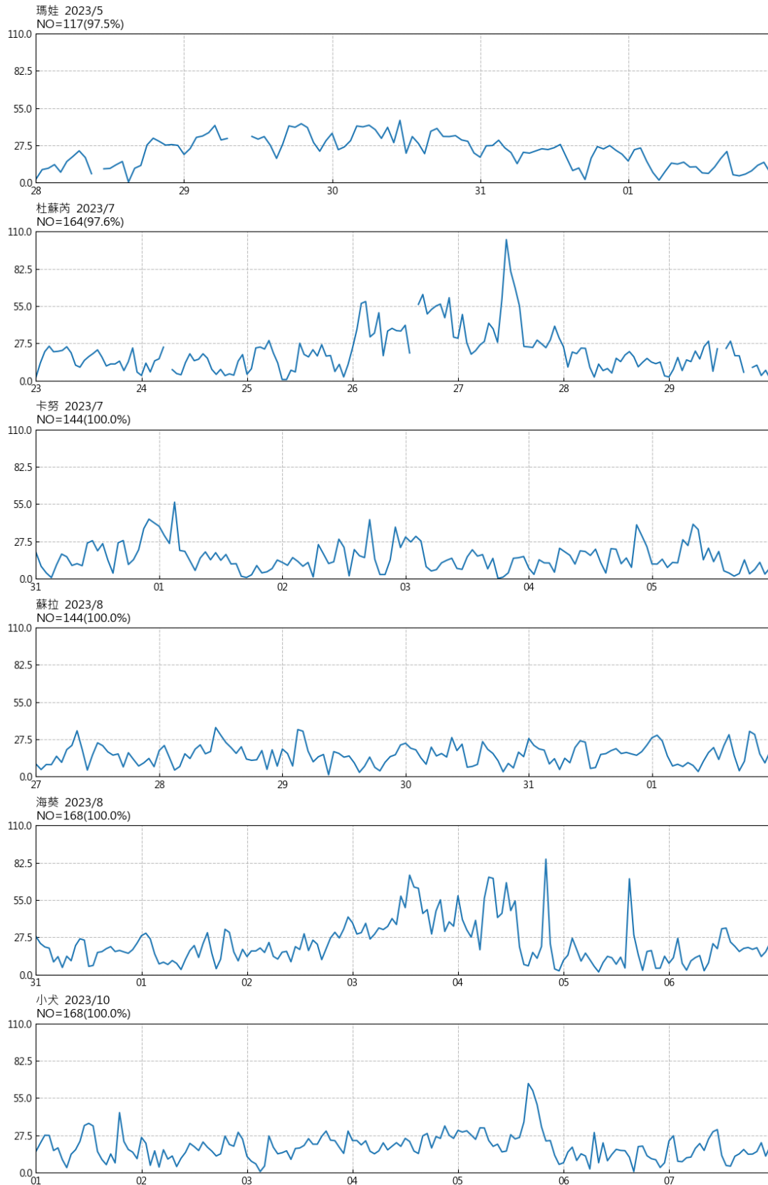
圖 5.9 2023 年花蓮港颱風期間流速歷線圖
