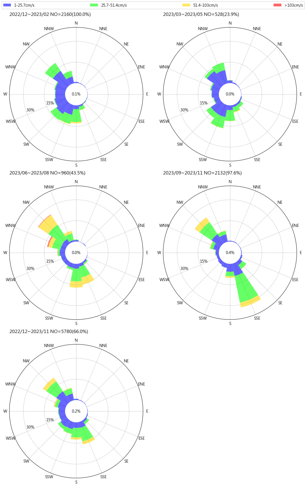
圖 7.6 2023 年安平港每季流速流向玫瑰圖
