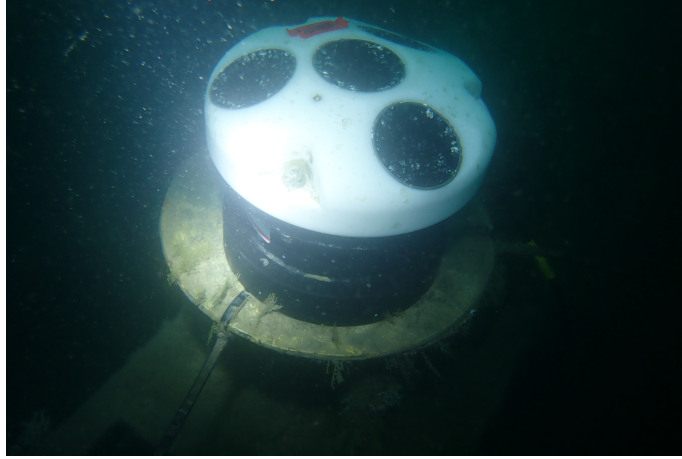
圖 2.2 臺北港海流觀測站現地照片
