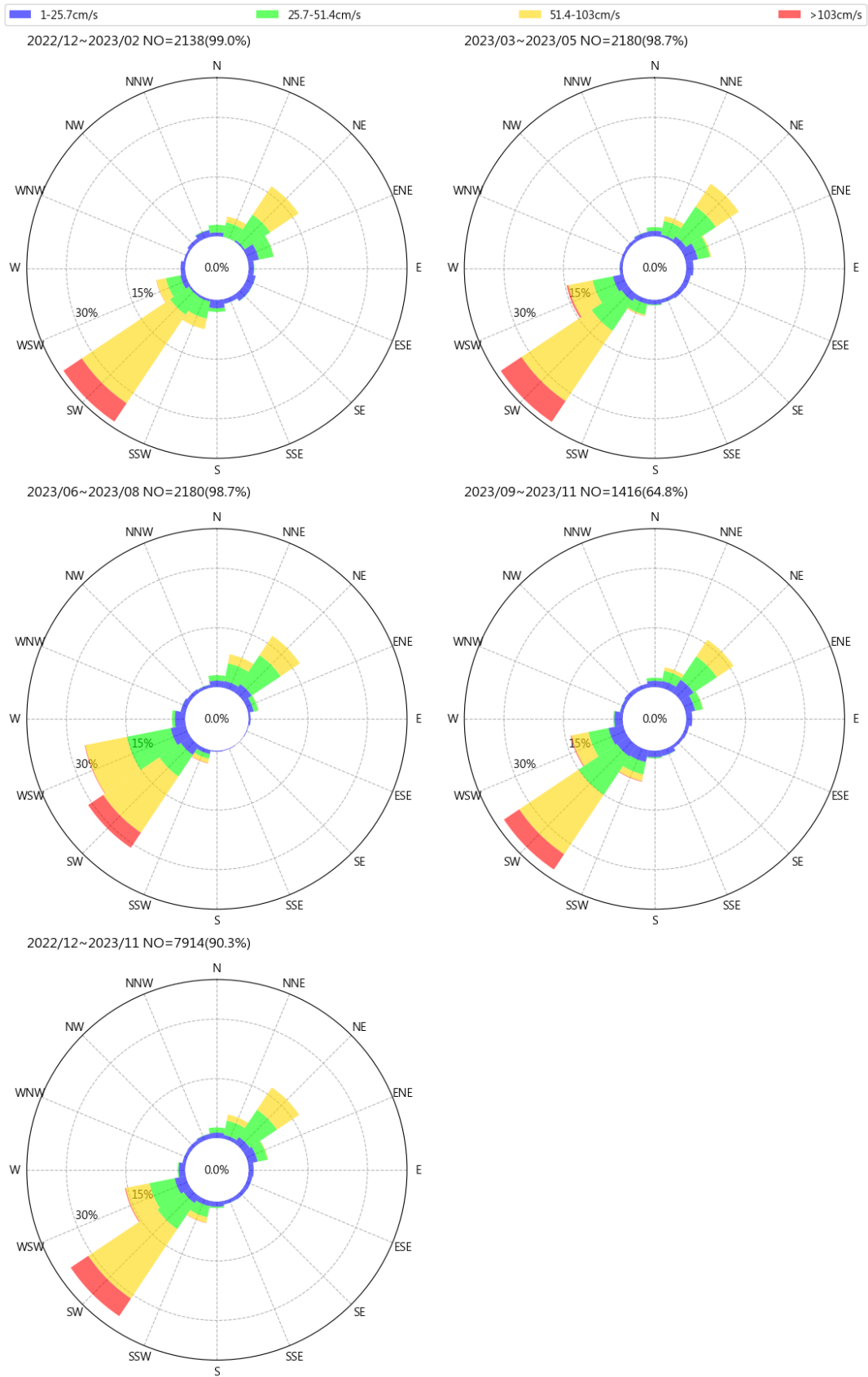
圖 11.6 2023 年金門水頭港每季流速流向玫瑰圖
