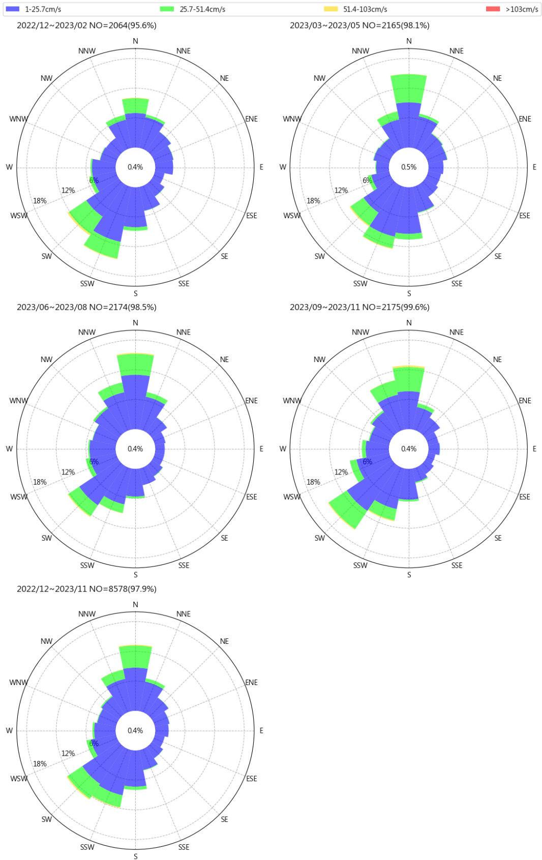
圖 4.6 2023 年蘇澳港每季流速流向玫瑰圖
