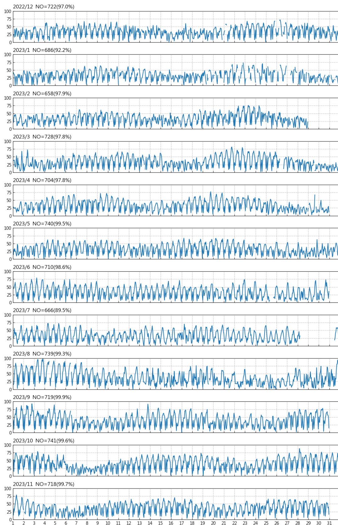
圖 10.3 2023 年澎湖龍門尖山港每月流速歷線圖
