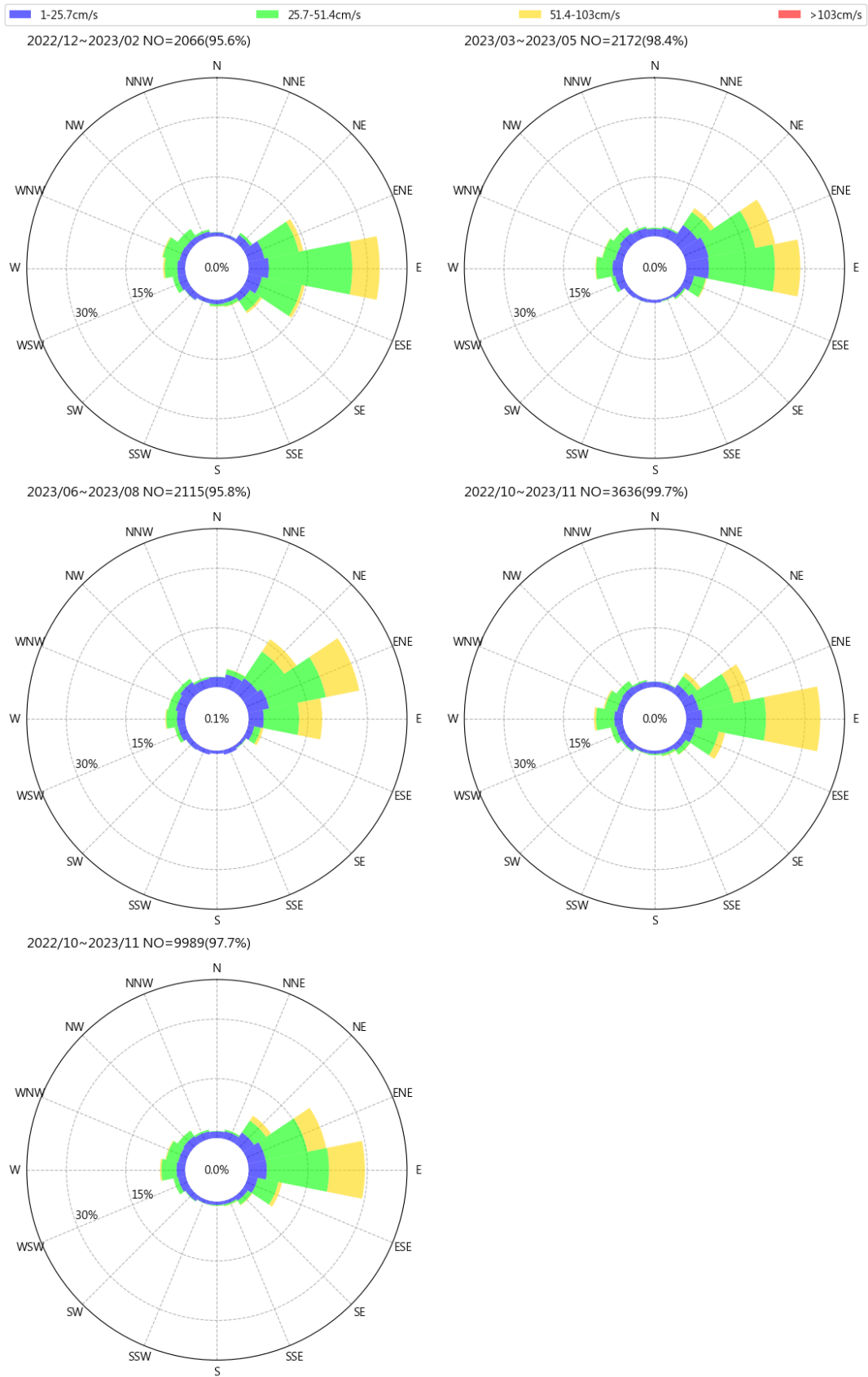
圖 10.8 歷年澎湖龍門尖山港每季流速流向玫瑰圖
