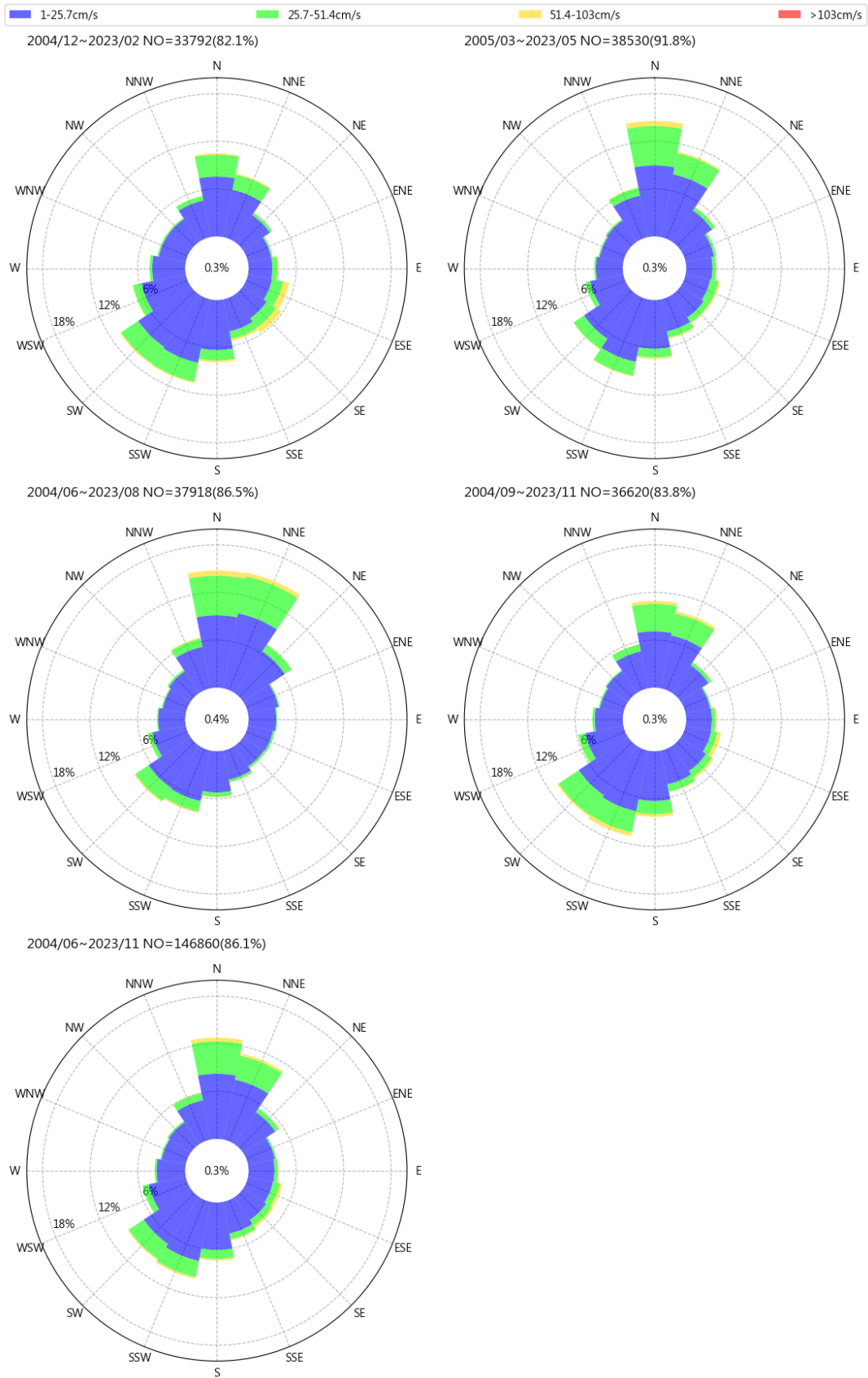
圖 4.8 歷年蘇澳港每季流速流向玫瑰圖
